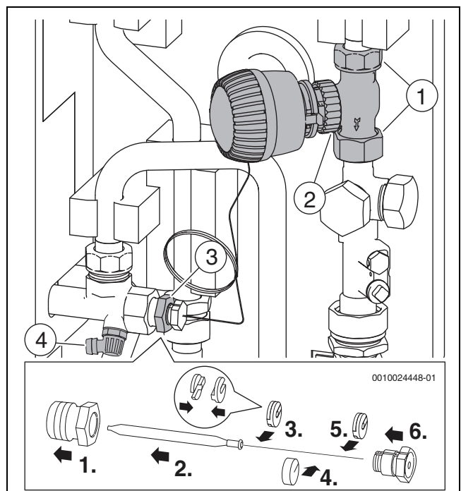
Bild 40 Warmwasserthermostat und Temperaturfühler
