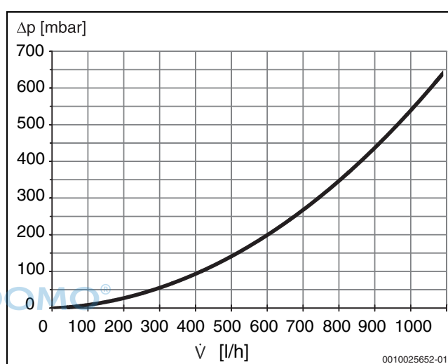
Bild 7 Druckverlust Primärseite
