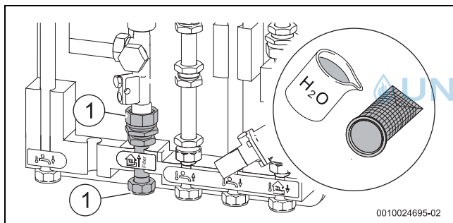
Bild 38 Filter reinigen
