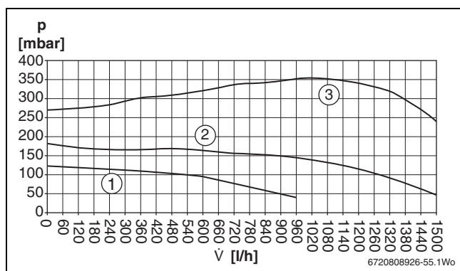
Bild 33 Restförderhöhe
