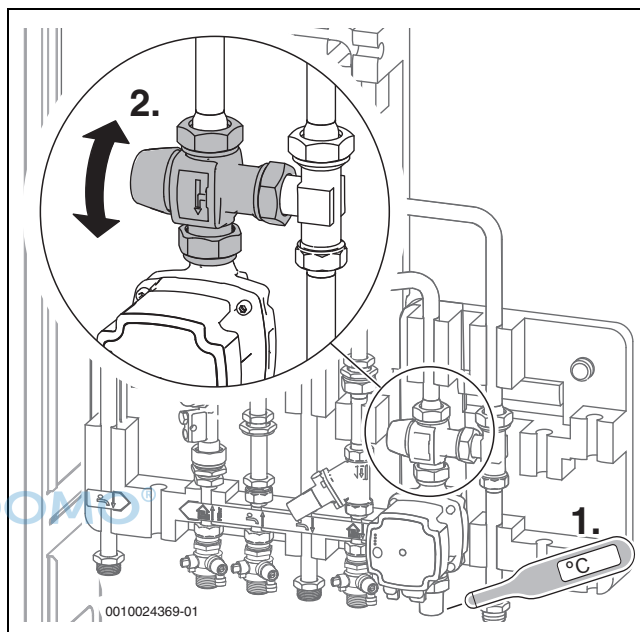
Bild 31 Maximale Vorlauftemperatur einstellen
