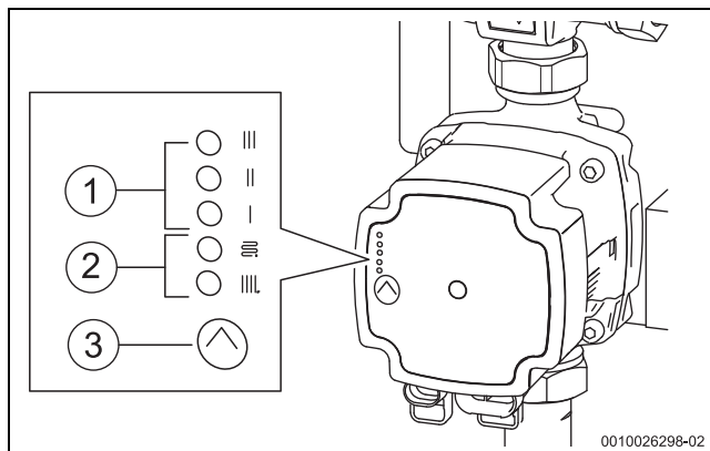
Bild 32 Statusanzeigen der integrierten Heizungspumpe
