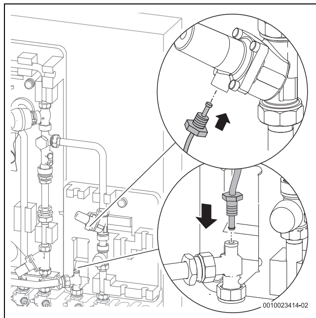
Bild 24 Kapillarleitung montieren
