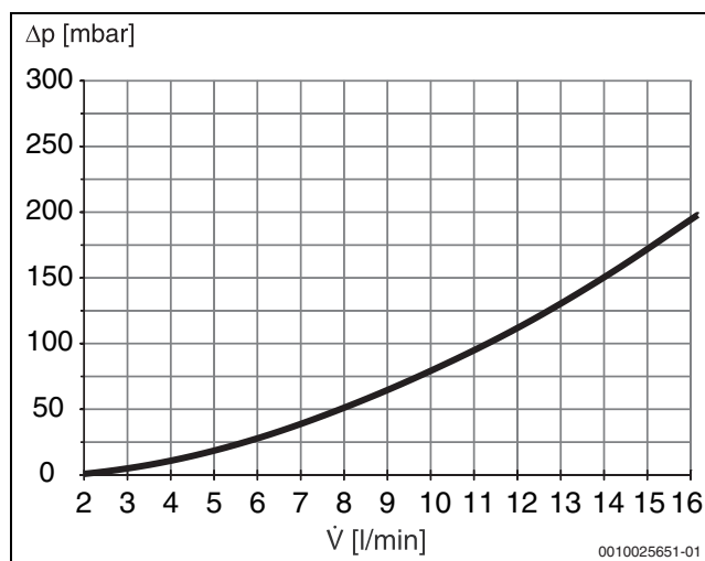
Bild 6 Druckverlust Trinkwasserseite
