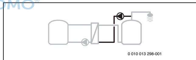
Bild 43 Tägliche Aufheizung
