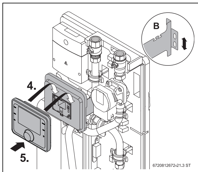
Bild 38 Bedieneinheit montieren
