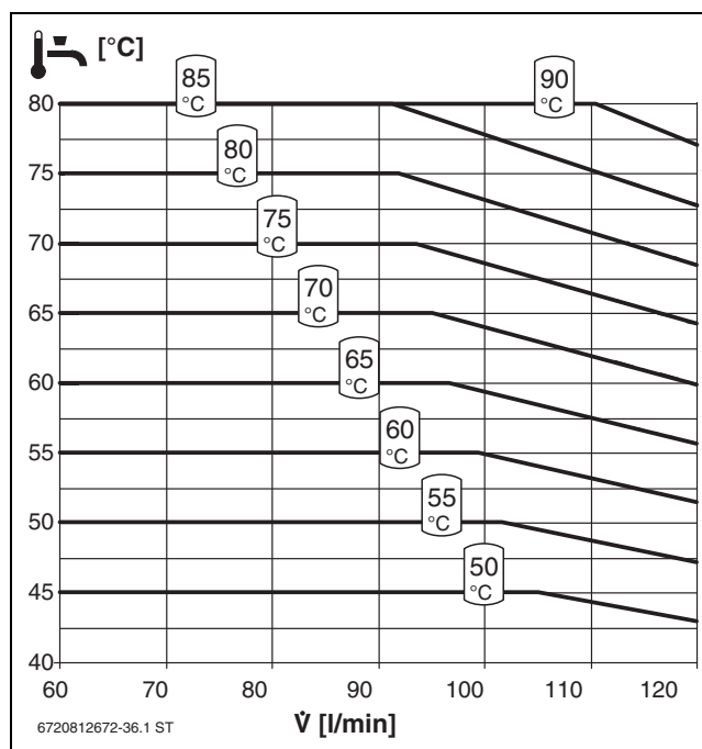
Bild 62 Temperaturverhalten Kaskade FF120S
