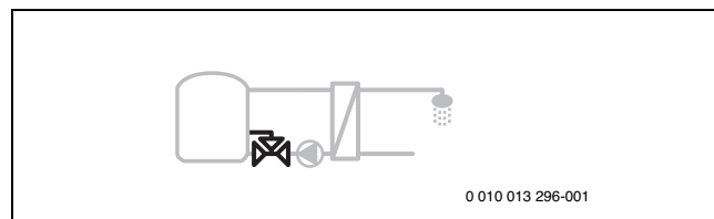
Bild 41 Ventil Rücklauf
