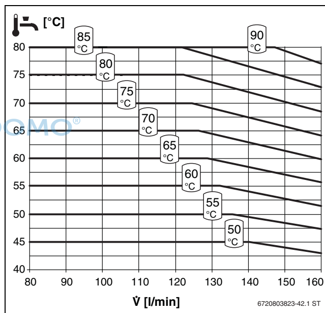
Bild 63 Temperaturverhalten Kaskade FF160S
