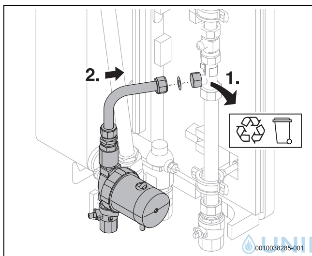
Bild 21 Zirkulationsstrang montieren
