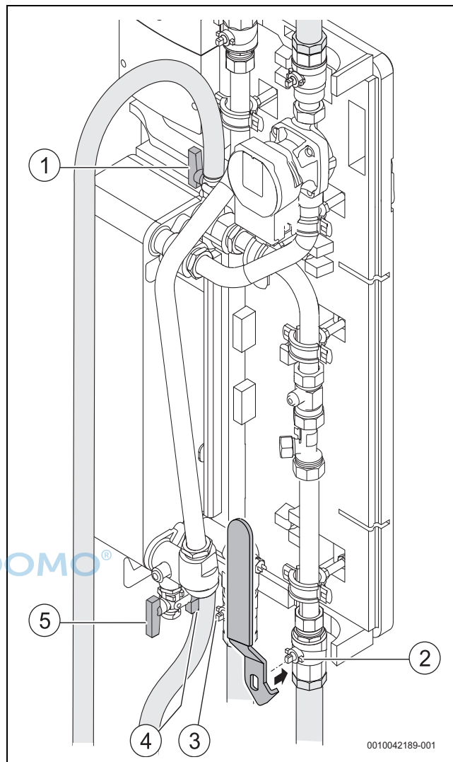
Bild 65 Wartung Frischwasserstation
