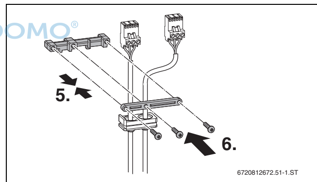
Bild 51 Zugentlastung montieren
