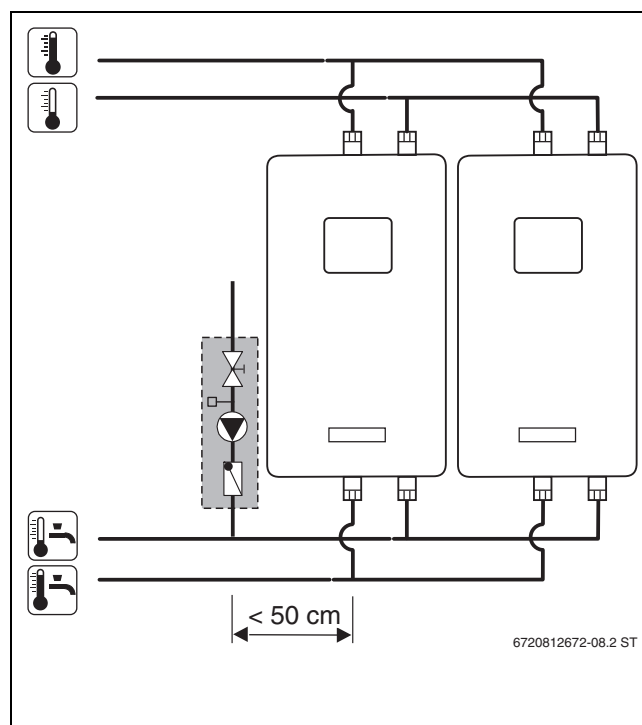
Bild 23 Zirkulationspumpe außerhalb der Kaskade
