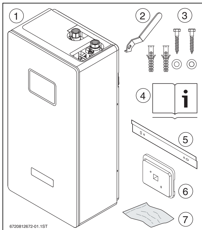
Bild 2 Lieferumfang Einzelstation
