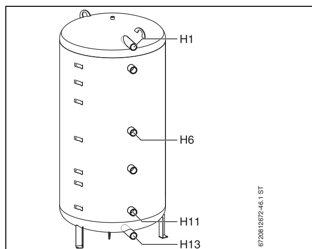
Bild 36 Pufferspeicher als Solarspeicher für Vorwärmesystem (auch mit internem Wärmetauscher möglich), Hydraulik (→ Bild 7, Seite 8)
