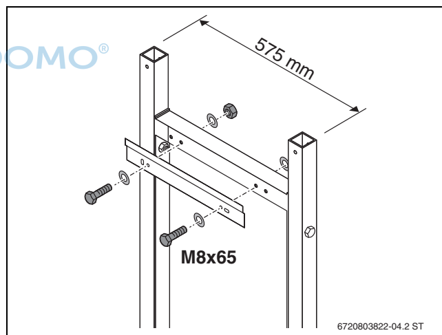
Bild 20 Wandhalter montieren
