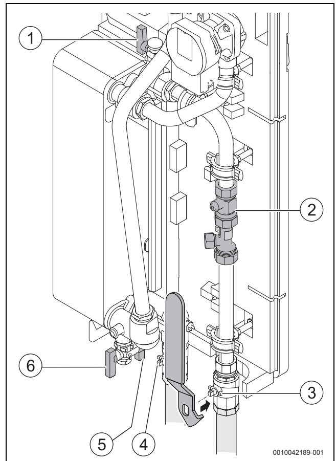
Bild 66 Volumenstromfühler wechseln
