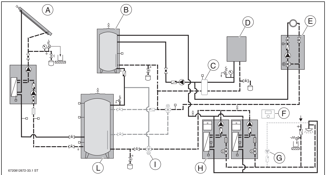
[A] Solaranlage [B] Pufferspeicher als Bereitschaftsspeicher [C] Hydraulische Weiche (optional) [D] Nachheizung [E] Heizkreis [F] Bedieneinheit (Zubehör, muss vorhanden sein) [G] Zirkulationspumpe (bauseits) [H] Frischwasserstation Kaskade mit Kaskadenventilen [I] Rücklaufventil VS5 (Zubehör für temperatursensible Einspeisung) [L] Pufferspeicher
