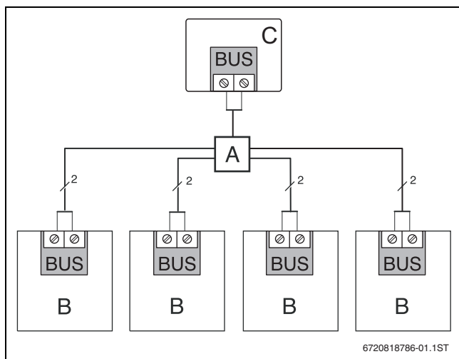
Bild 53 BUS-Leitungen anschließen
