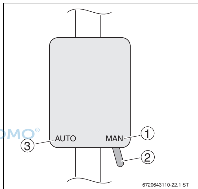
Bild 54 Zum Befüllen und Spülen das 2-Wege-Motorventil auf „MAN“ stellen
