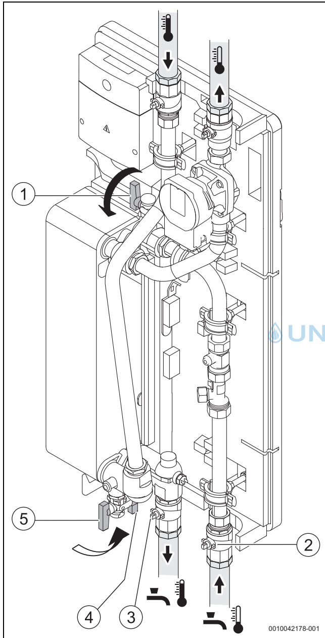
Bild 55 Spül-/Befüllvorrichtungen an der Einzelstation
