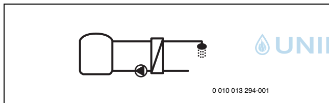
Bild 39 Frischwassersystem
