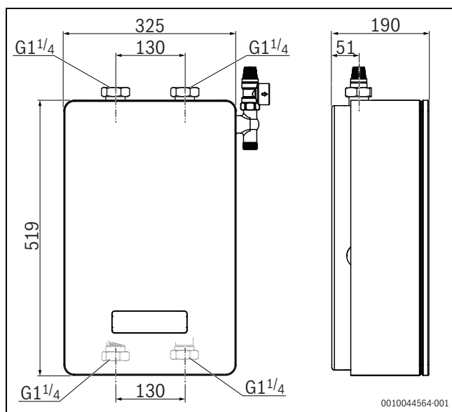
Bild 31 Abmessungen
