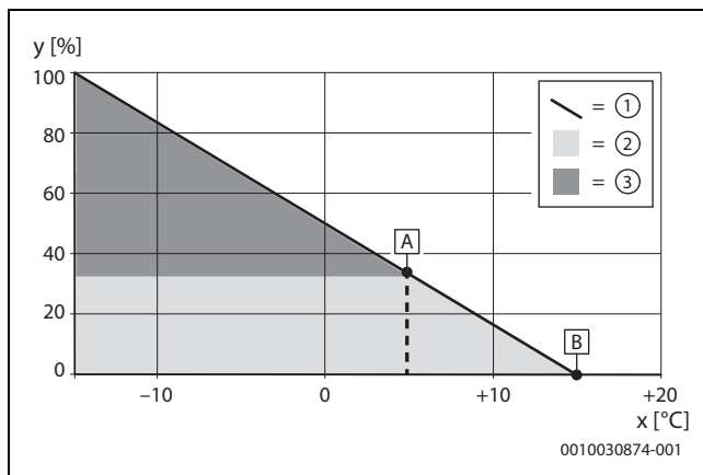
Bild 1 Außentemperatur parallel
