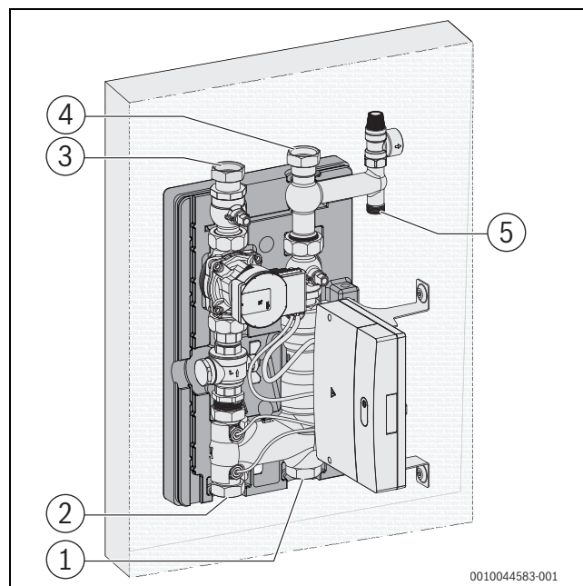
Bild 12 Anschlüsse am Hybrid-Set
