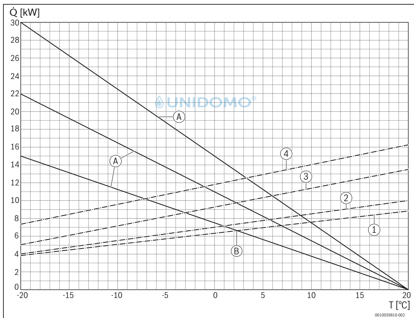
Bild 28 Diagramm zu Tab. 13; Zur Bestimmung der Bivalenzpunkte bei 45 °C Vorlauftemperatur
