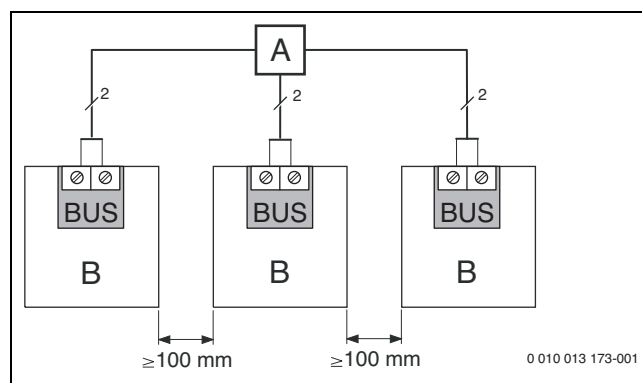
Bild 15 Verteilerdose anschließen
