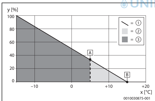
Bild 2 Außentemperatur alternativ
