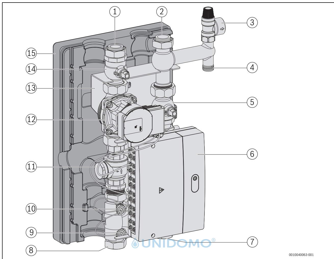
Bild 5 Produktübersicht (Dargestellt: Anschluss-Set HW)
