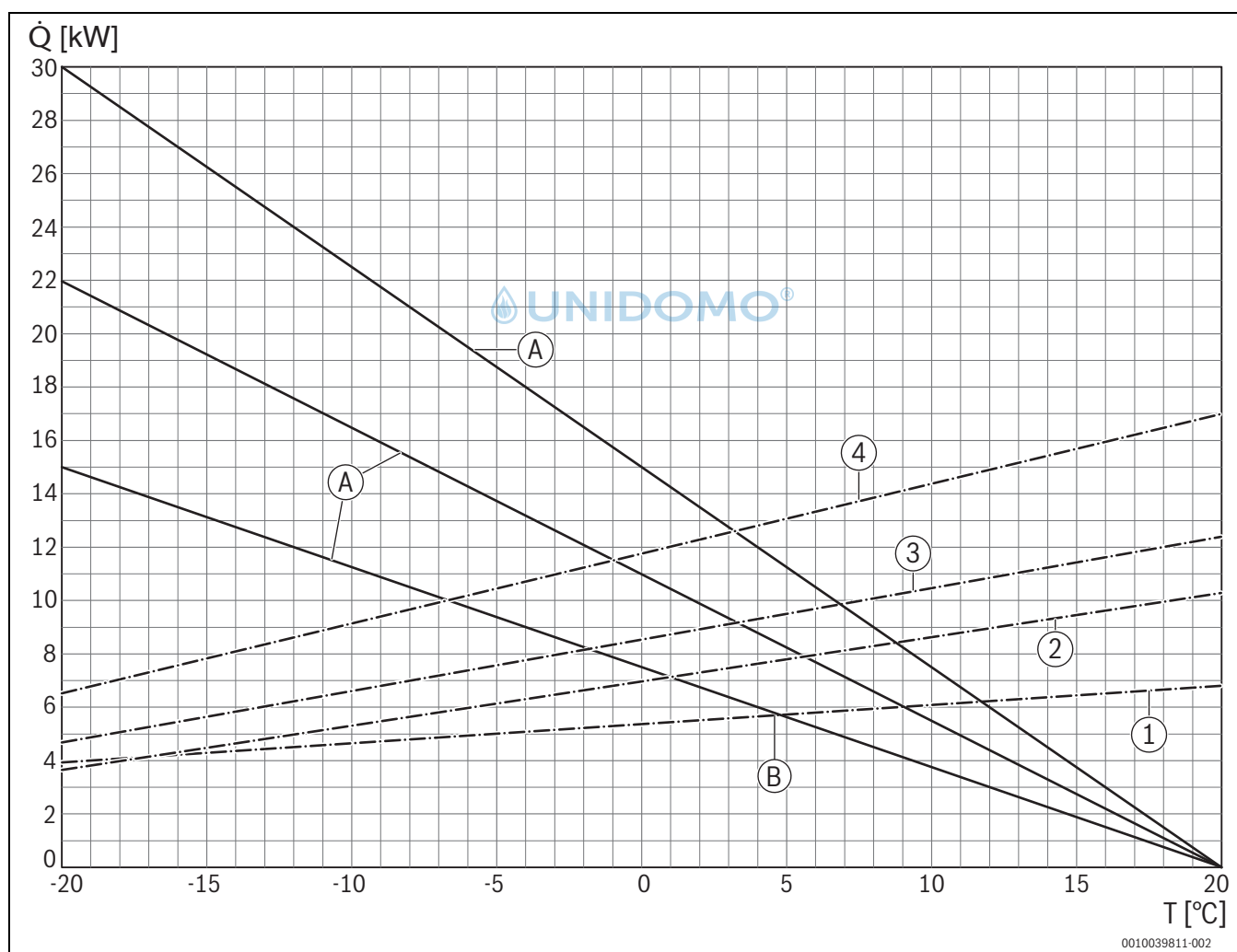
Bild 29 Diagramm zu Tab. 14; Zur Bestimmung der Bivalenzpunkte bei 55 °C Vorlauftemperatur
