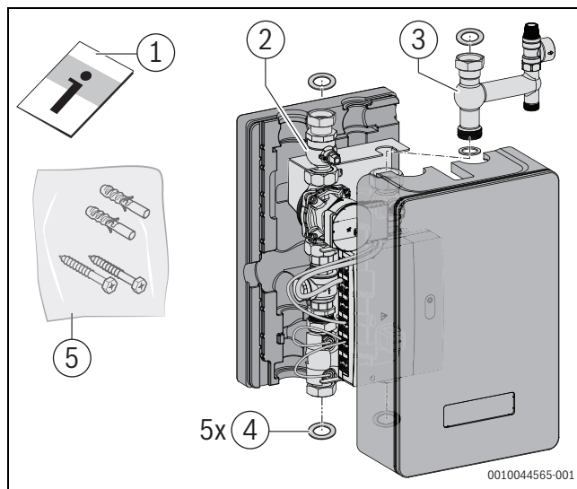
Bild 4 Lieferumfang HW-Set HYC25
