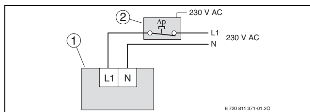
Bild 54 Anschluss Differenzdruckwächter in elektrischer Leitung
