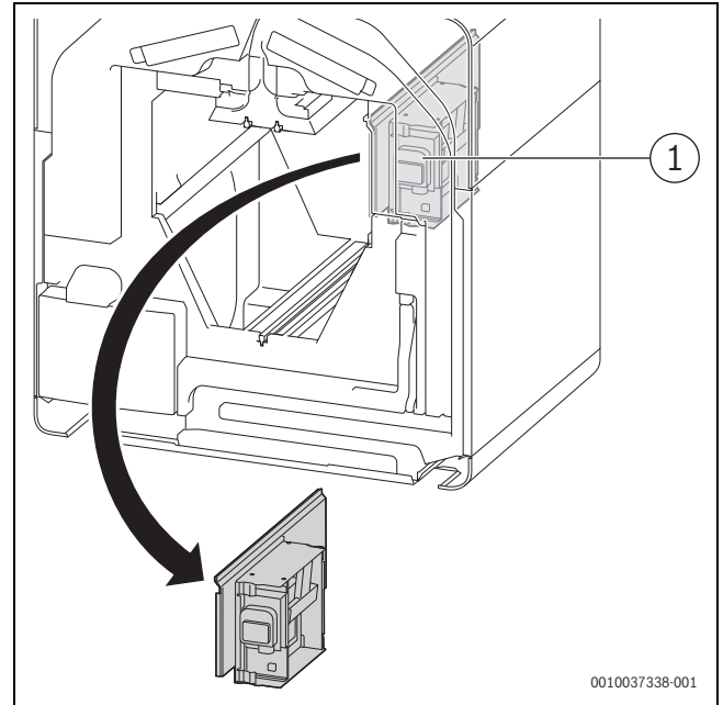
Bild 60 Bypass herausnehmen
