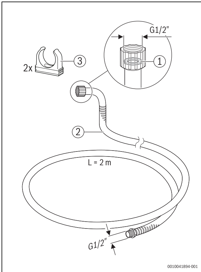
Bild 37 Schlauchsiphon-Anschluss-Set
