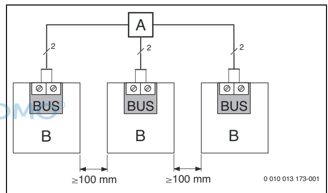
Bild 52 BUS-Verbindungen Leiterquerschnitte
