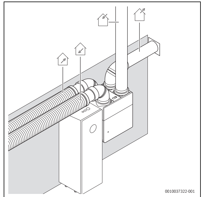
Bild 47 Variante 3: Geräteanschlüsse senkrecht - Luftführung Variante A
