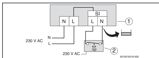
Bild 53 Anschluss Differenzdruckwächter an der Elektronik
