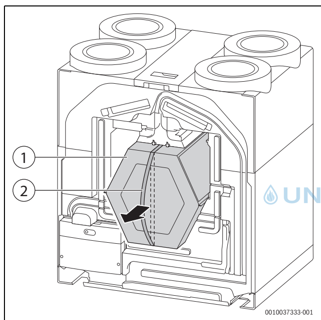
Bild 58 Wärmetauscher herausziehen
