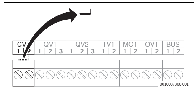
Bild 29 Brücke entfernen
