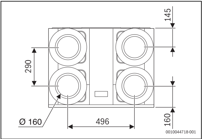
Bild 5 Abmessungen Anschlussstutzen
