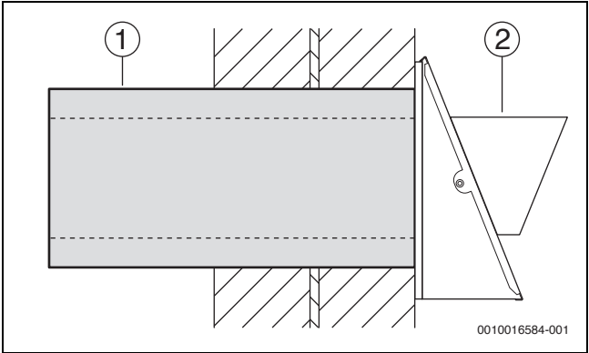
Bild 41 Rohrdämmung
