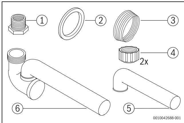
Bild 39 Kugelsiphon-Anschluss-Set
