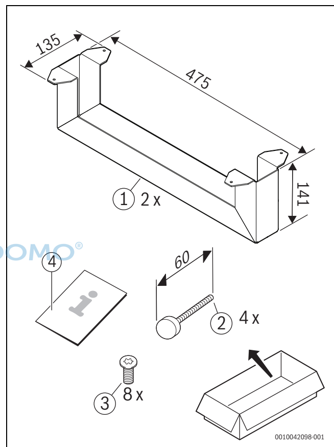
Bild 35 Lieferumfang HRV-FMS
