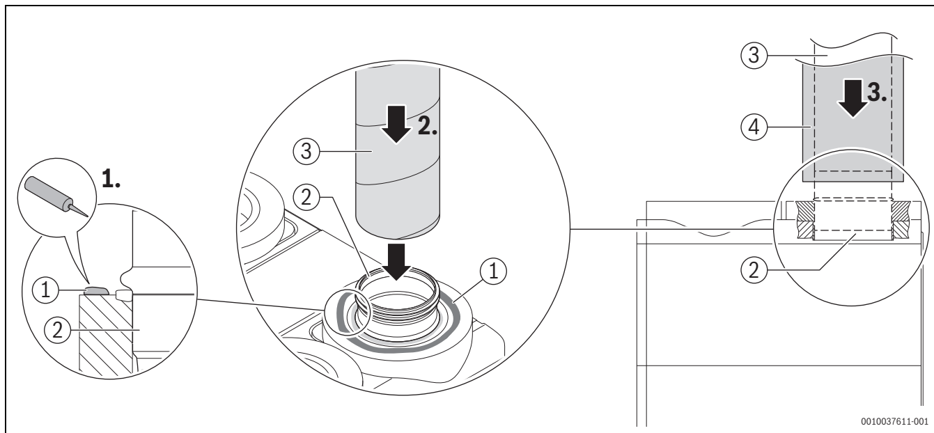
Bild 44 Aufbau Luftrohranschluss
