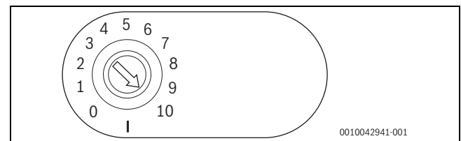
Bild 57 Kodierschalter auf Position 10 = autarker Betrieb
