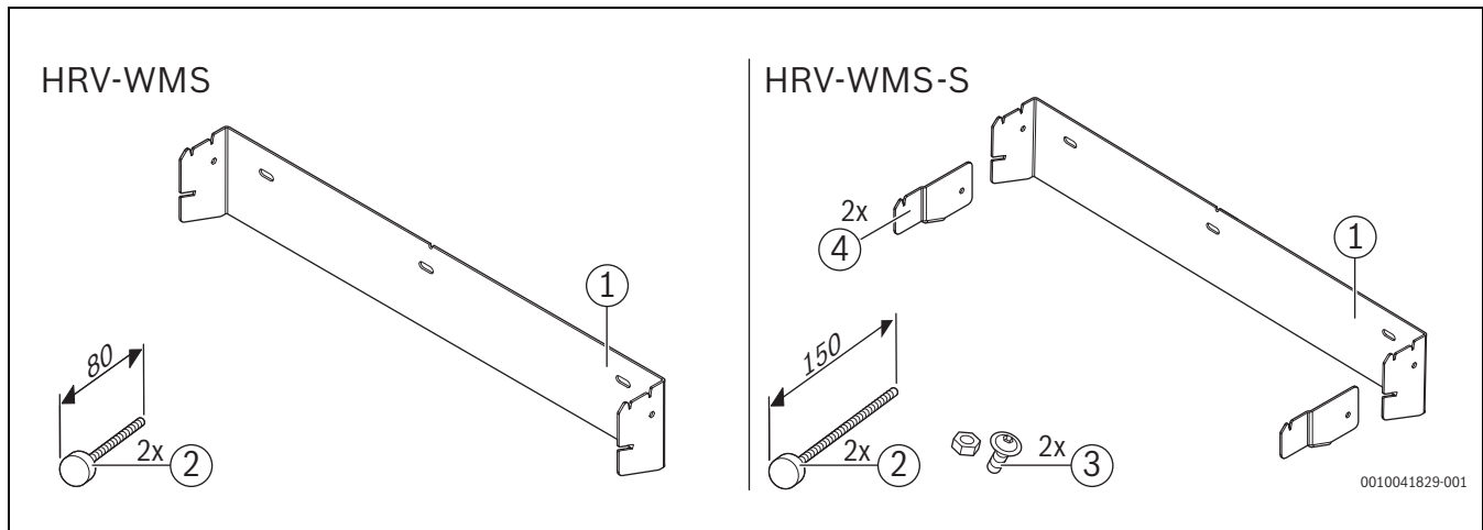
Bild 31 Lieferumfang HRV-WMS/HRV-WMS-S
