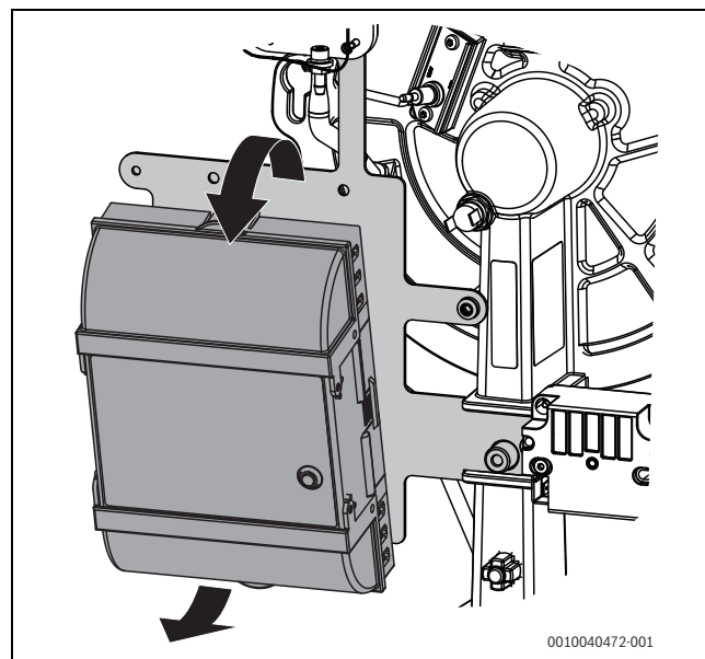
Fig. 52 Sgancio dell'automatismo di combustione
