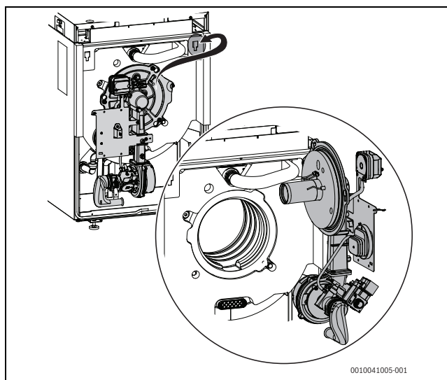
Fig. 58 Bruciatore in posizione di manutenzione
