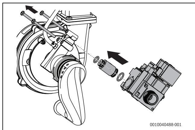
Fig. 30 Udskift gasdysen
