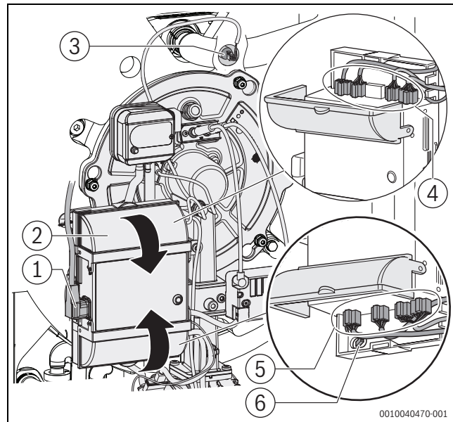
Fig. 51 Distacco giunti ad innesto
