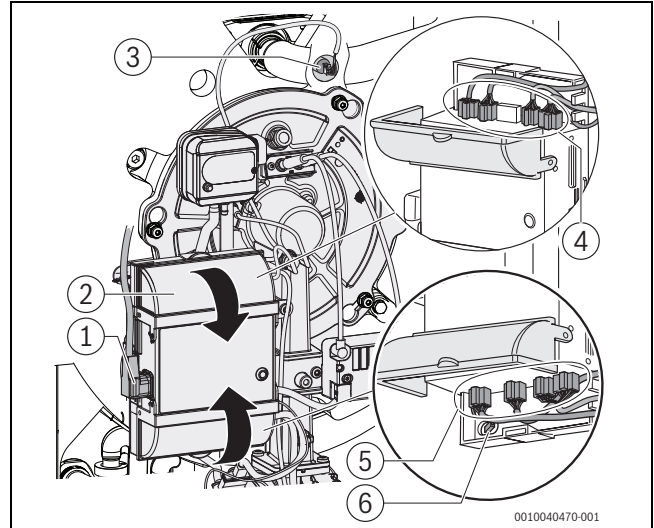
Afb. 67 Steekverbindingen losmaken
