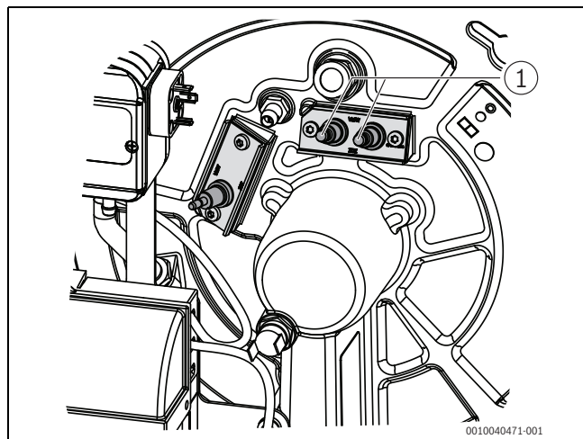
Fig. 53 Elettrodo accensione
