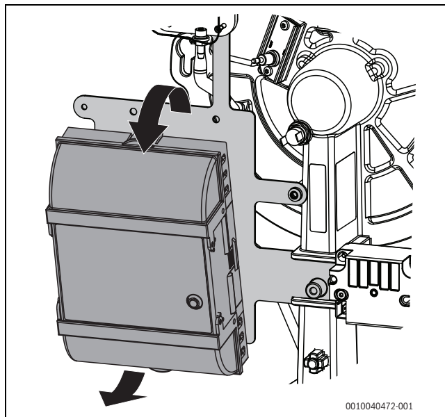
Bild 4 Feuerungsautomat lösen
