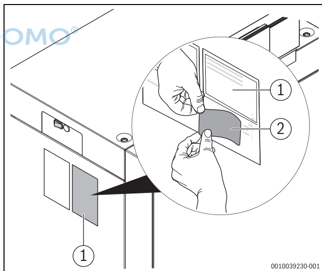
Fig. 32 Opmatér typeskiltet (eksempel med kedelvisning)
