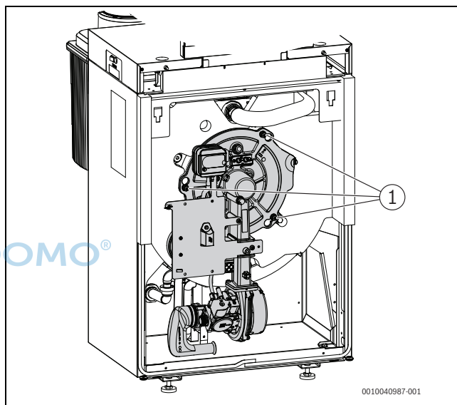
Fig. 25 Løsn fastspændingsmøtrikkerne
