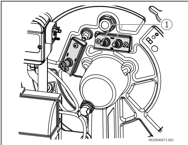
Afb. 69 Ontstekingselektrode
