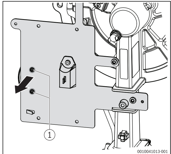
Afb. 76 Laaglastdrukcontrole demonteren
