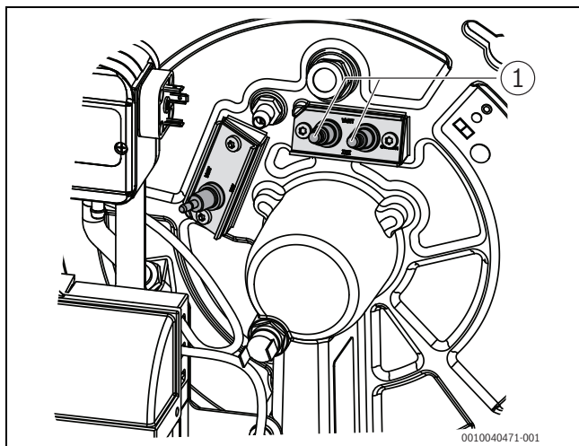
Fig. 21 Tændelevtrode
