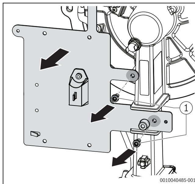
Bild 13 Halteblech demontieren
