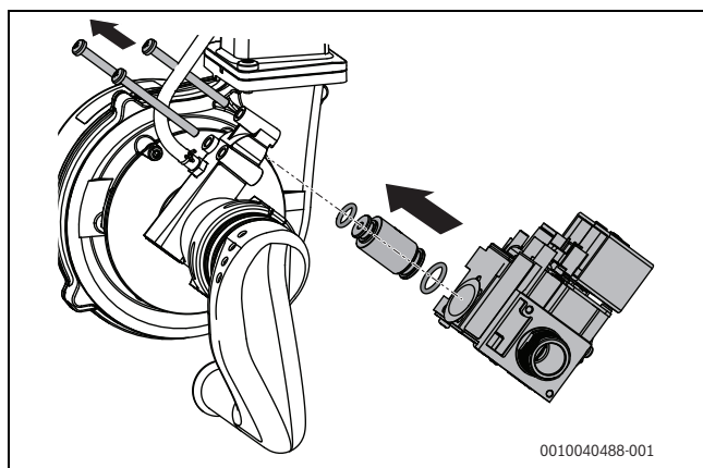
Fig. 46 Remplacer l'injecteur
