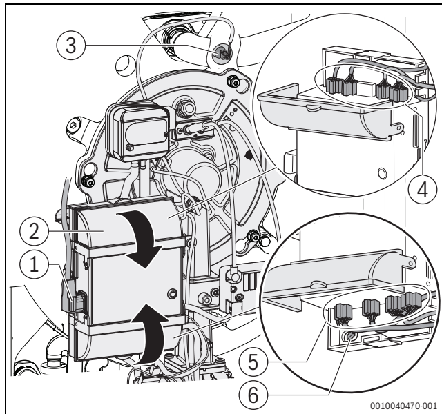
Bild 3 Steckverbindungen lösen
