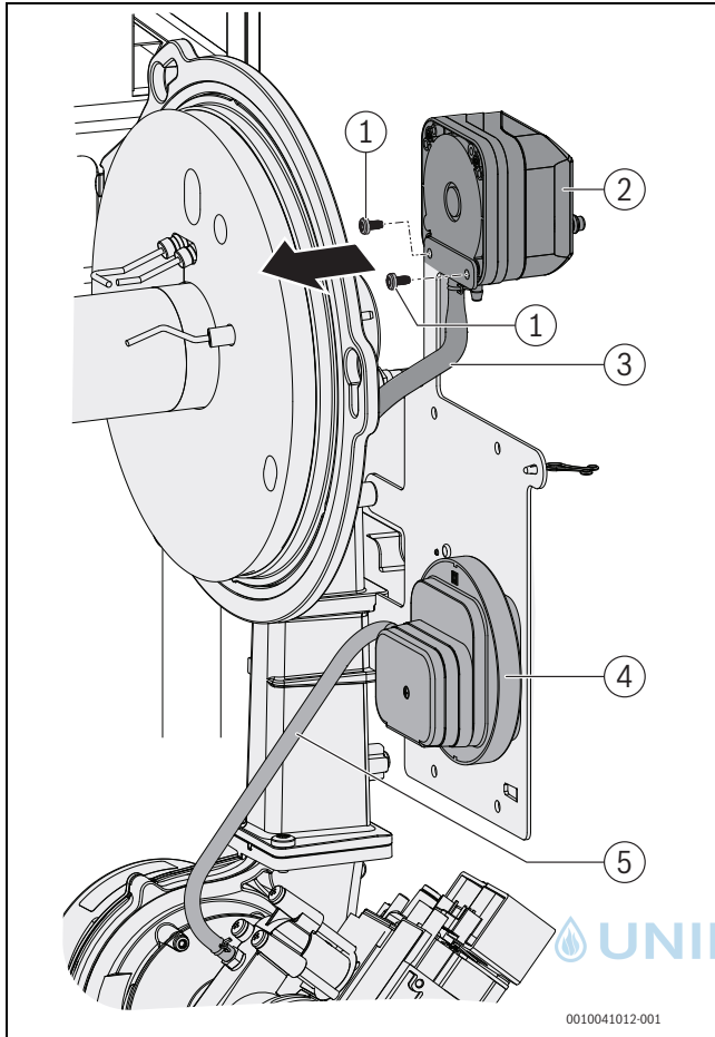
Fig. 59 Smontare il pressostato basso carico e camera di combustione
