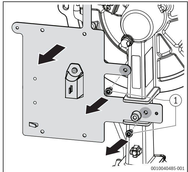
Afb. 77 Bevestigingsplaat demonteren
