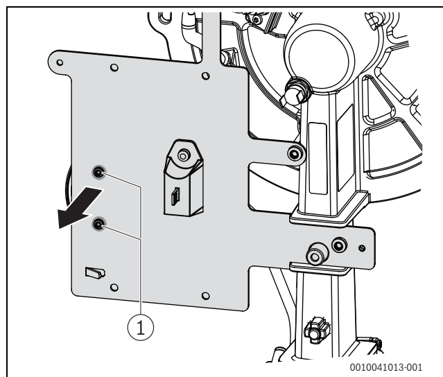
Bild 12 Kleinlast-Druckwächter demontieren
