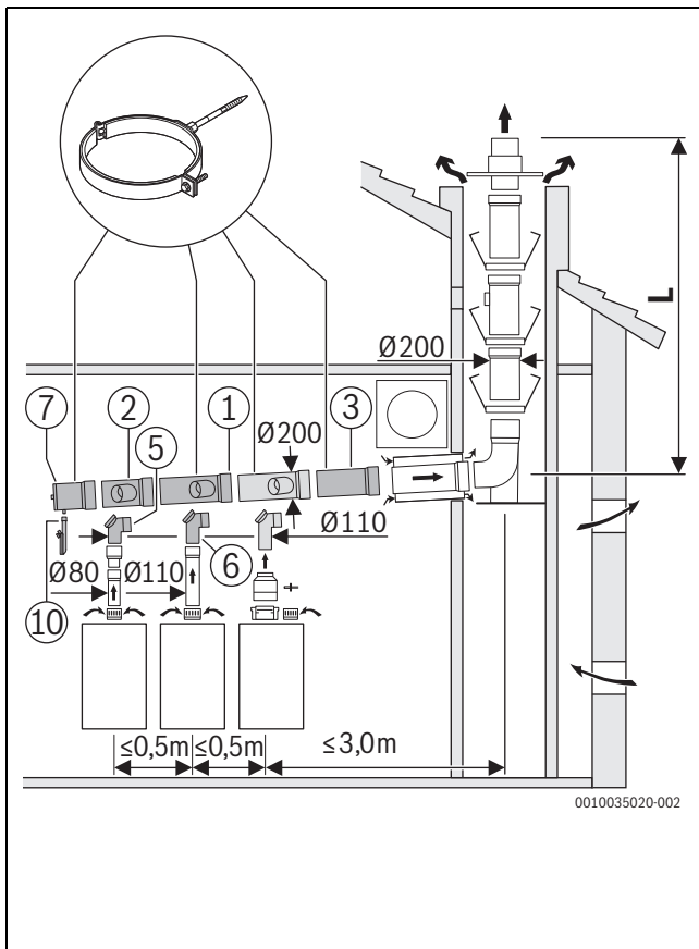
9 DN200 - DN200
