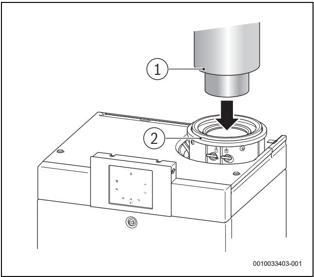
Bild 1 Konzentrisches Rohr (raumlufunabhängig)
