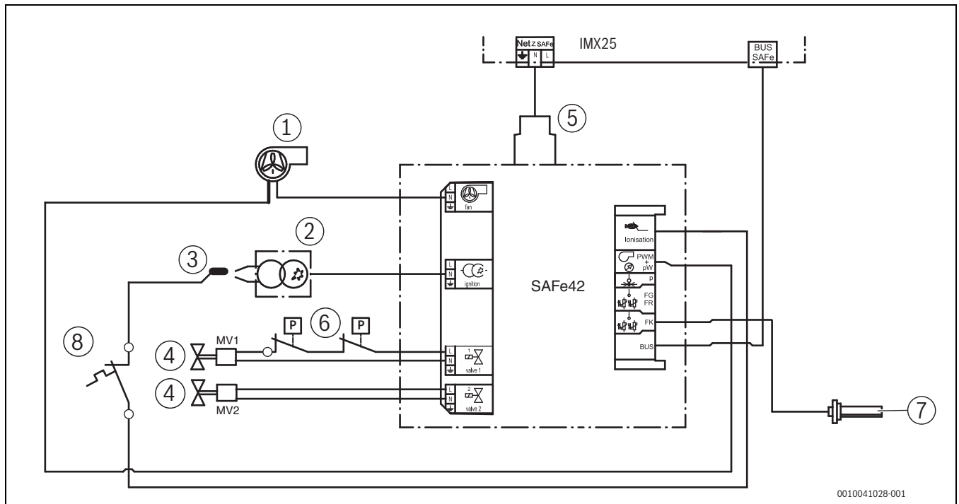
Bild 57 Anschlussplan Feuerungsautomat
