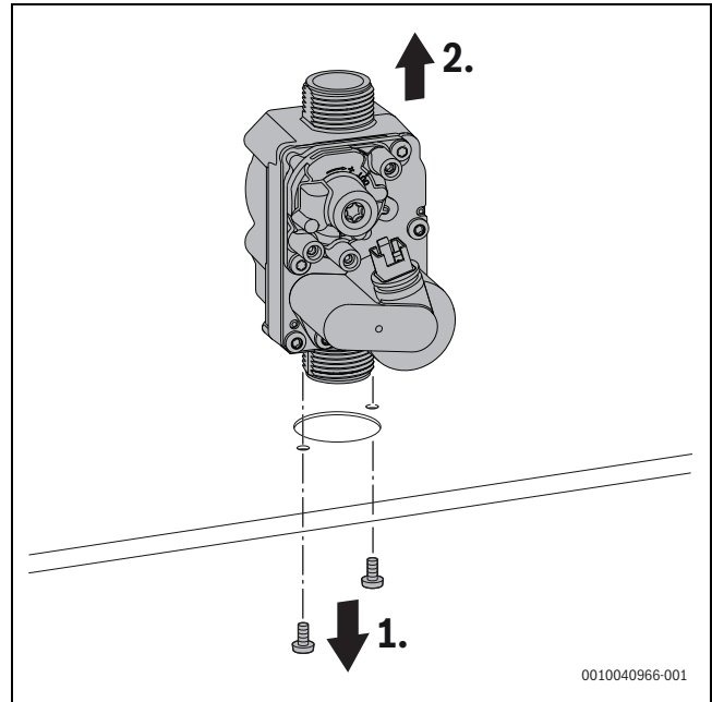
Bild 87 Gasarmatur ausbauen
