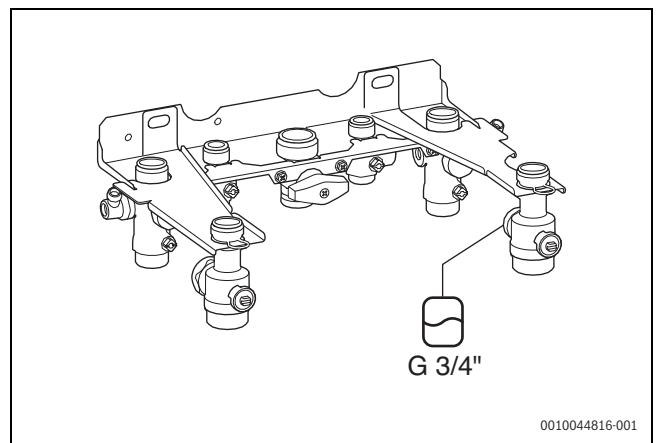
Bild 38 Ausdehnungsgefäß anschließen
