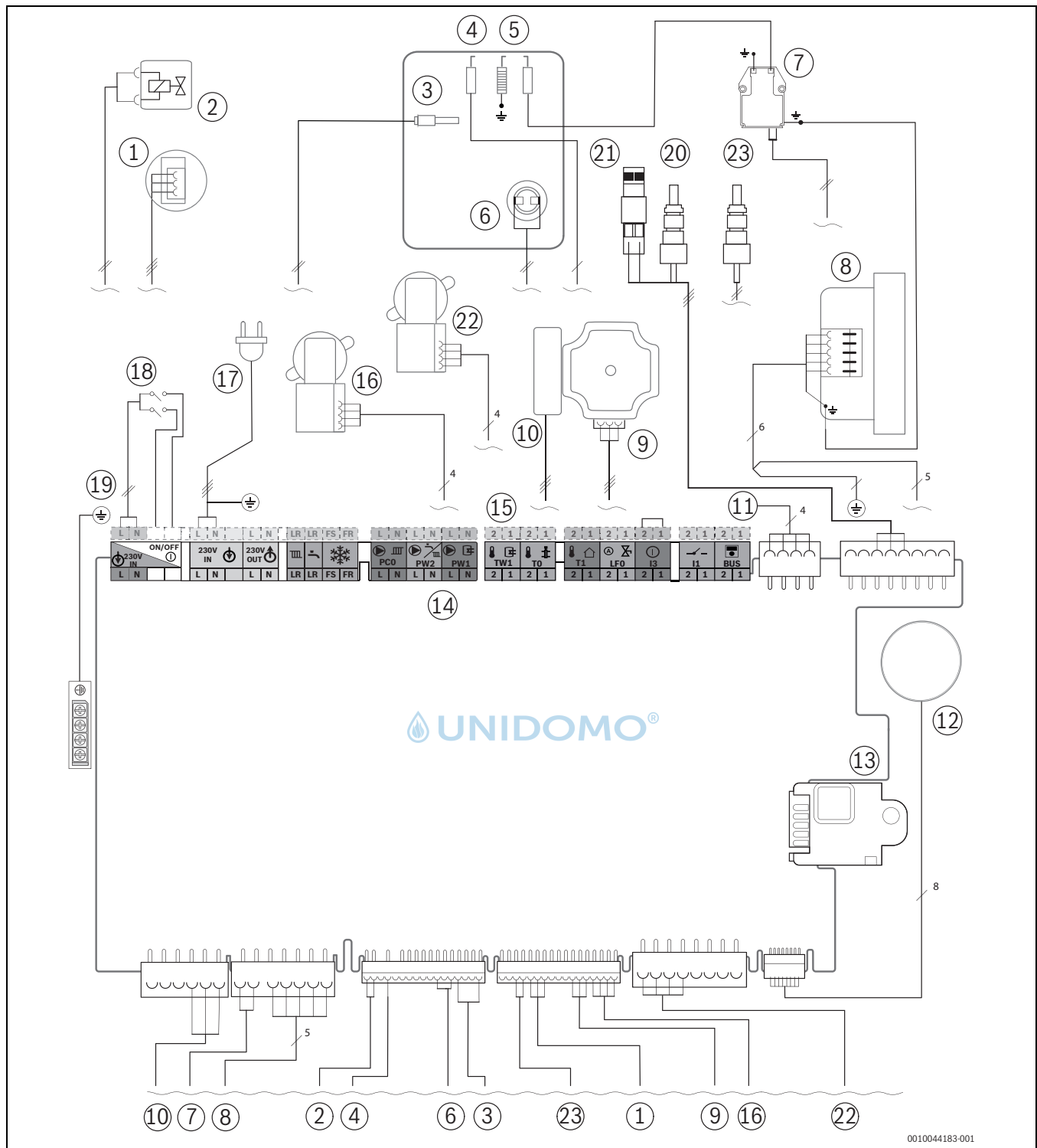
Bild 98 Elektrische Verdrahtung
