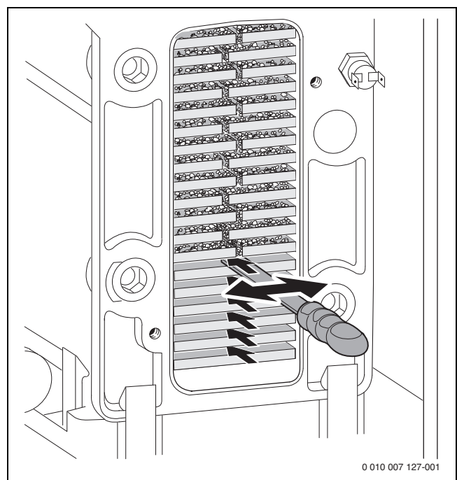
Bild 88 Reinigungsmesser
