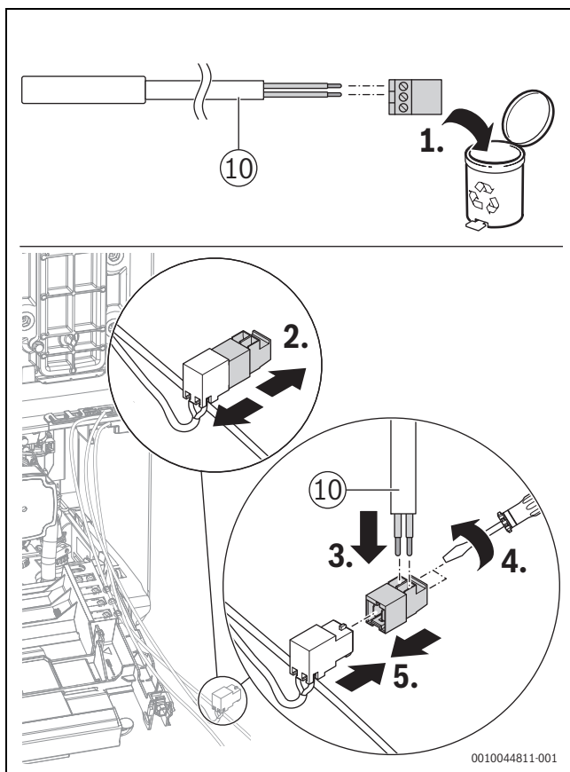
Bild 57 Pufferspeicher-Temperaturfühler anschließen
