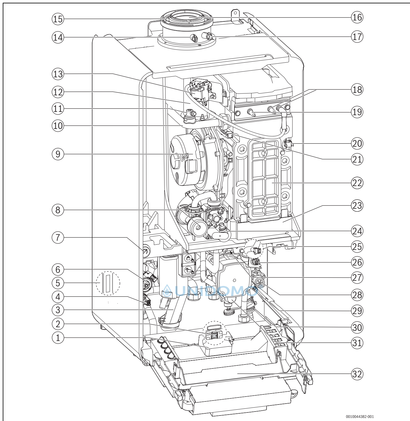
Bild 4 Produktübersicht
