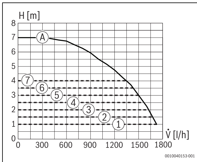
Bild 97 Pumpenkennfelder und Pumpenkennlinien
