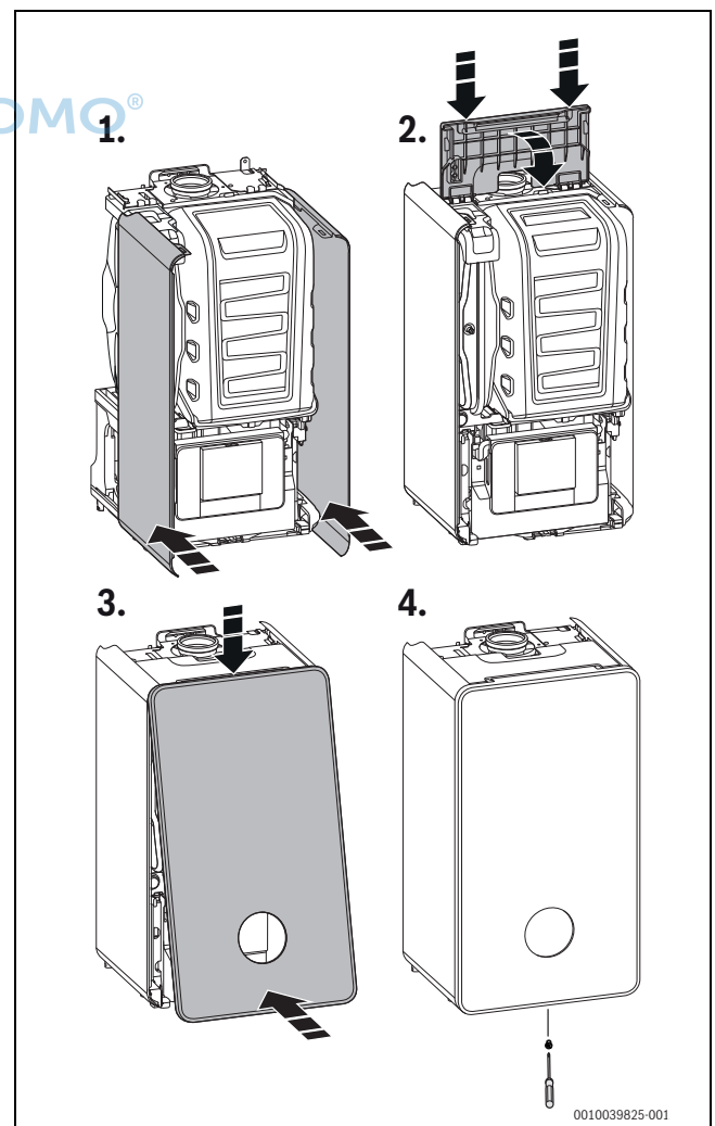
Bild 64 Verkleidung montieren
