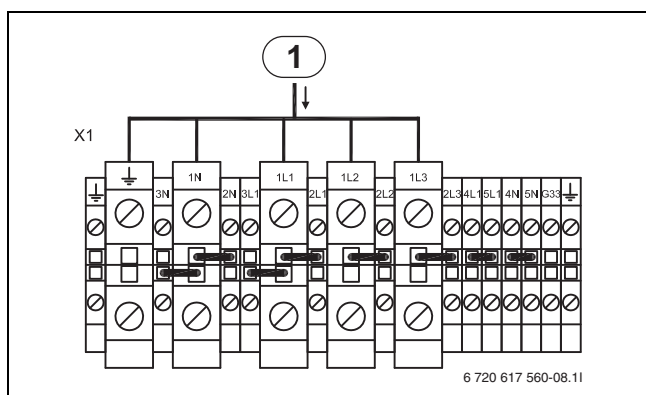
Bild 23 Standardausführung, STE 130-1 - 170-1
