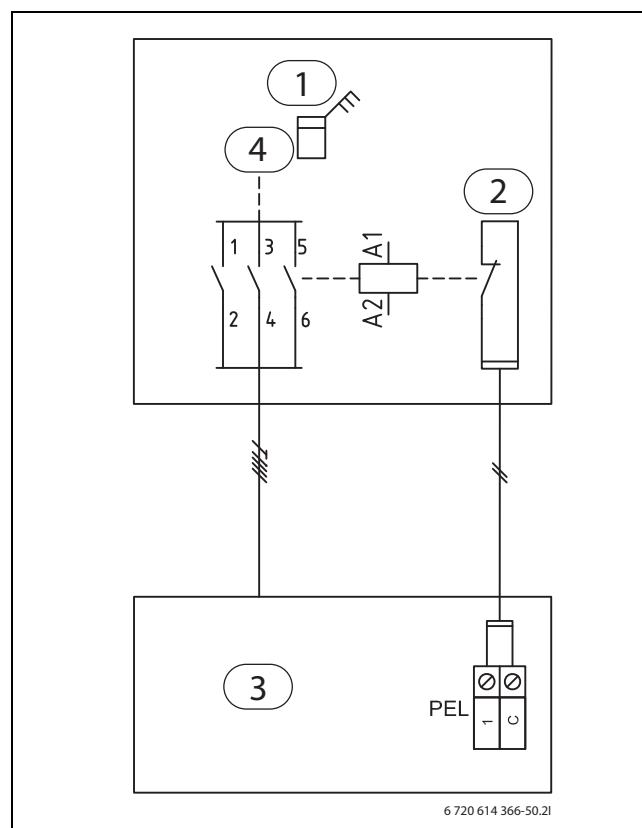
Bild 17 Sperrzeit aktiv
