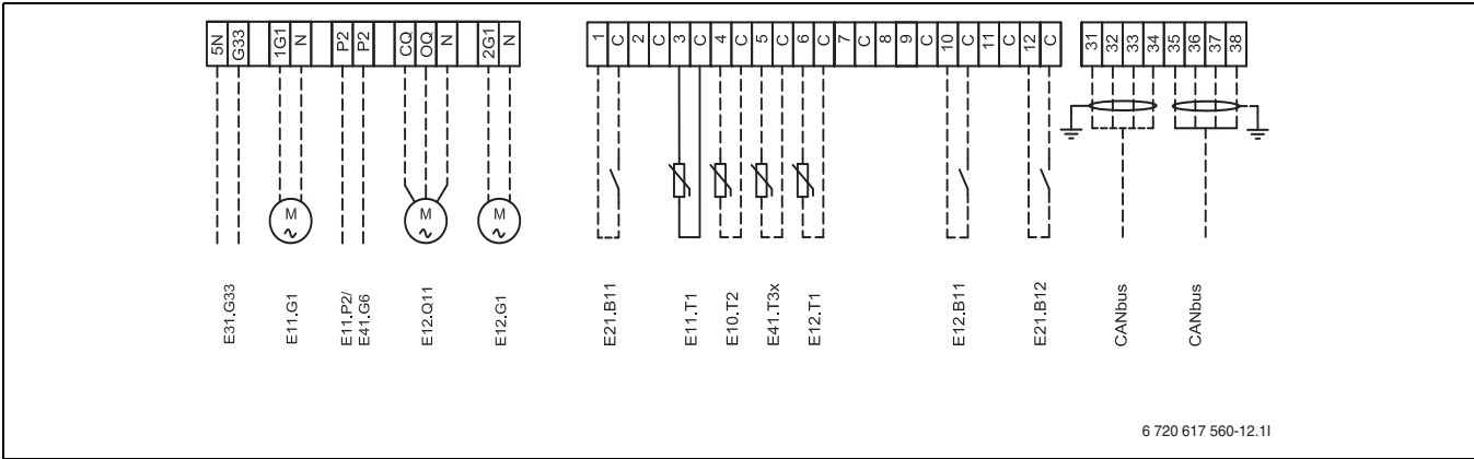
Bild 27 Externe Anschlüsse
