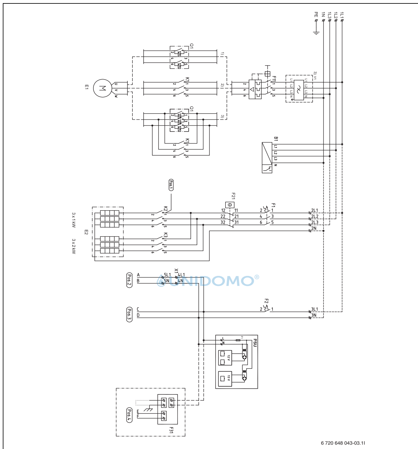
Bild 29 Interner Schaltplan
