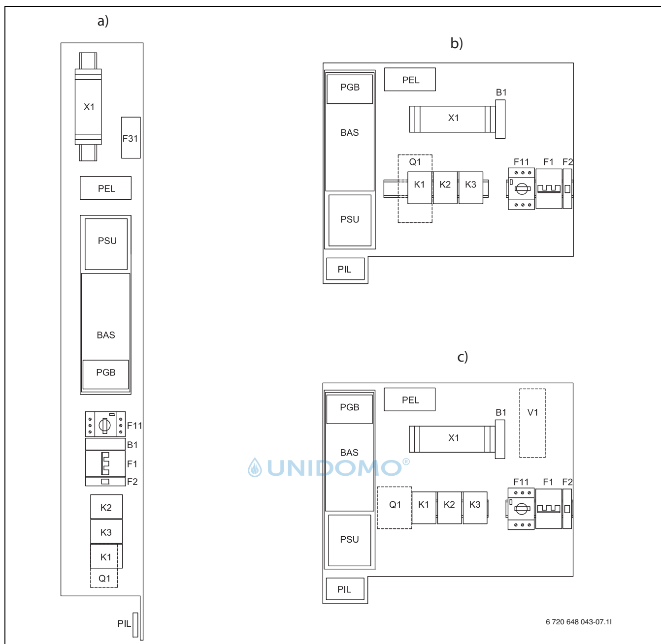
Bild 14 Übersicht Leiterplatte
