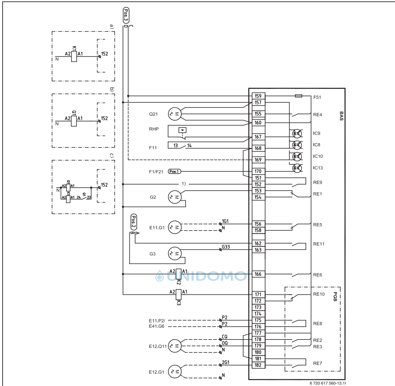
Bild 30 Kompletter Anschlussschaltplan (230 V)
