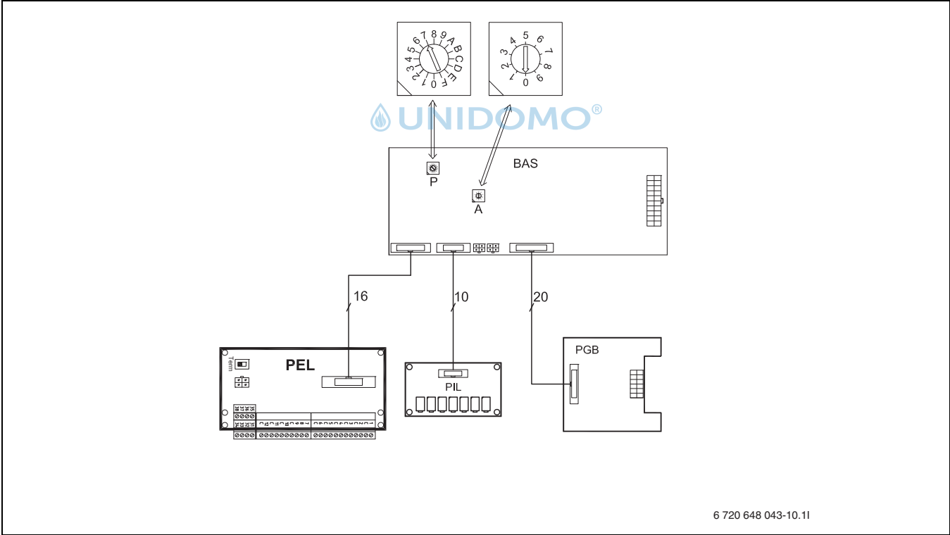
Bild 16 Leiterplattenverbindungen
