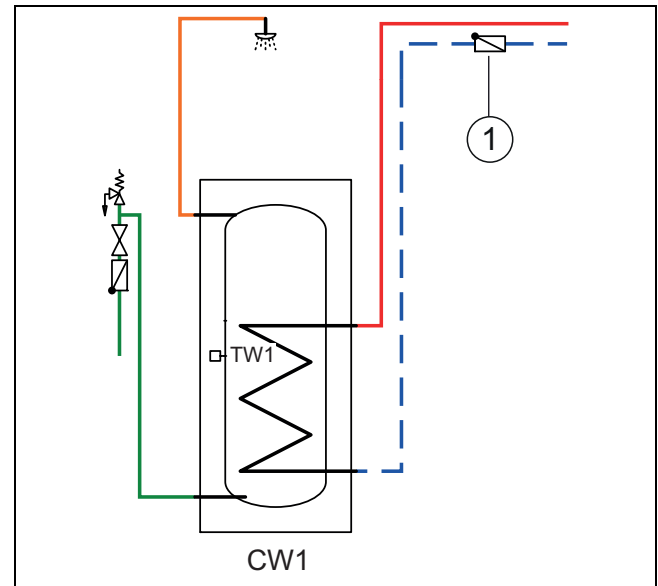
Bild 19 Warmwasserspeicher
