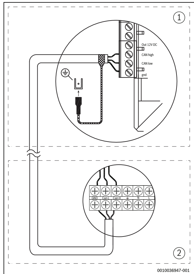
Bild 12 CAN-BUS-Verbindung
