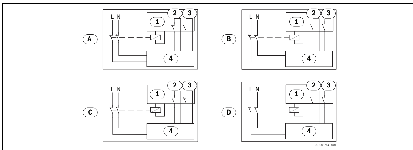
Bild 47 Anschlussplan für EVU/SG (1-phasig)
