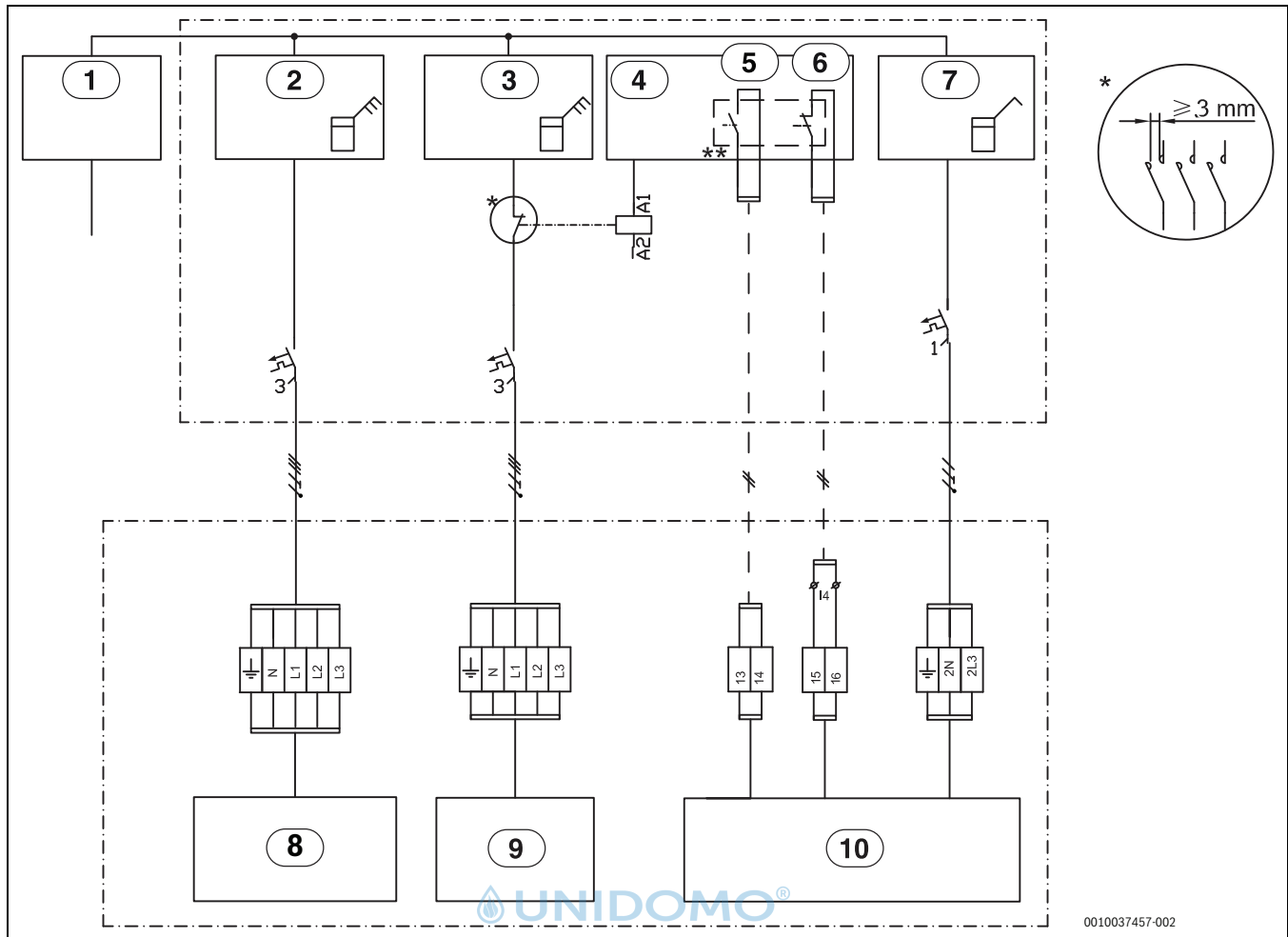
Bild 51 EVU Typ 3
