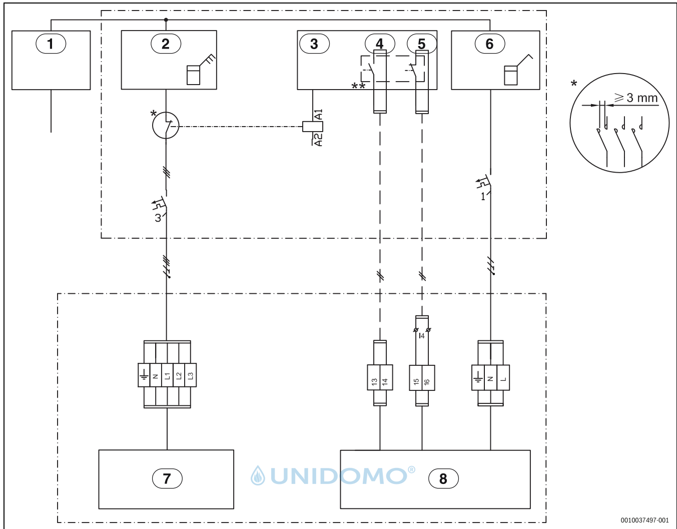
Bild 46 EVU 2, nur Ausschalten des Kompressors
