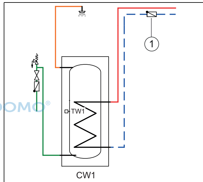
Bild 21 Warmwasserspeicher
