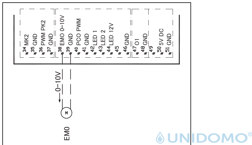
Bild 17 0- bis 10-V-Ansteuerung für externe Zuheizer
