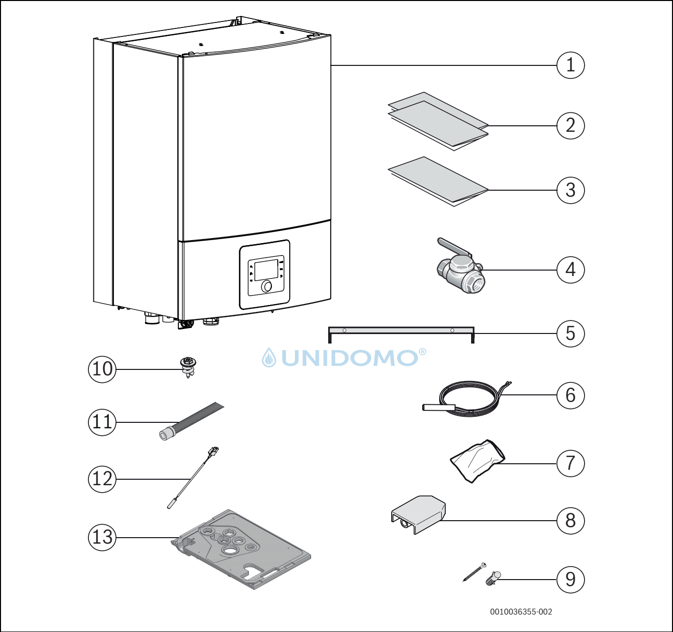
Bild 2 Lieferumfang
