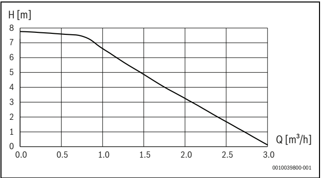
Bild 29 Leistungskurve der Primärumwälzpumpe (PC0)
