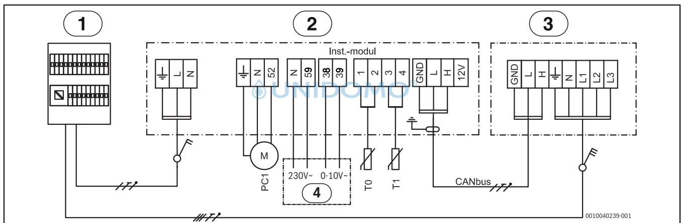
Bild 40 Schaltplan
