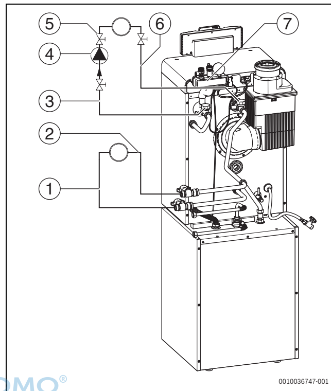
Bild 23 Anschlusschema Hydraulik OC8000i FM (Beispiel mit Anschluss-Set Heizkreis links/rechts für 2 Heizkreise)
