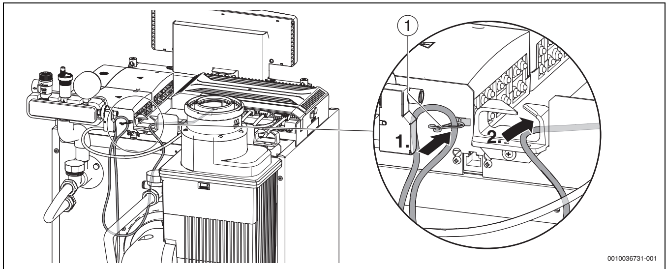
Bild 16 Fühlerkabel befestigen und einstecken (Kessel)
