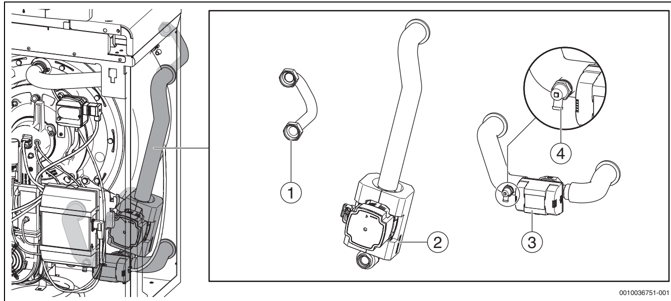
Bild 30 Übersicht Bauteile der internen Hydraulik
