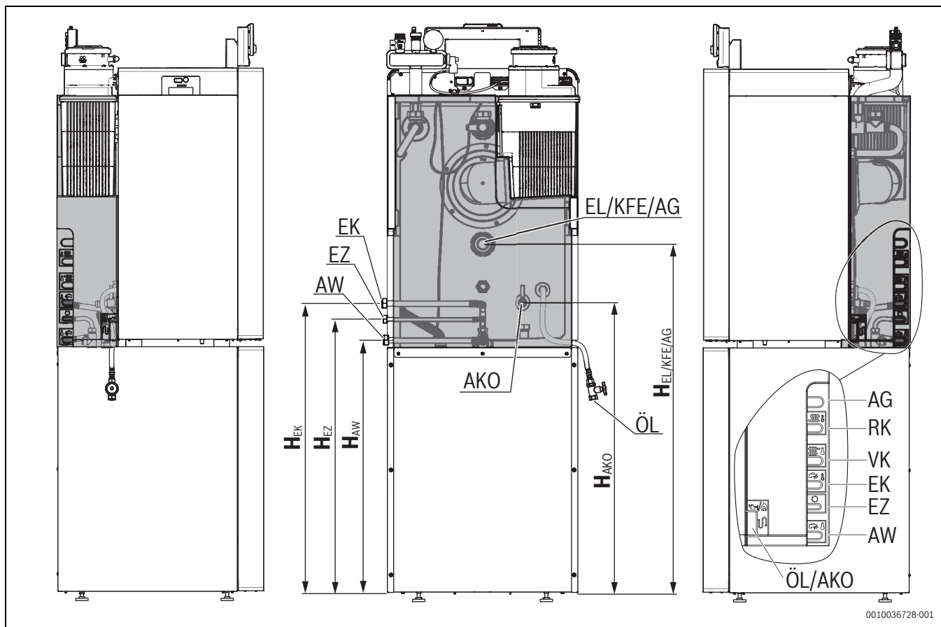
Bild 4 Anschlüsse und Abmessungen (Trinkwasser, Öl, Kondensat) am Heizkessel mit untergestelltem Warmwasserspeicher, OC8000i FM 19/25, (Maße in mm; teilweise mit Wärmeschutz dargestellt; Darstellung enthält Zubehör)
