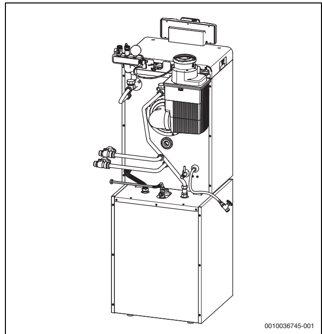
Bild 21 Rohre Zirkulation zur Anbindung links oder rechts (in Abbildung dargestellt) montieren
