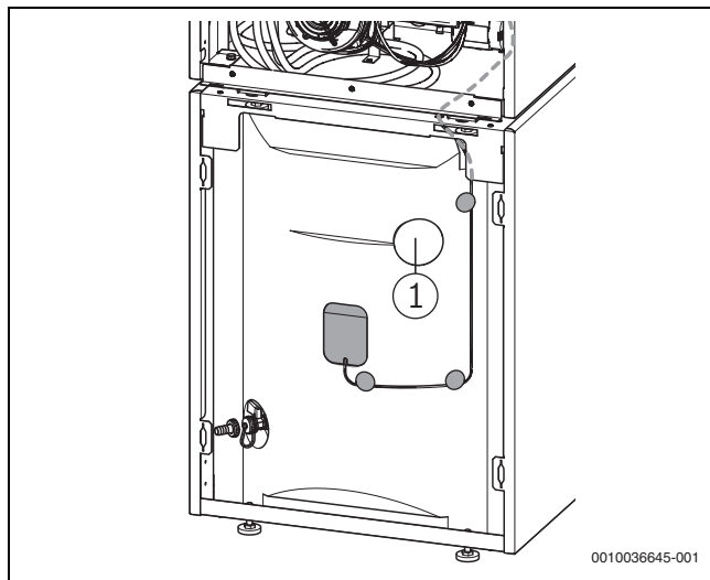
Bild 33 Position Schutzanode
