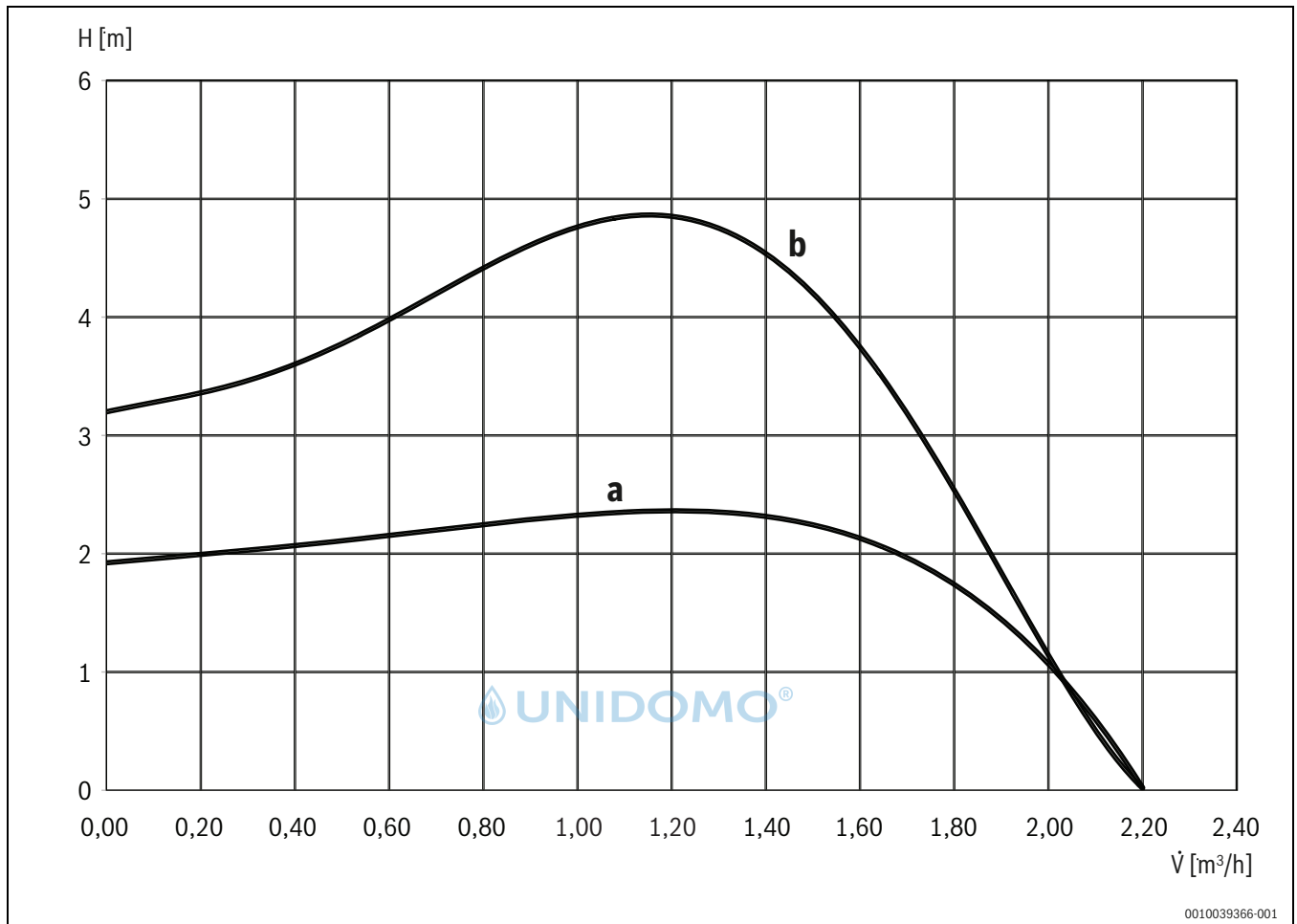
Bild 26 Restförderhöhe OC8000i FM 19/OC8000i FM 25 mit integrierter Hocheffizienzpumpe Grundfos UPM3 AUTO 15-70 130
