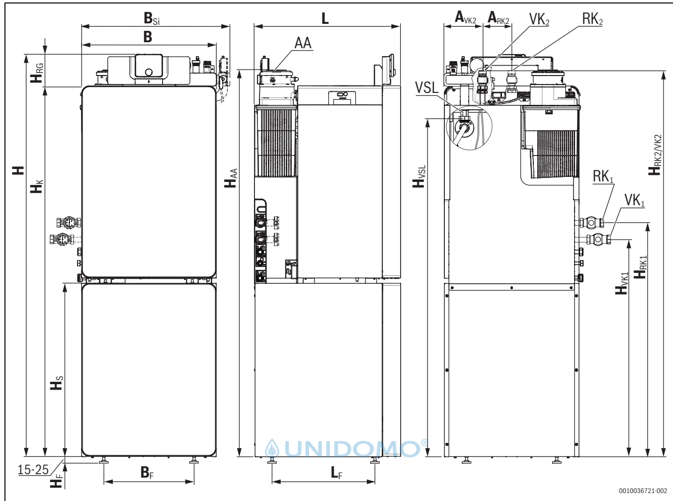
Bild 3 Anschlüsse und Abmessungen am Heizkessel mit untergestelltem Warmwasserspeicher, OC8000i FM 19/25, (Maße in mm; Darstellung enthält Zubehör)
