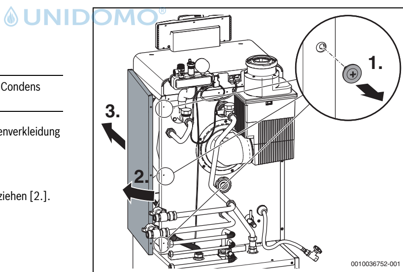
Bild 31 Seitenverkleidung demontieren
