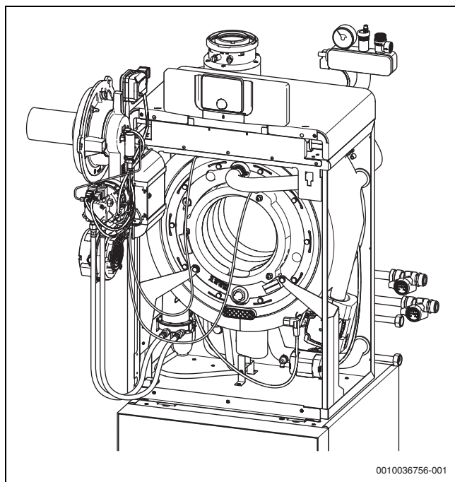
Bild 32 Brenner in Serviceposition links bringen
