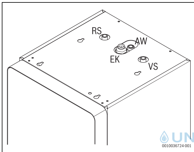
Bild 5 Hydraulische Anschlüsse Warmwasserspeicher
