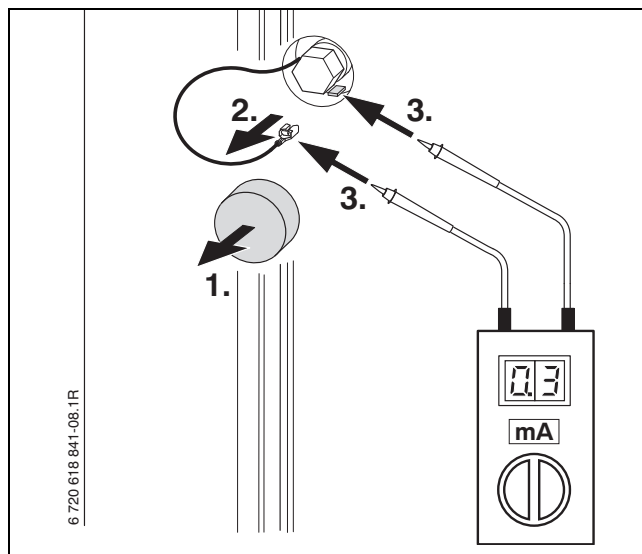
Bild 34 Schutzanode prüfen
