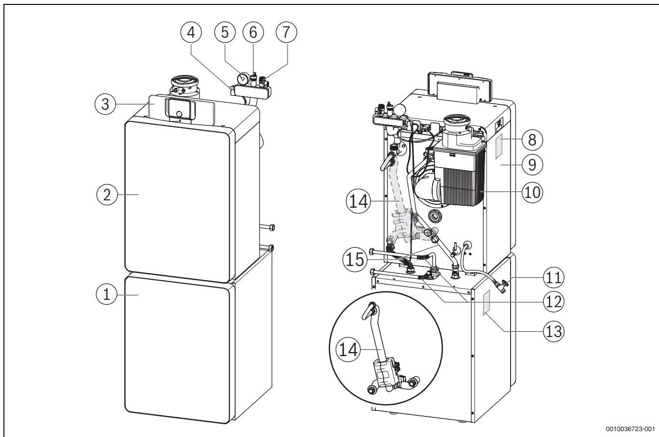
Bild 2 Hauptbestandteile Heizkessel inkl. Speicher und Verrohrung
