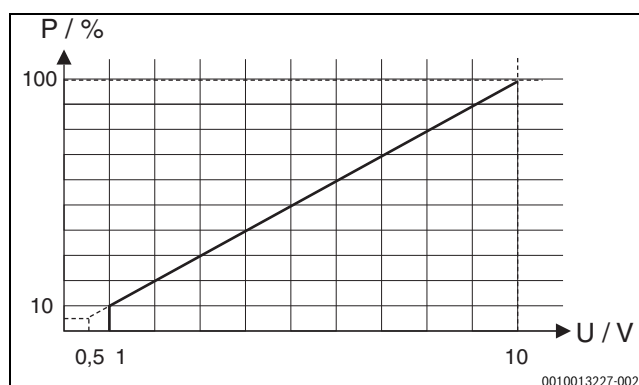
Afb. 1 Lineaire relatie tussen 0-10 V-sigitaal (U in Volt) en gevraagde vermogen P (in procenten gerelateerd aan het maximale vermogen van de installatie)
