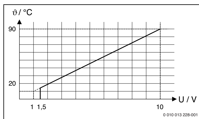
Bild 2 Linearer Zusammenhang zwischen 0-10V-Signal ( U in Volt) und angeforderter Vorlauftemperatur \theta (in °C bezogen auf den Bereich minimale Vorlauftemperatur bis maximale Vorlauftemperatur [Grundeinstellung 20 °C bis 90 °C])
