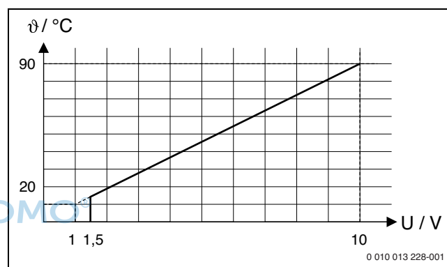
图2 0-10 V 信号 ( U 单位为 V) 和要求的出水温度 \theta (单位为 ^{\circ}\text{C} ，以最低出水温度至最高出水温度的范围为准 [基本设置 20^{\circ}\text{C} 至 90^{\circ}\text{C} ]) 之间的线性关系
