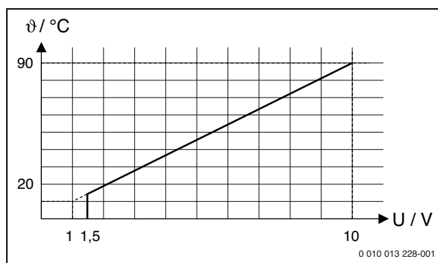
Afb. 2 Lineaire relatie tussen 0-10 V-sigitaal (U in Volt) en gevraagde aanvoertemperatuur θ (in °C gerelateerd aan het bereik minimale aanvoertemperatuur tot maximale aanvoertemperatuur [basisinstelling 20 °C tot 90 °C])
