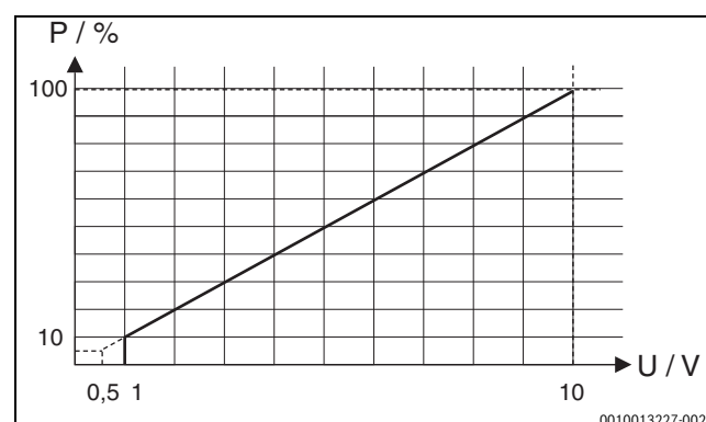
Fig. 1 Relazione lineare tra segnale 0-10 V (tensione elettrica in V) e potenza richiesta P (in percentuale, riferita alla potenza massima dell'impianto)
