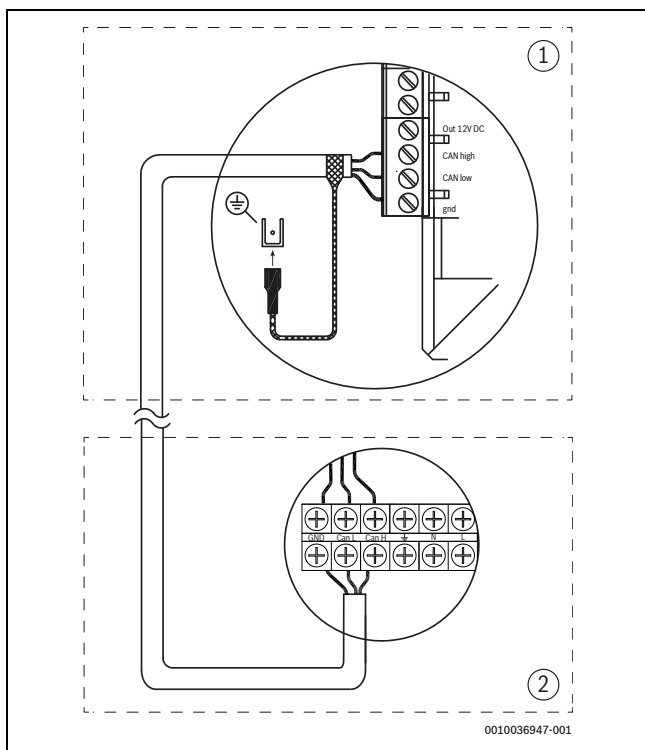
Bild 18 CAN-BUS-Verbindung
