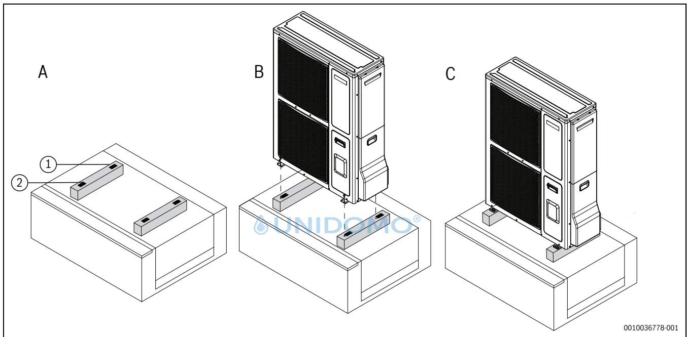
Bild 7 Bodenstehende Außeninheit
