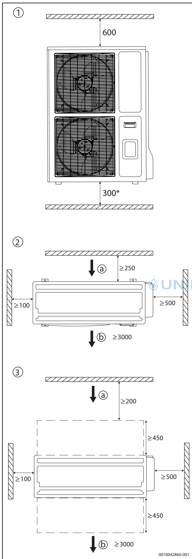
Bild 3 Mindestabstände (mm)
