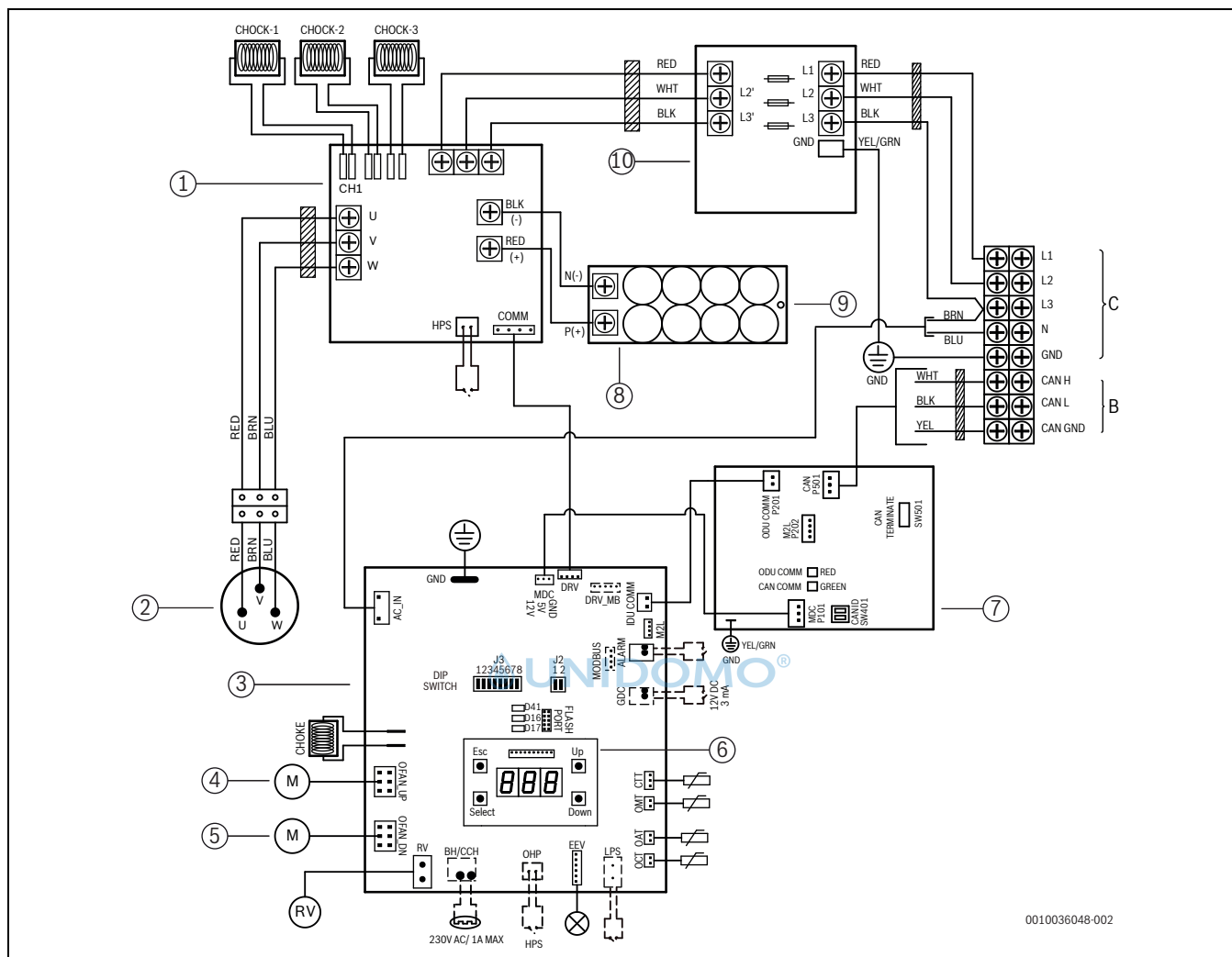
Bild 26 Schaltplan für dreiphasige Außenanlage CS3400iAWS 10-14 OR-T
