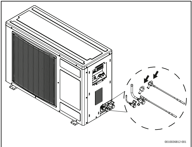
Bild 15 Verschraubung
