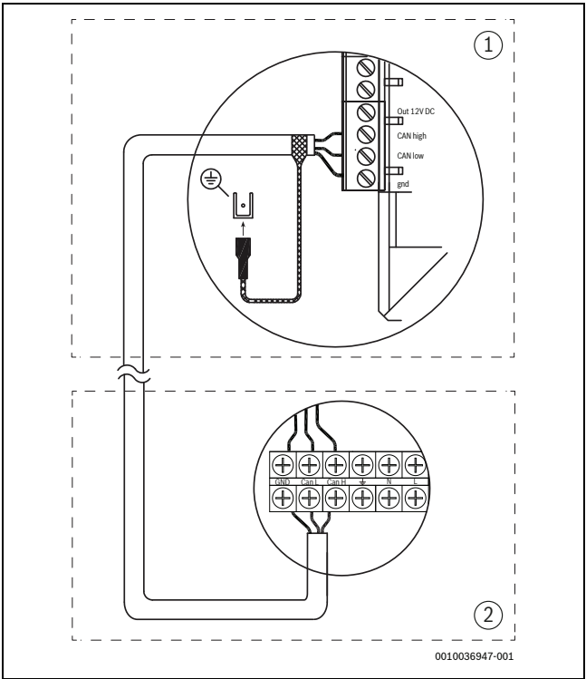
Bild 20 CAN-BUS-Verbindung
