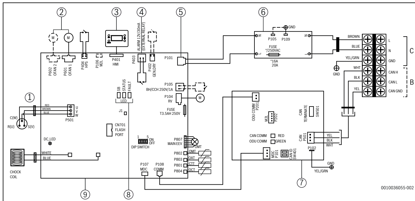
Bild 27 Schaltplan für einphasige Außenanlage CS3400iAWS 6 OR-S CS3400iAWS 8 OR-S und CS3400iAWS 10 OR-S
