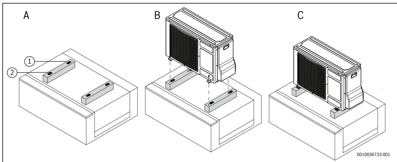
Bild 9 Bodenstehende Außeneinheit
