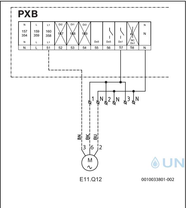
Bild 25 Schaltplan 3-Wege-Umschaltventil
