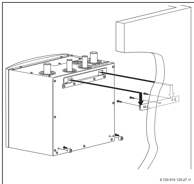
Bild 15 Montage
