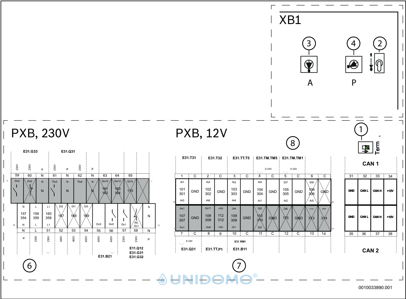
Bild 23 Schaltplan PXB
