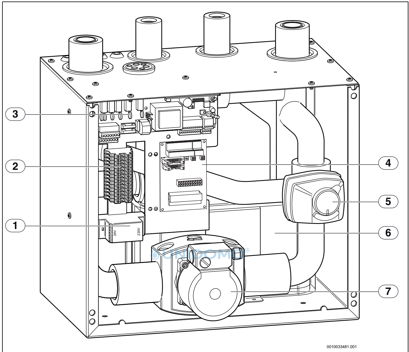
Bild 8 Komponenten
