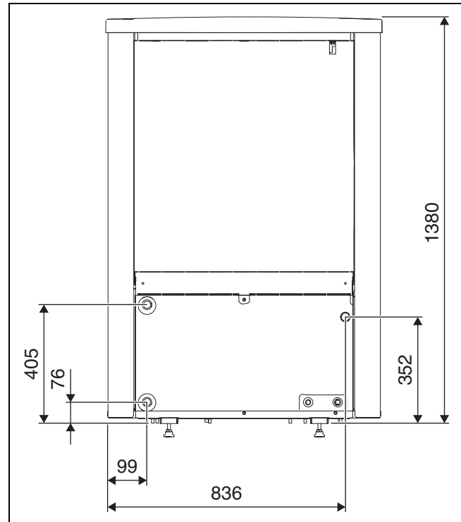
Bild 4 Abmessungen und Anschlüsse der Wärmepumpenmodelle 5 OR-S-9 OR-S, Rückseite
