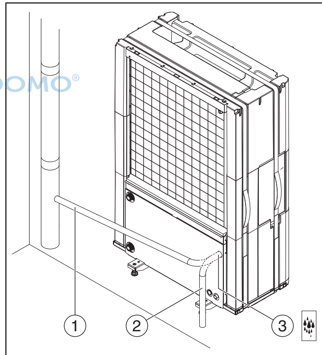
Bild 17 Kondensatrohranschlüsse, gültig für alle Größen
