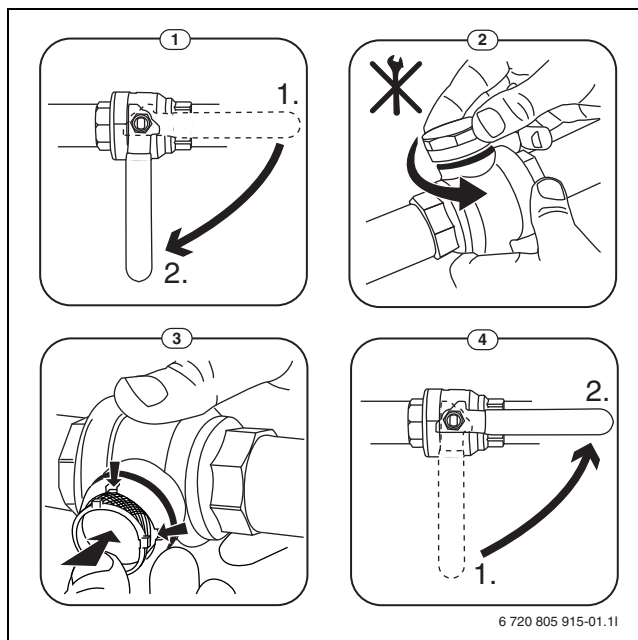
Bild 22 Siebreinigung
