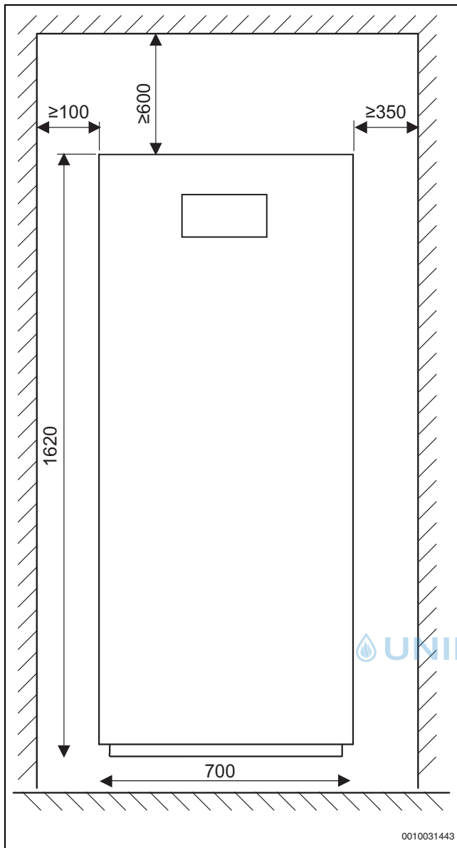
Bild 4 Abmessungen der Wärmepumpe 22–28 kW
