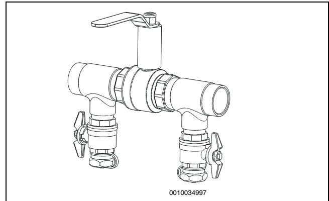
Bild 17 Befüllschiene in Befüllposition
