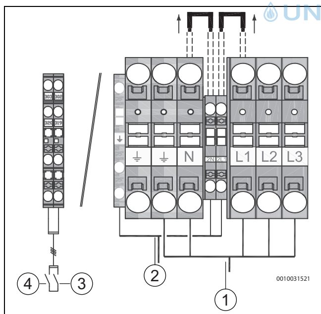
Bild 38 Belegung bei Stromversorgung im Niedertarif
