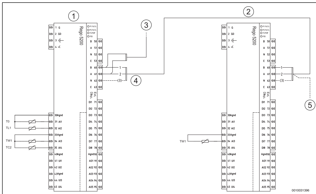
Bild 49 Schaltplan Kaskadenschaltung
