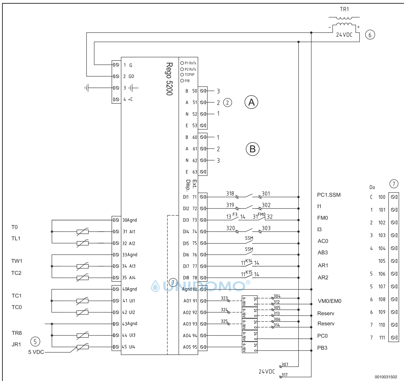
Bild 32 Schaltplan mit Sammelalarm für Anlaufstrombegrenzer (22–28 kW)
