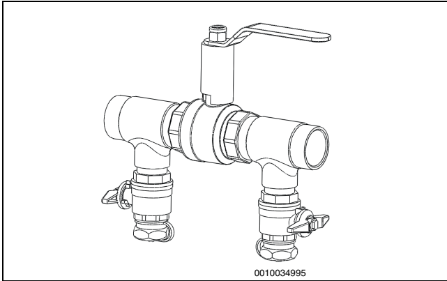
Bild 15 Befüllstation
