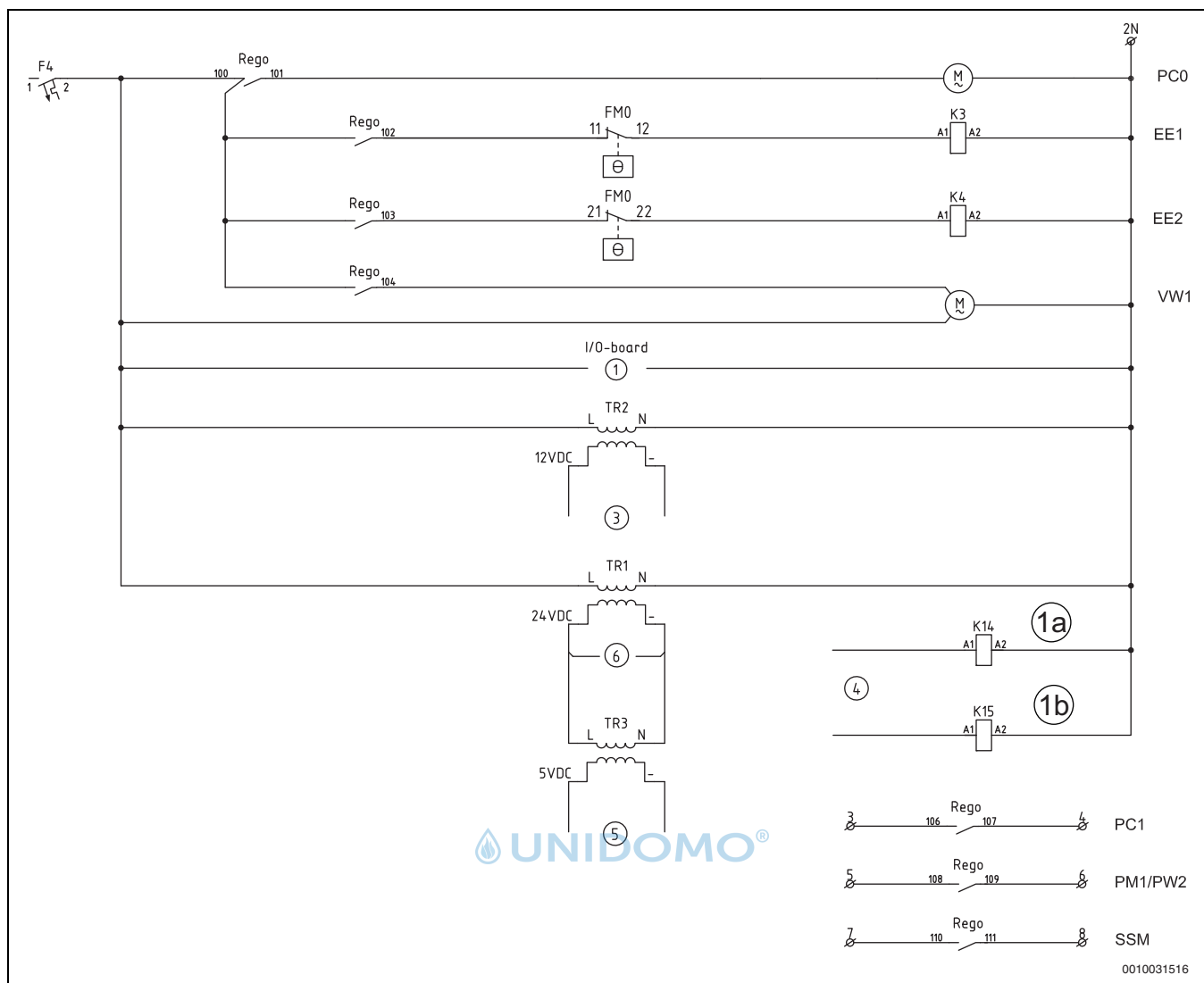
Bild 35 Schaltplan 22–28 kW
