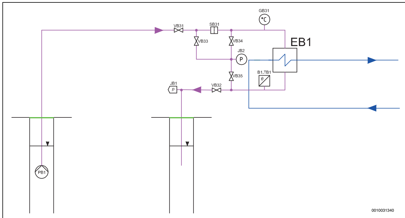
Bild 54 Grundwassersystem
