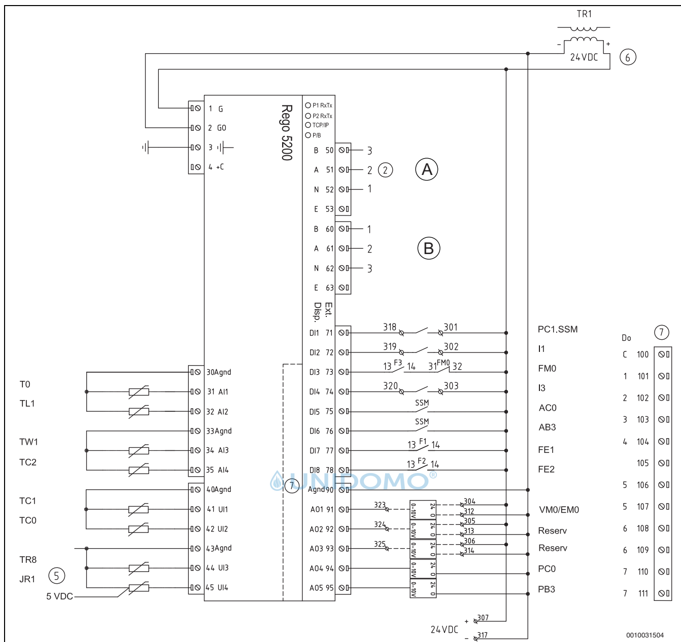
Bild 31 Schaltplan mit Steuerungssicherung (22–28 kW)
