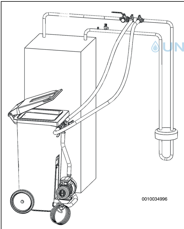
Bild 16 Befüllen mit Befüllstation
