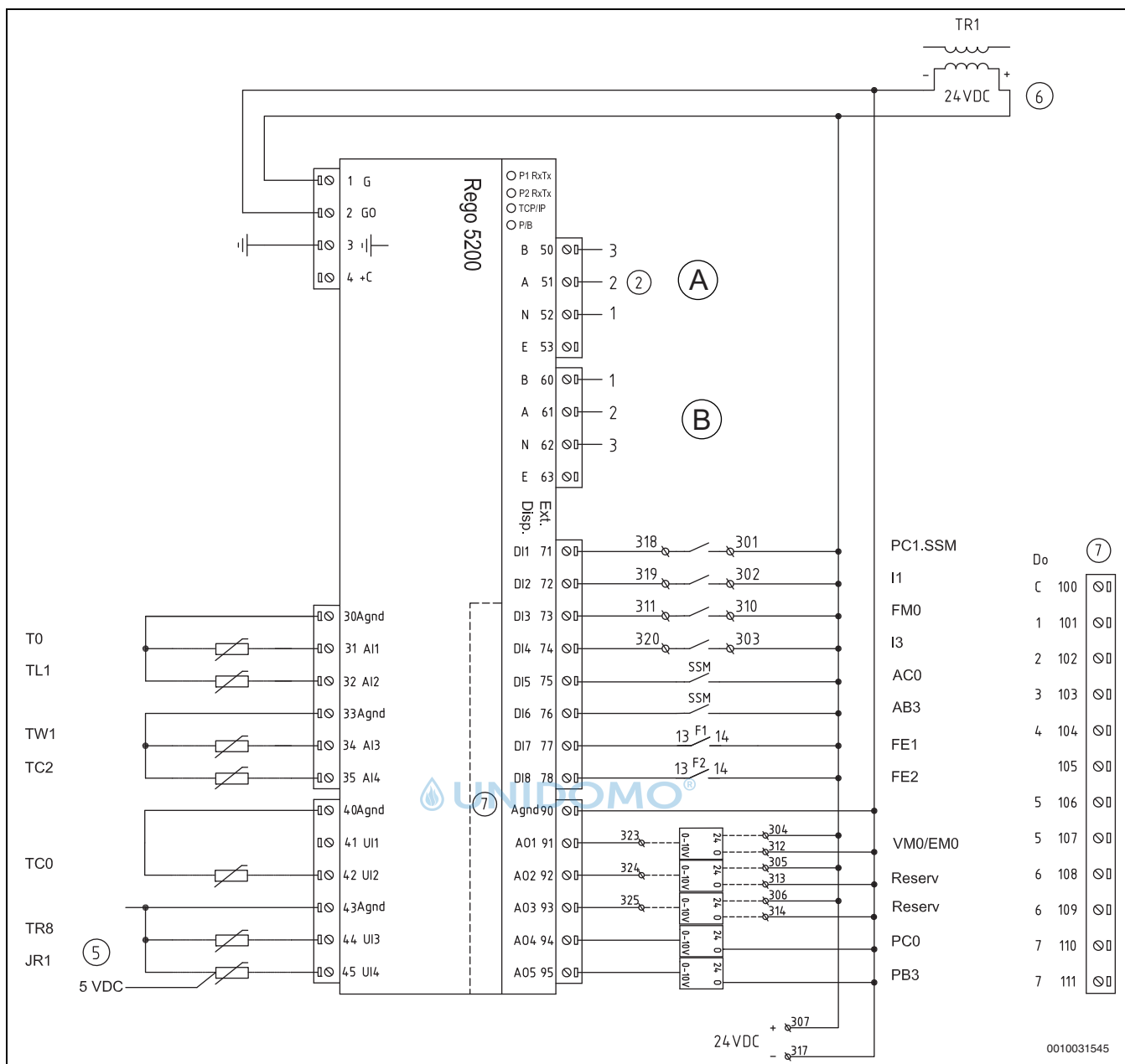
Bild 43 Schaltplan mit Steuerungssicherung (38–48 kW)
