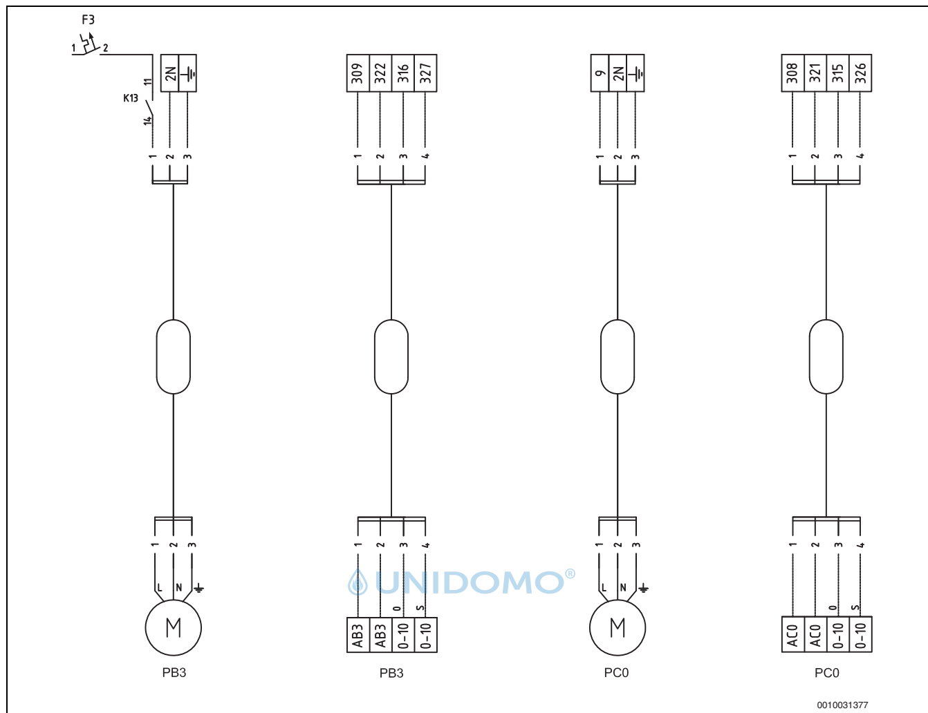
Bild 32 Anschluss Solekreispumpe/Heizkreispumpe
