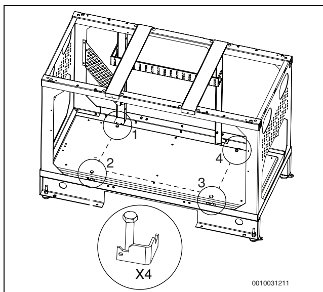
Bild 6 Transportsicherungen, Wärmepumpe
