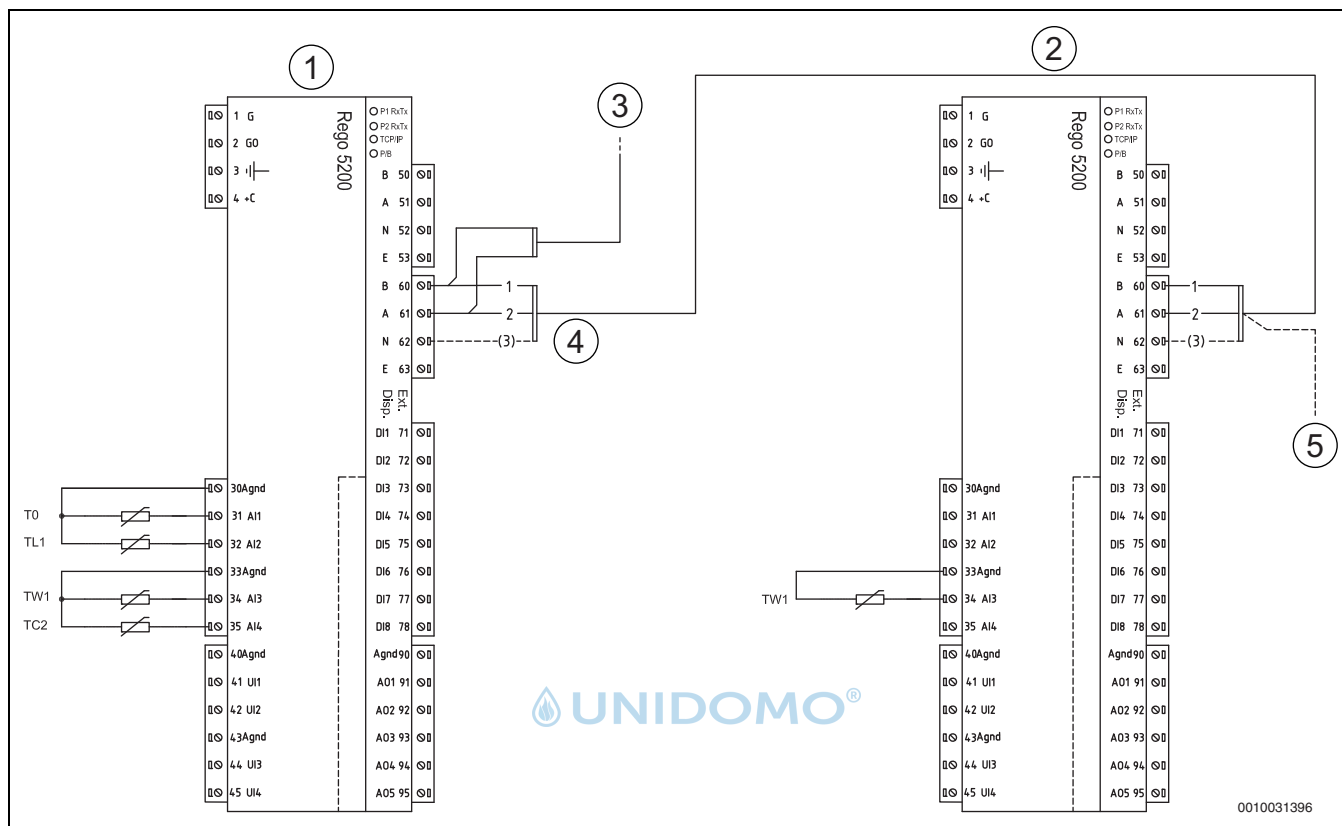
Bild 33 Schaltplan Kaskadenschaltung
