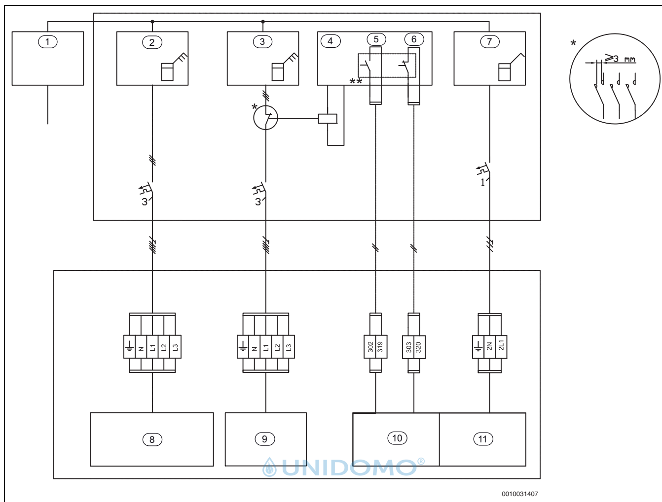
Bild 37 EVU Typ 3 mit Abschaltung von Kompressor und Elektro-Heizeinsatz
