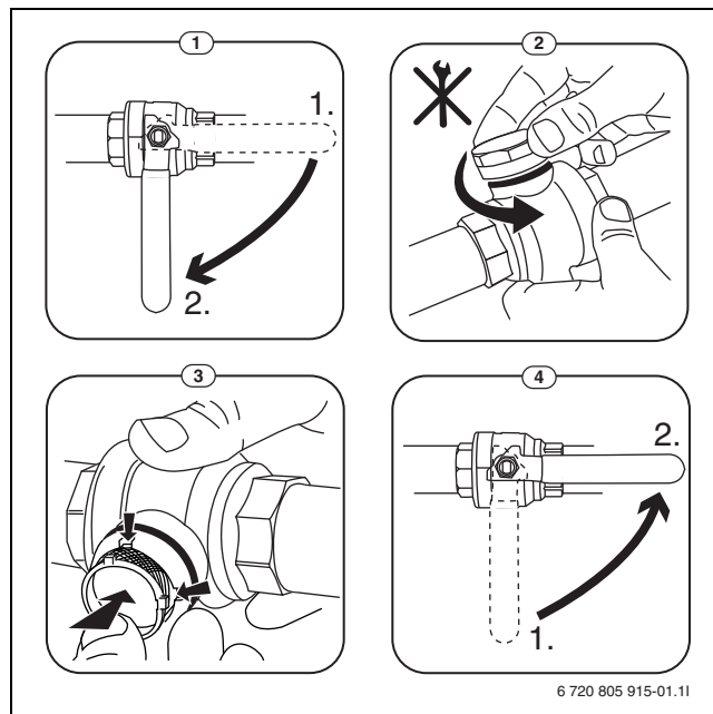
Bild 15 Siebreinigung
