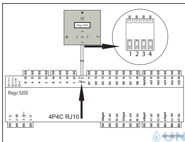
Bild 19 Überblick Klemmenkasten
