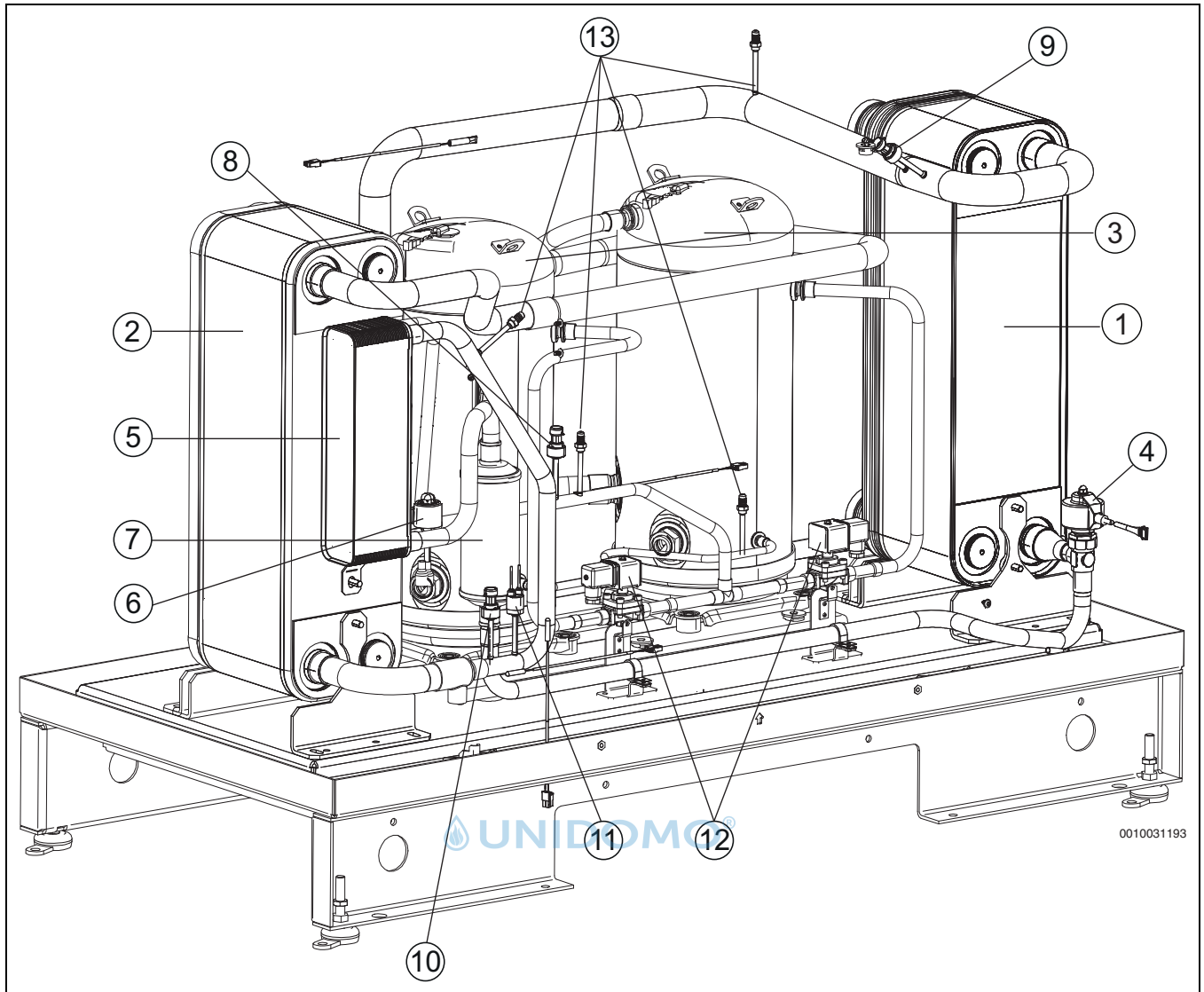
Bild 2 Produktübersicht
