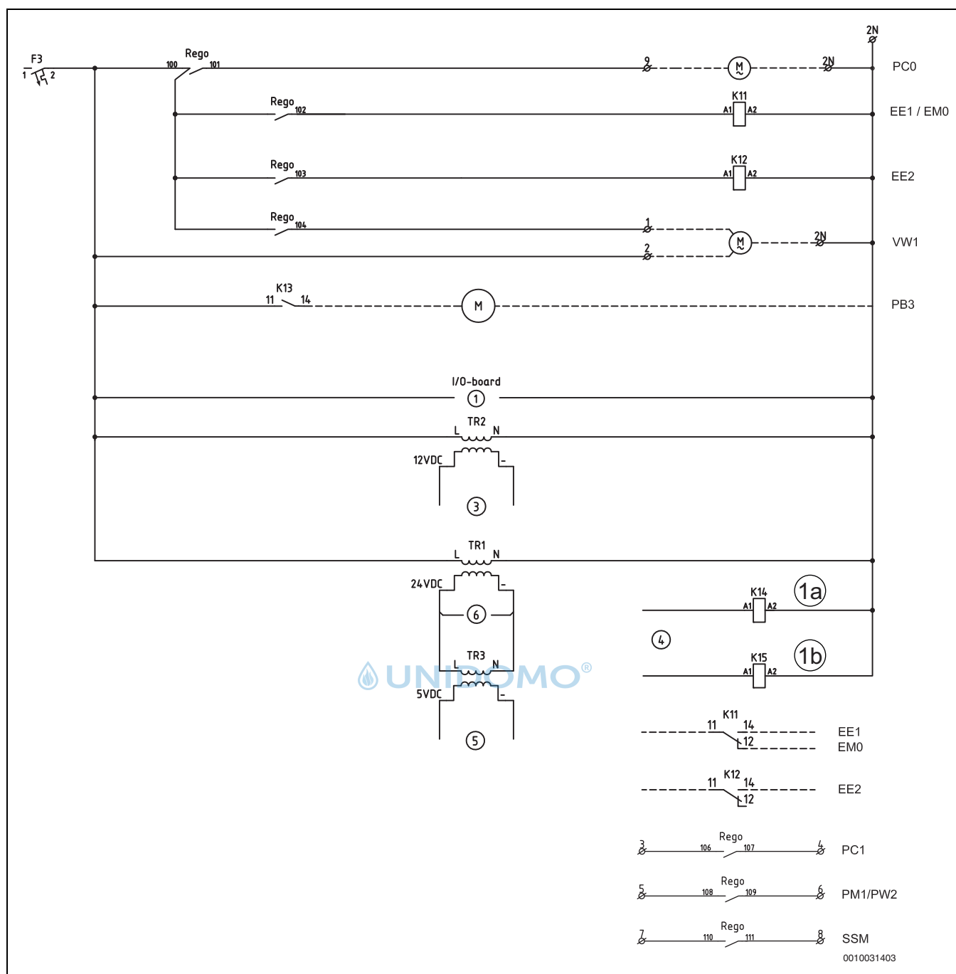
Bild 30 Schaltplan Wärmepumpe
