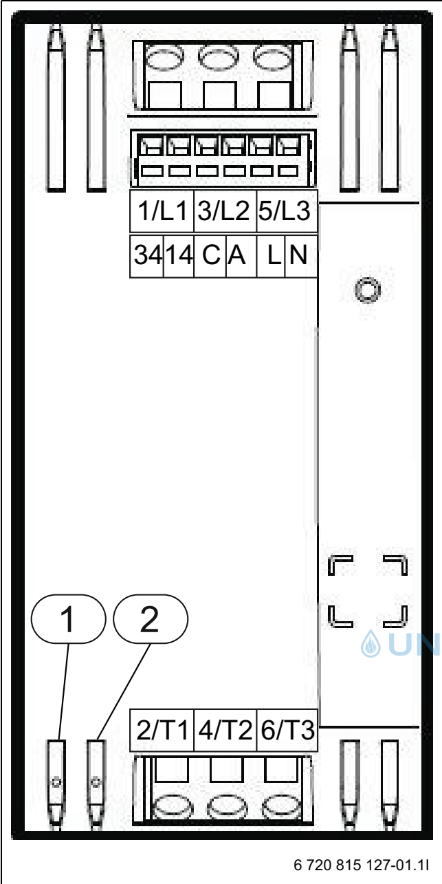
Bild 5 Sanftanlauf
