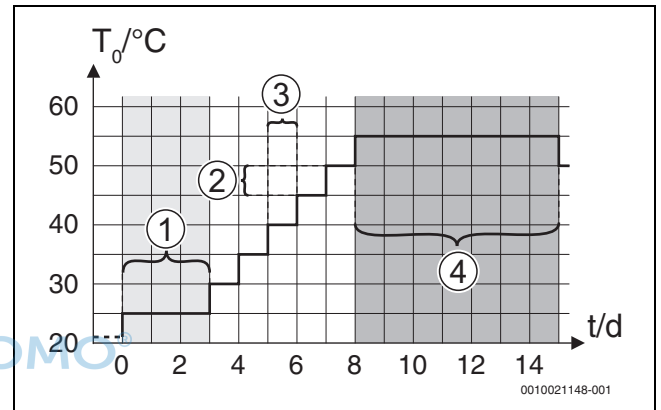
Bild 6 Ablauf der Estrichtrocknung mit den Grundeinstellungen in der Aufheizphase
