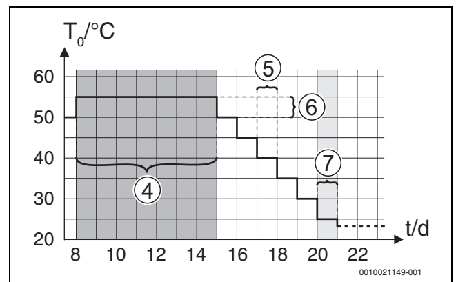
Bild 7 Ablauf der Estrichtrocknung mit den Grundeinstellungen in der Abkühlphase
