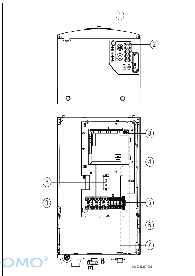
Bild 10 Kabeldurchführungen (Ansicht von unten und vorn)
