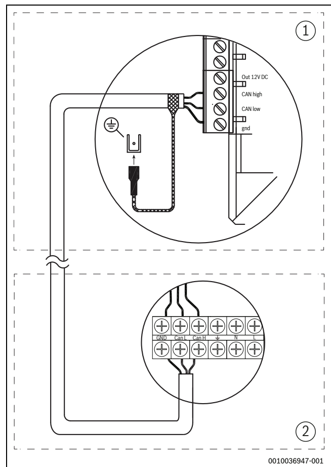
Bild 12 CAN-BUS-Verbindung
