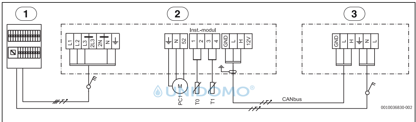
Bild 38 Schaltplan 5,85 kW 3 N~
