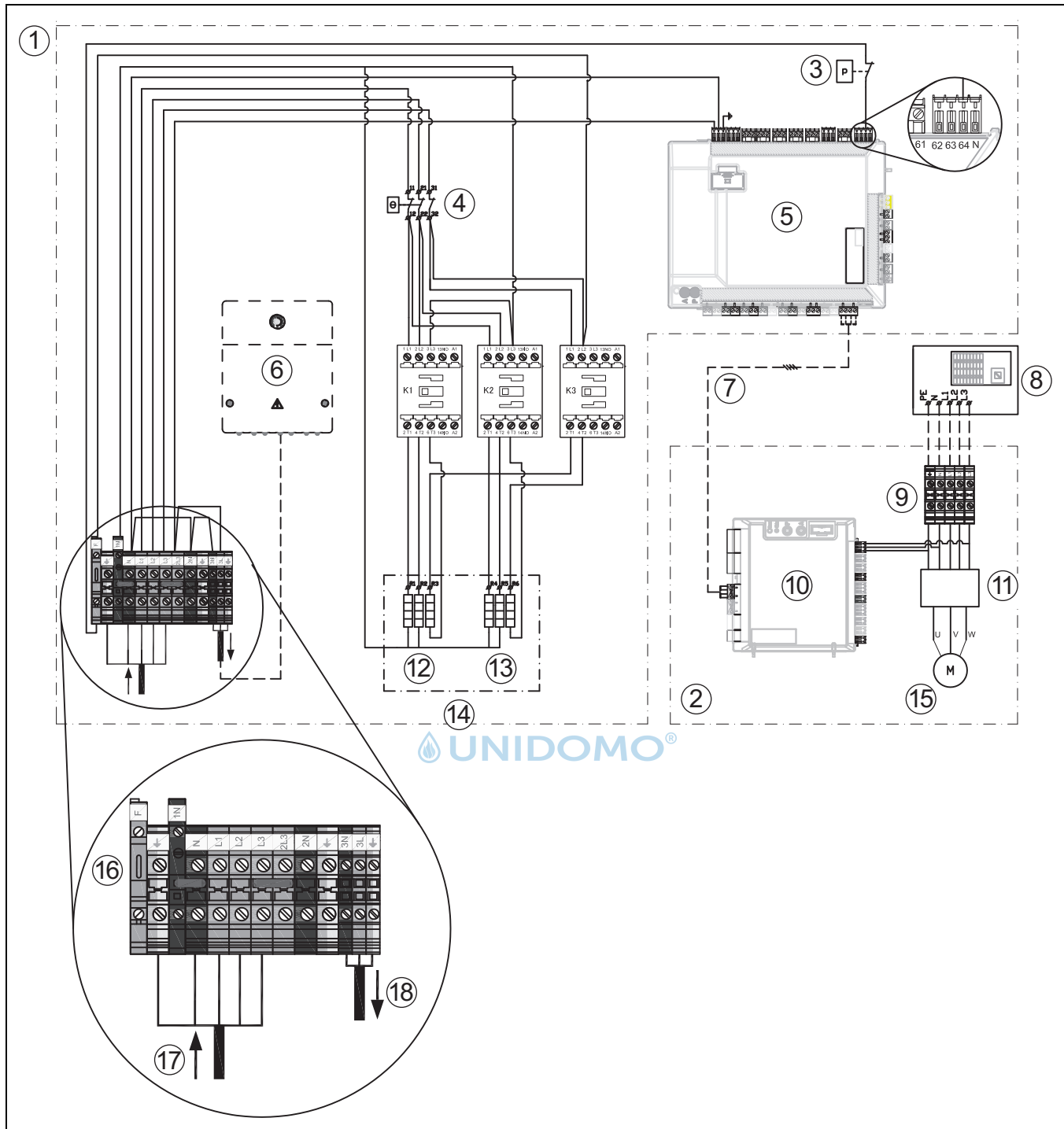
Bild 31 Wärmepumpe (Drehstrom) mit integriertem elektrischen Zuheizer (Drehstrom)
