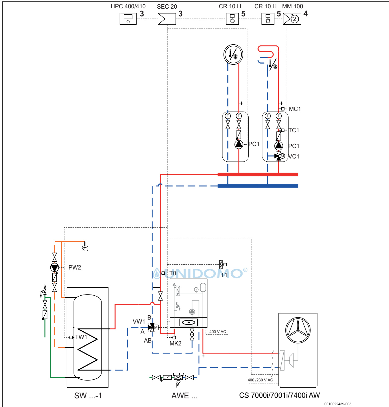
Bild 28 Elektrischer Zuheizter mit Warmwasserbereiter
