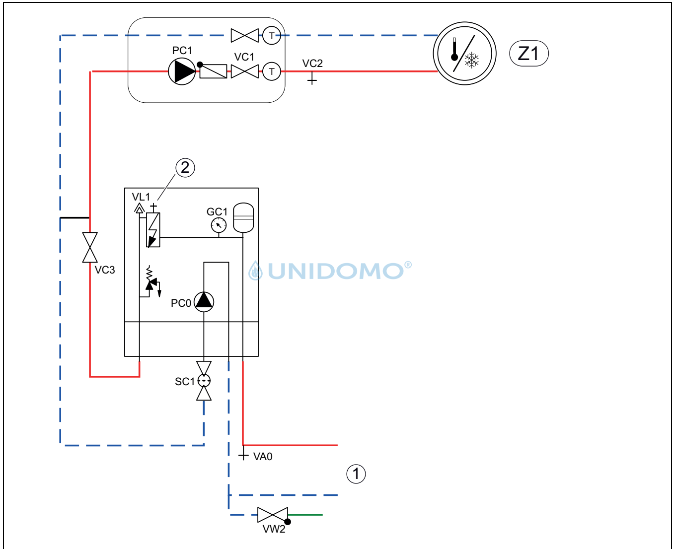
Bild 15 Inneneinheit mit integriertem elektrischen Zuheizler und Heizsystem
