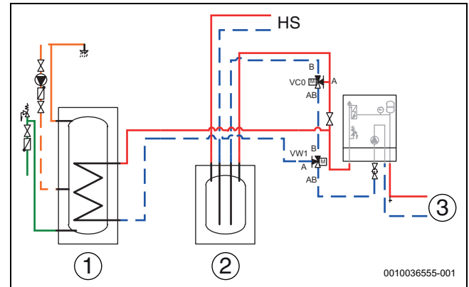
Bild 25 Puffer, VC0-Bypassventil
