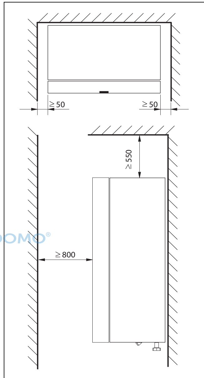
Bild 4 Mindestabstand (mm)
