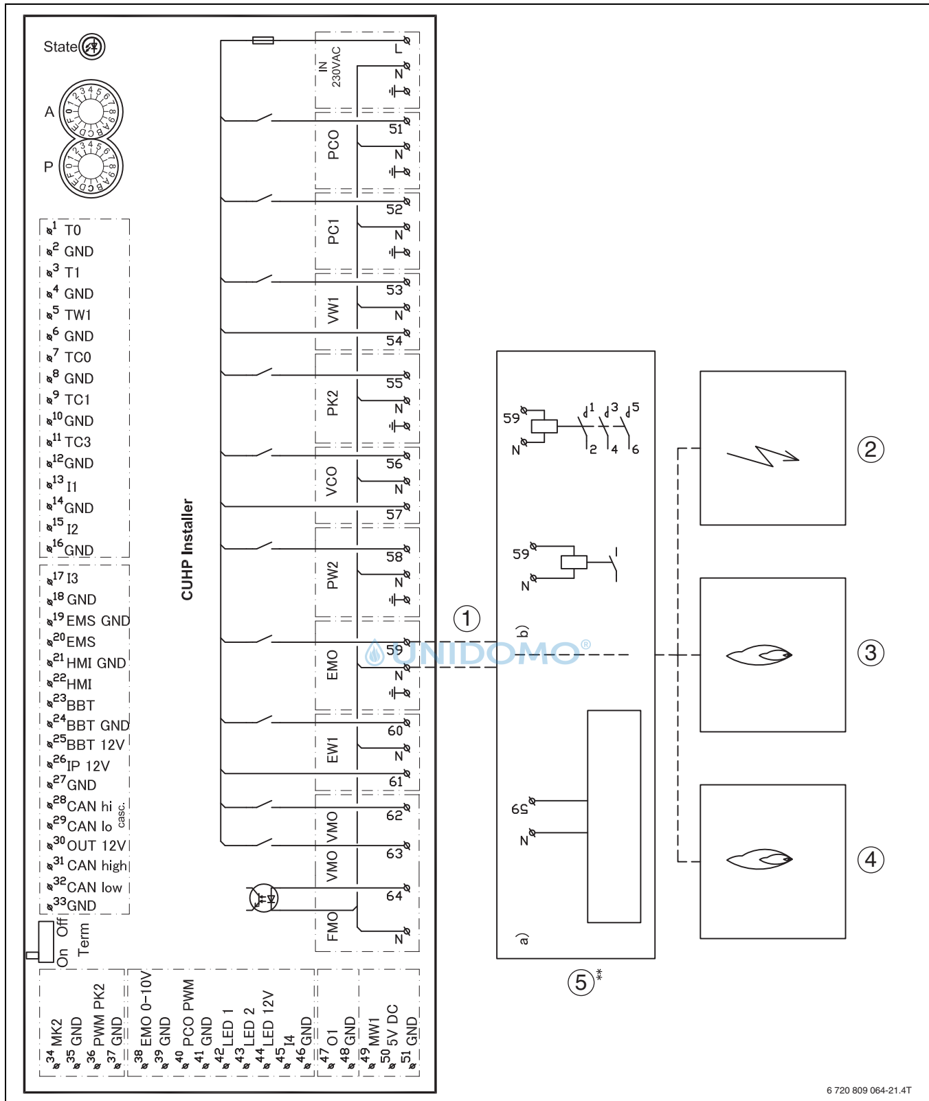
Bild 34 Schaltplan für Installationsmodul, Start/Stop mit externem Zuheiz
