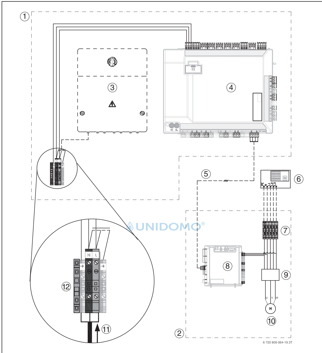
Bild 32 Dreiphasige Wärmepumpe und Inneneinheit mit externem Zuheizler
