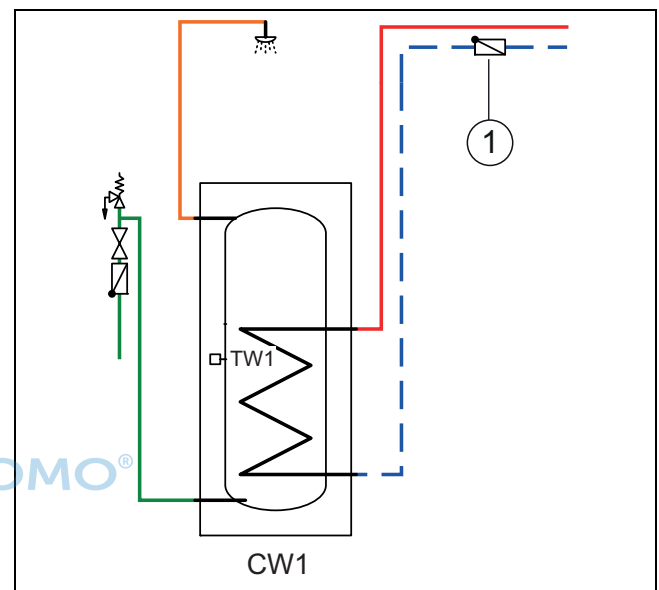
Bild 20 Warmwasserspeicher
