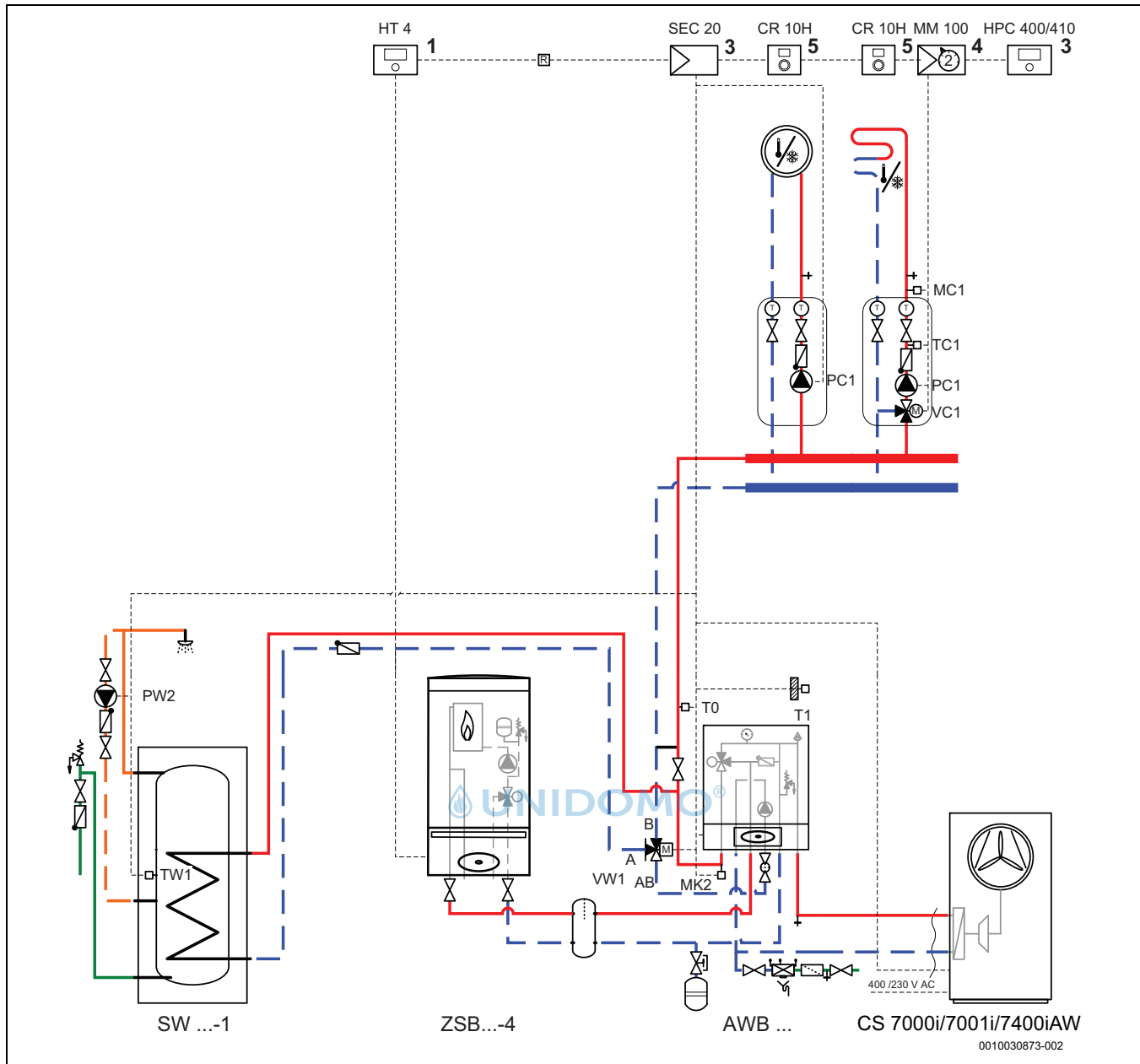
Bild 29 Zuheizer mit Mischer mit Warmwasserspeicher
