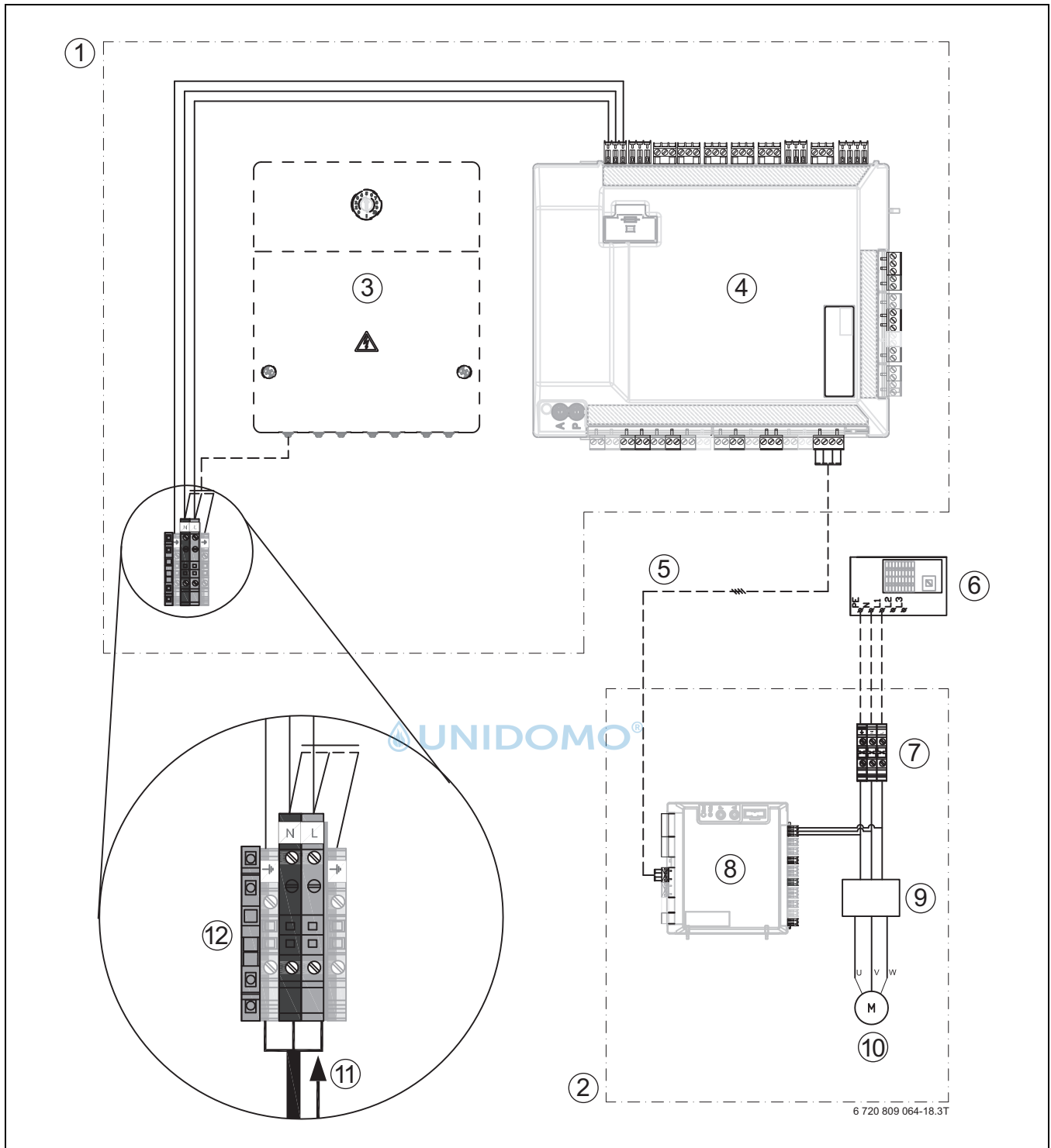
Bild 31 Einphasige Wärmepumpe und Inneneinheit mit externem Zuheizier
