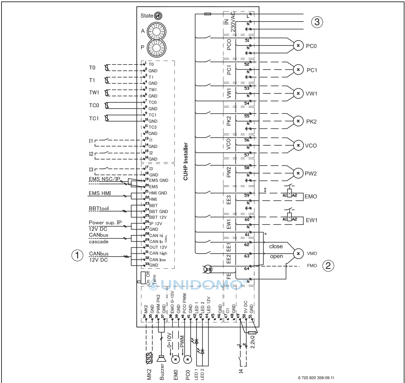
Bild 33 Schaltplan Installationsmodul für Inneneinheit mit Mischer für externen Zuheizier
