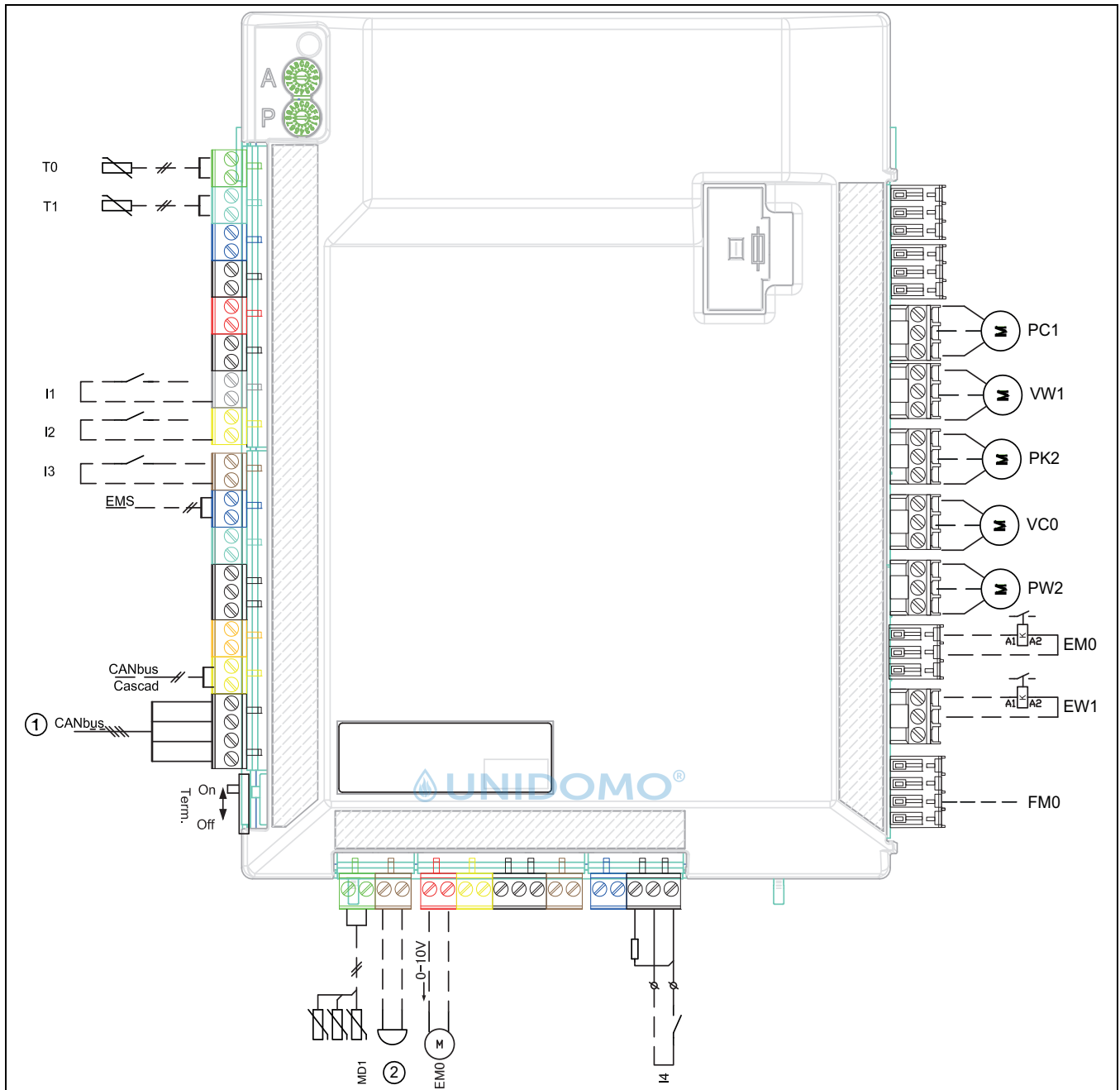
Bild 13 Anschlüsse Installationsmodul
