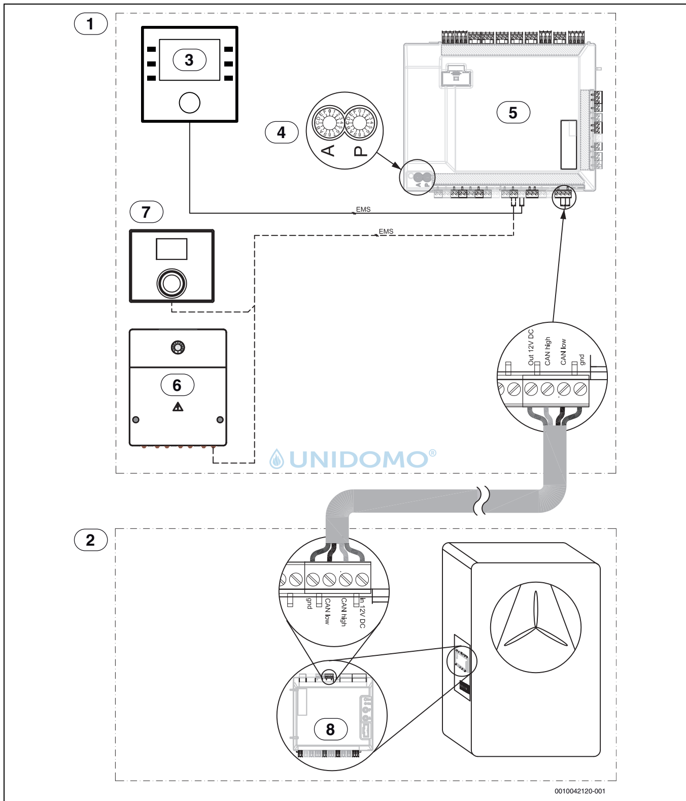
Bild 30 Inneneinheit mit Mischer für externen Zuheizier – Überblick CAN-/EMS-BUS
