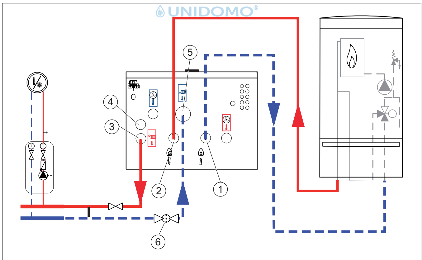
Bild 8 Anschluss der Inneneinheit mit Mischer für externen Zuheizier an die Heizungsanlage und den Zuheizier
