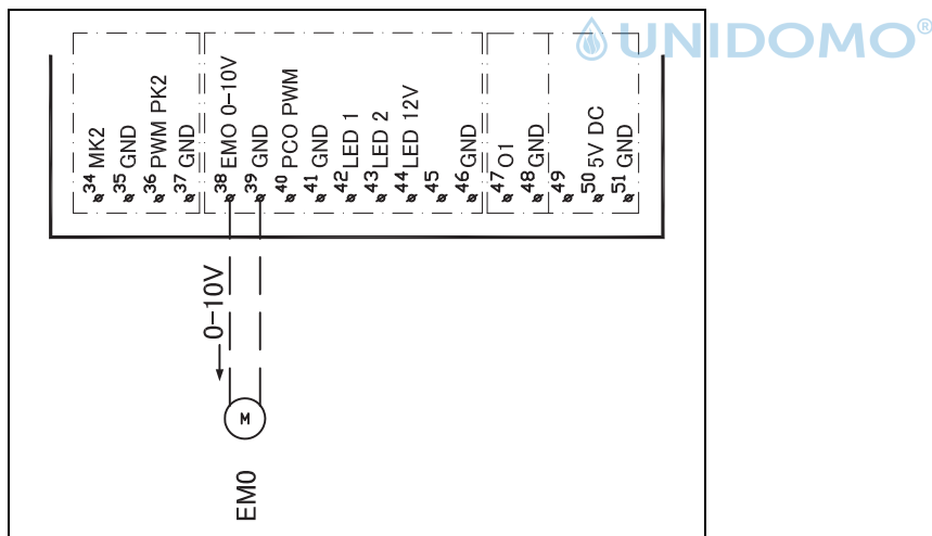
Bild 14 0- bis 10-V-Ansteuerung für externe Zuheizers
