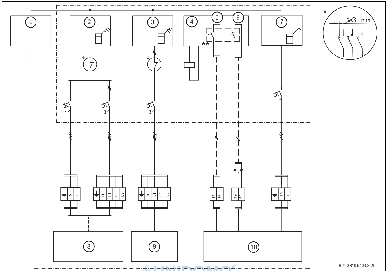
Bild 33 EVU Typ 1
