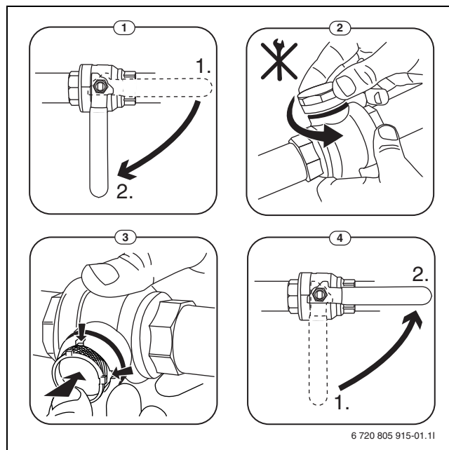
Bild 19 Siebreinigung
