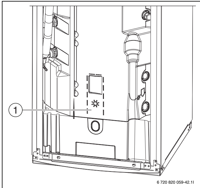
Bild 21 Anordnung von Temperaturfühler TW1 und ggf. TS2
