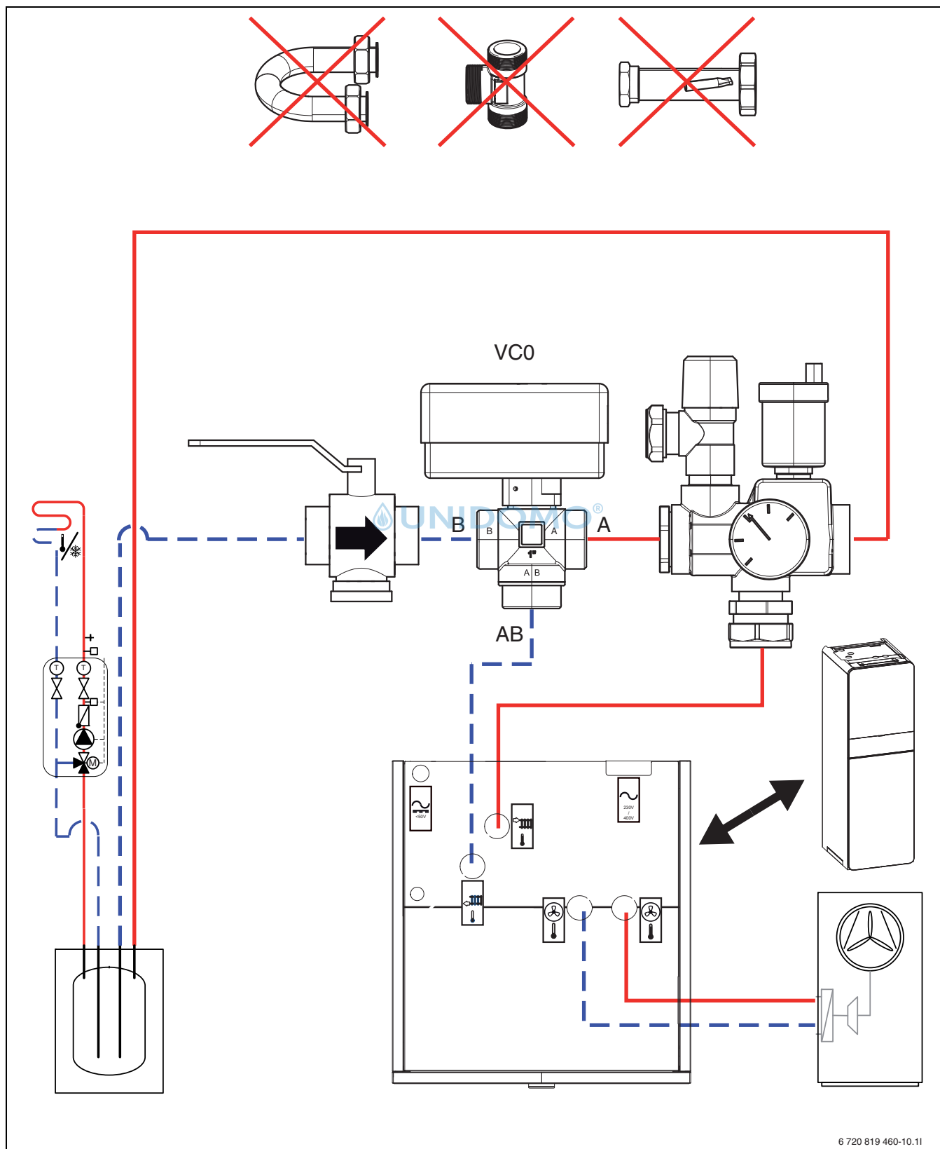
Bild 23 Installation mit Pufferspeicher
