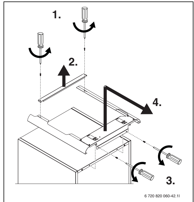
Bild 8 Abdeckung an der Oberseite abnehmen
