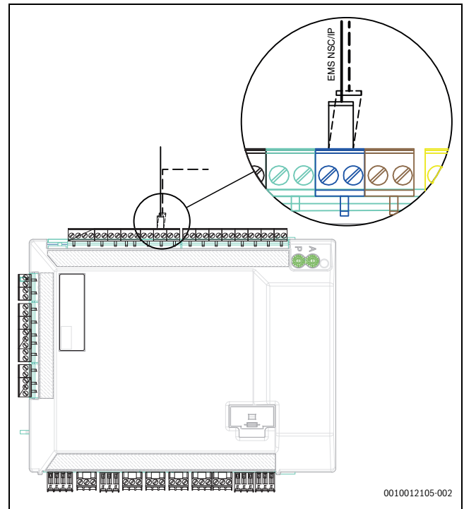
Bild 20 EMS-Anschluss am Installationsmodul
