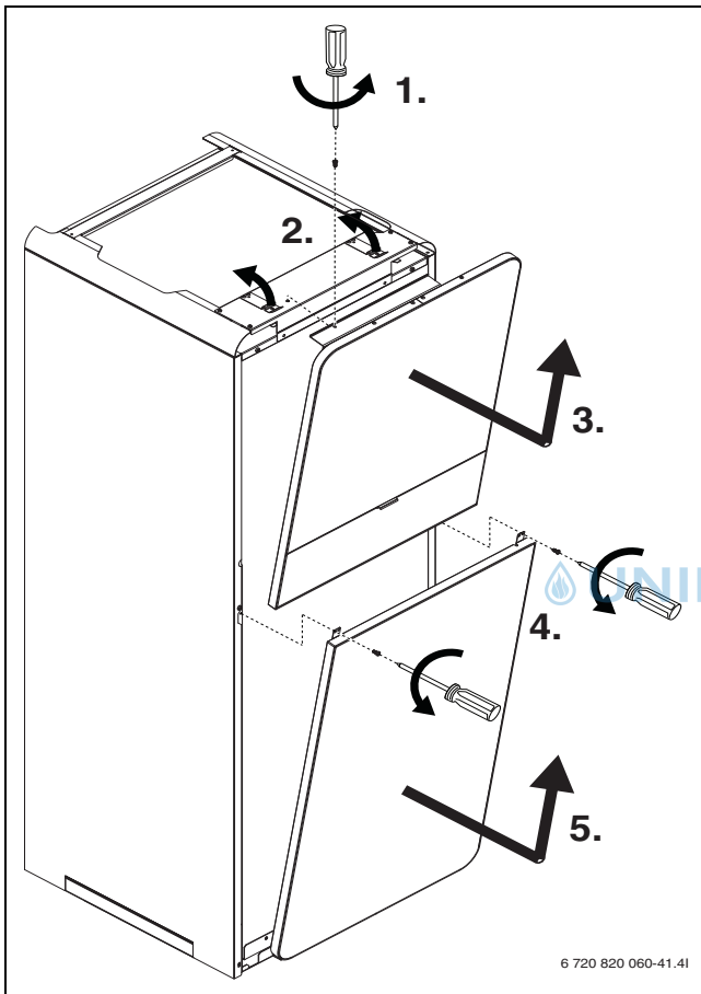
Bild 7 Frontplatten abnehmen
