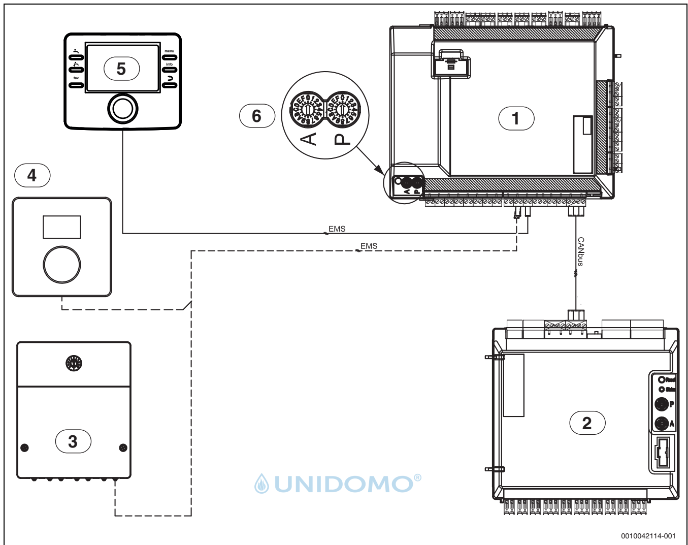
Bild 29 CAN-BUS und EMS – Überblick
