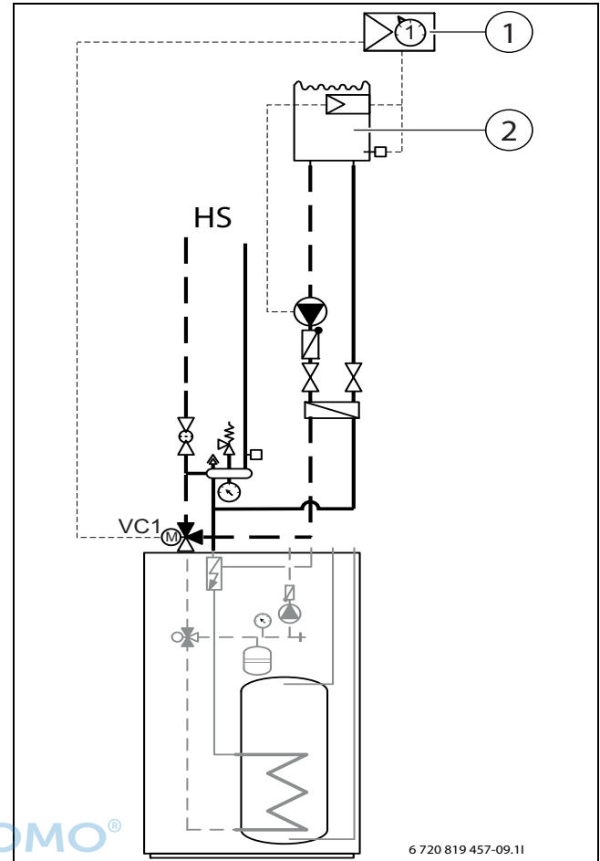
Bild 22 Beispieldarstellung für Pool-Installation
