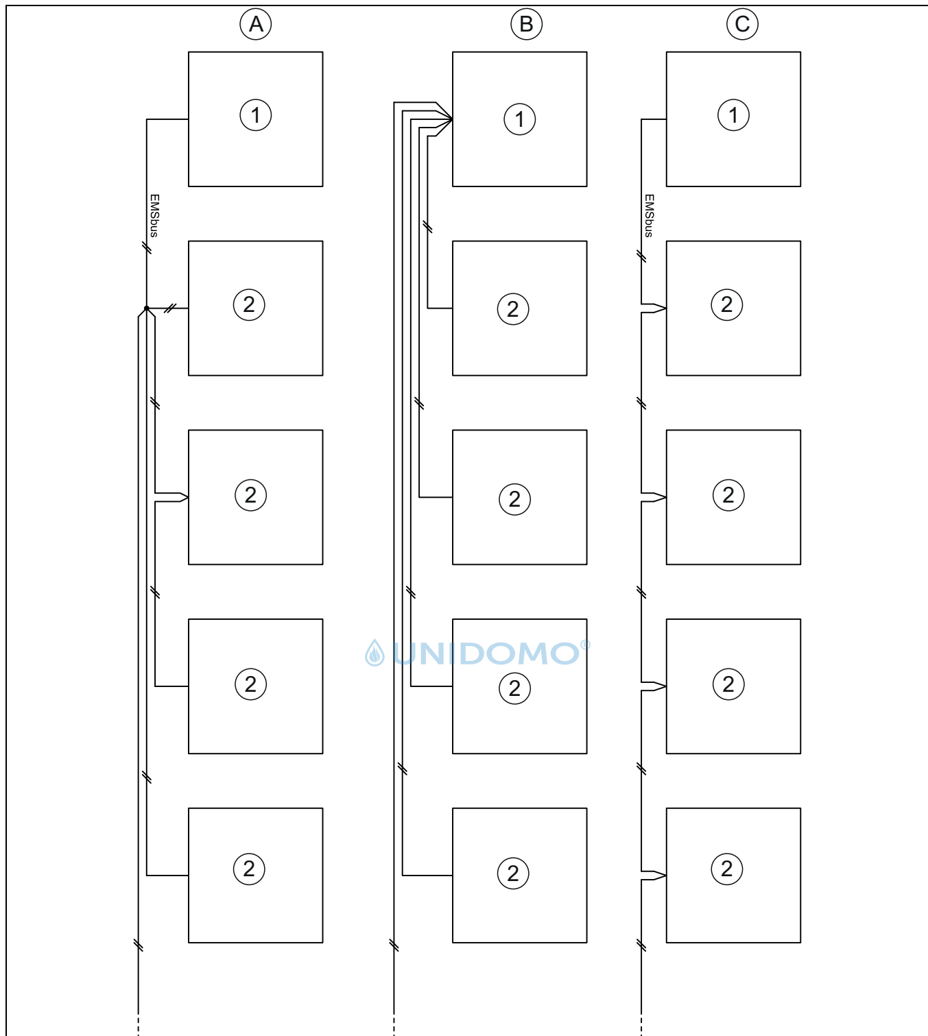
Bild 30 Anschlussalternativen für EMS-Bus
