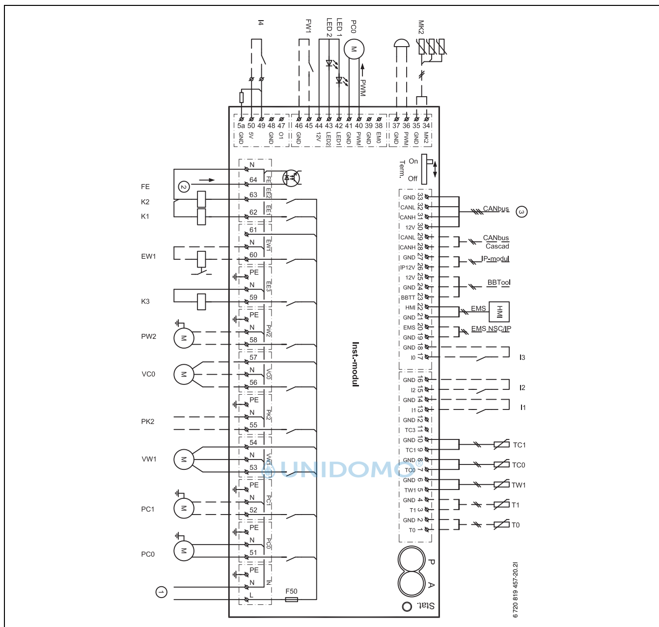
Bild 28 Schaltplan, Installationsmodul
