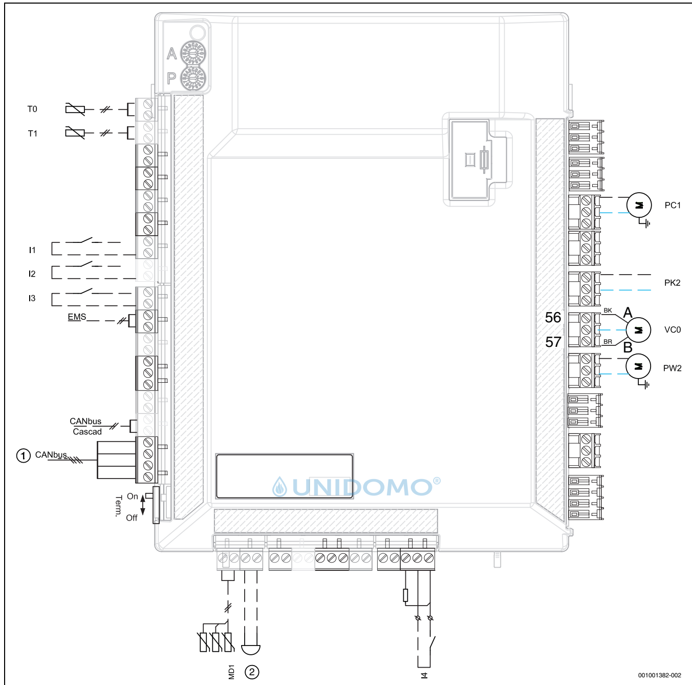
Bild 16 Anschlüsse Installationsmodul
