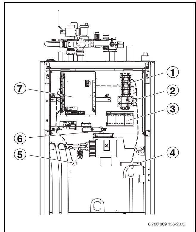
Bild 15 Komponentenanzordnung im Schaltkasten und Kabelkanäle
