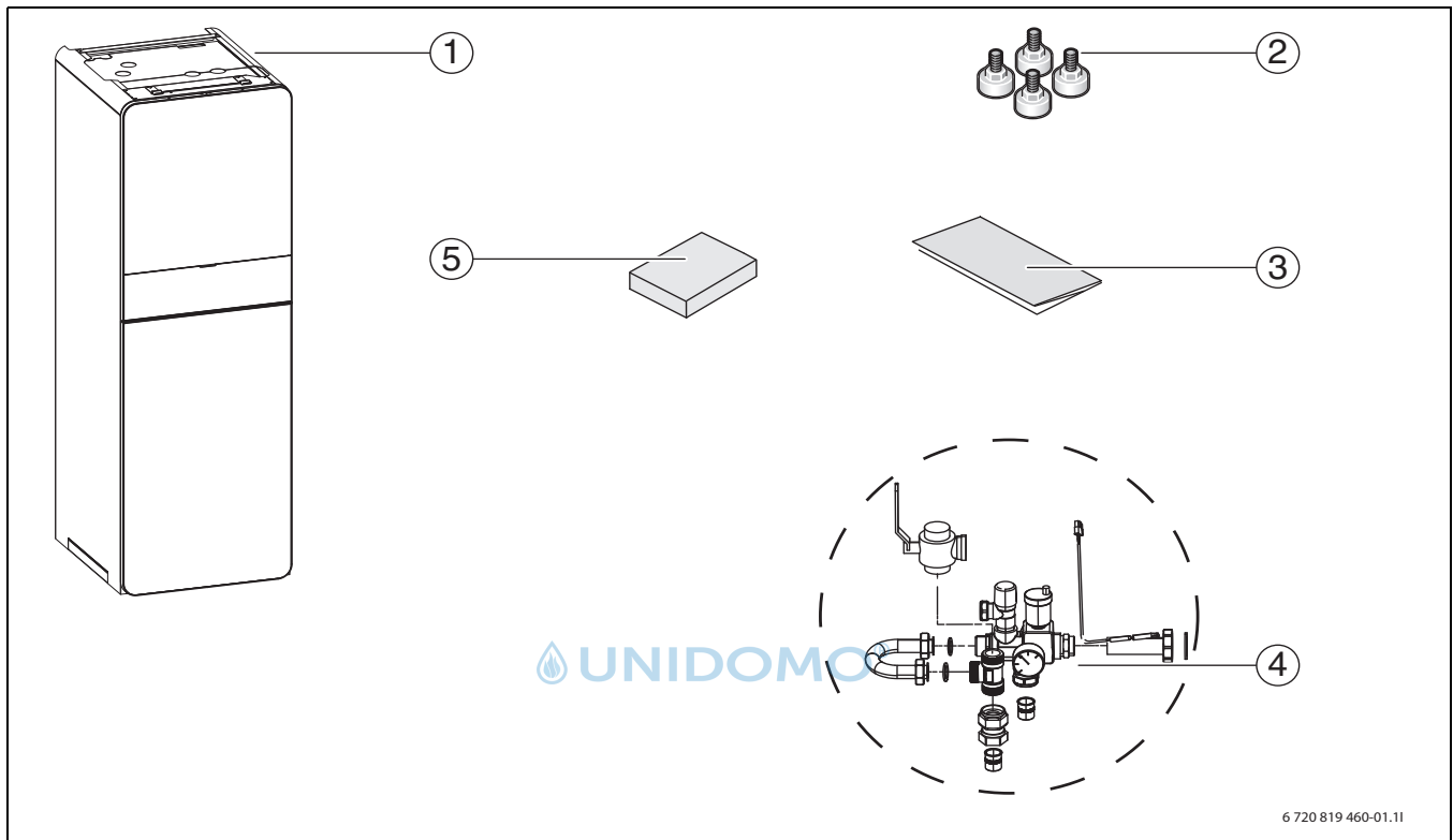
Bild 2 Lieferumfang
