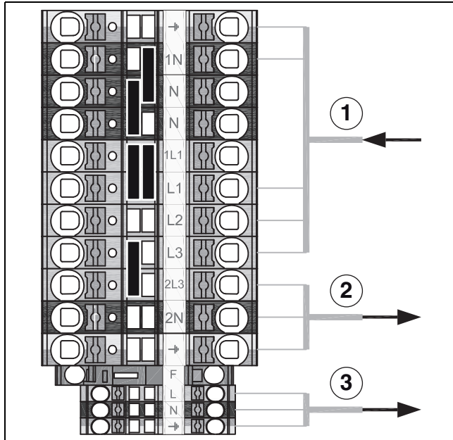
Bild 17 Standardausführung
