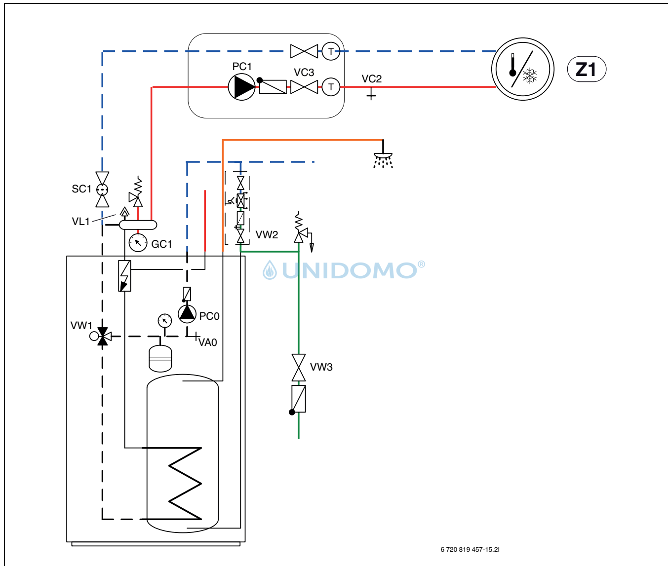
Bild 18 Inneneinheit und Heizungsanlage
