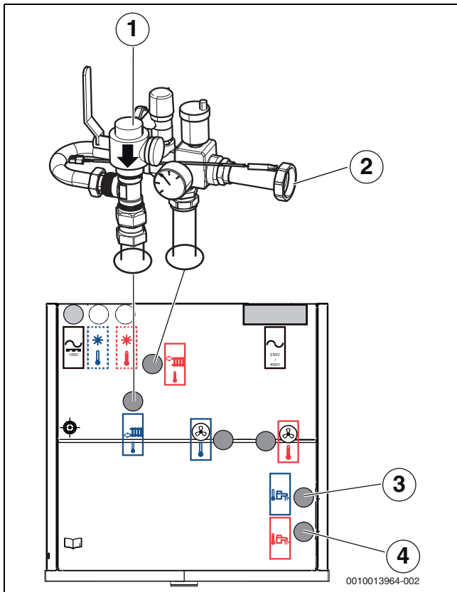
Bild 10 Anschlüsse der Inneneinheit für die Heizungsanlage und Warmwasser
