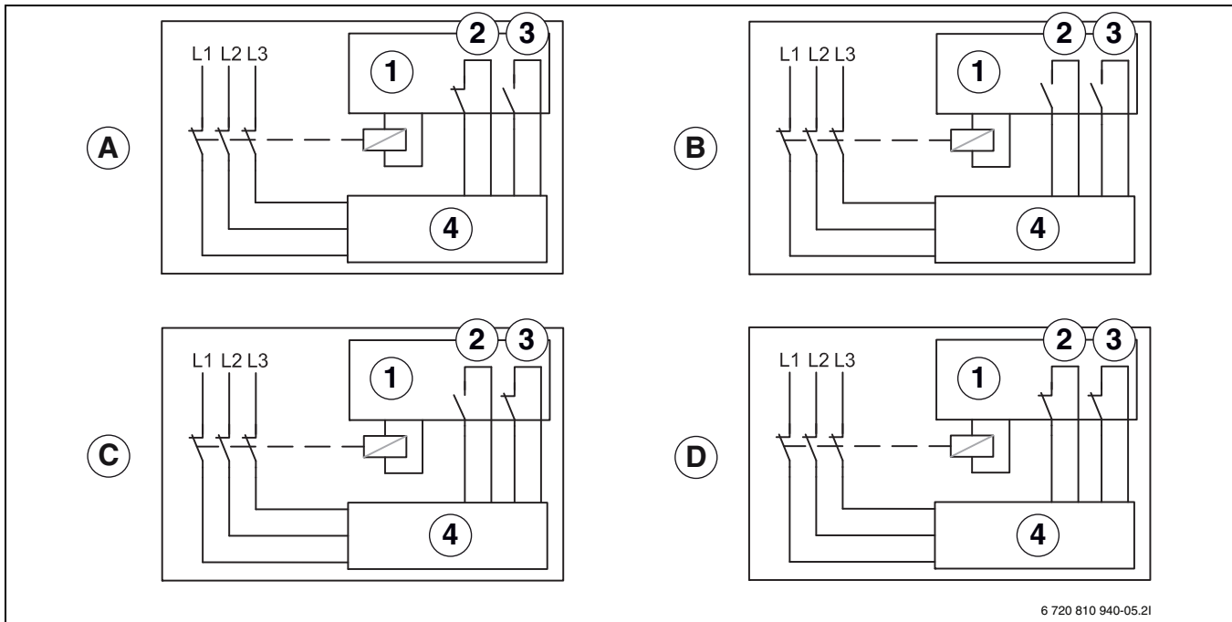
Bild 32 Anschlussplan für EVU/SG
