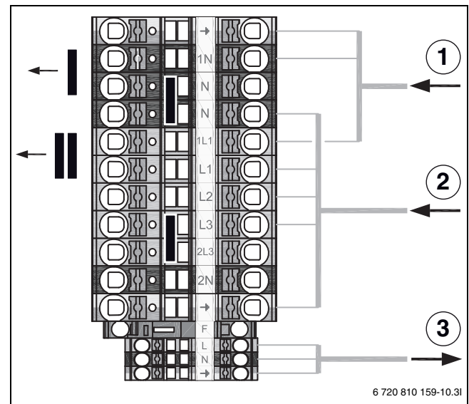
Bild 31 Klemmenanschlüsse und Anordnung der Brücken
