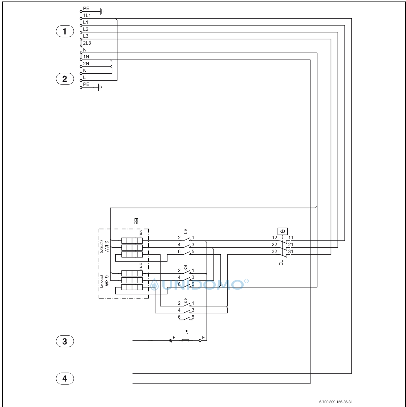
Bild 27 Stromversorgung Inneneinheit und Wärmepumpe
