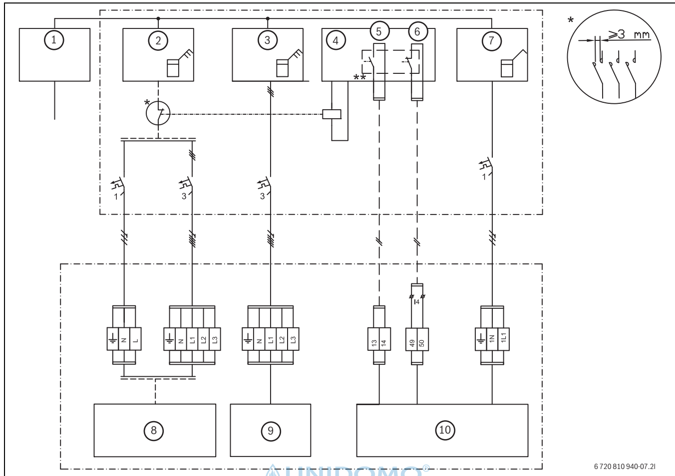
Bild 34 EVU Typ 2
