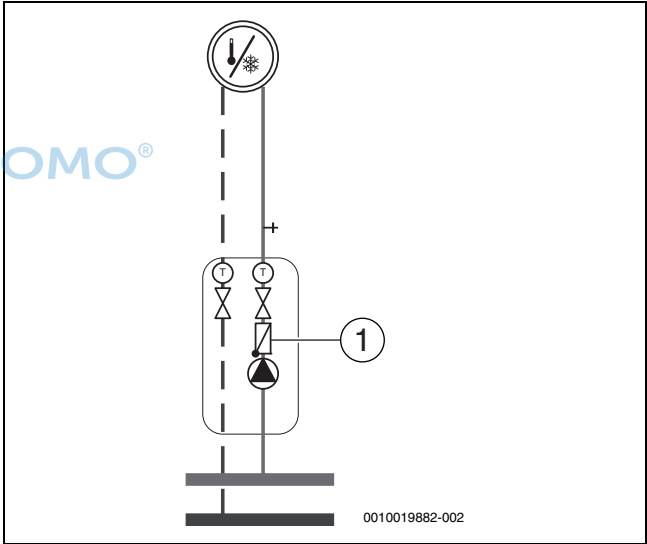
Bild 24 Heizkreis
