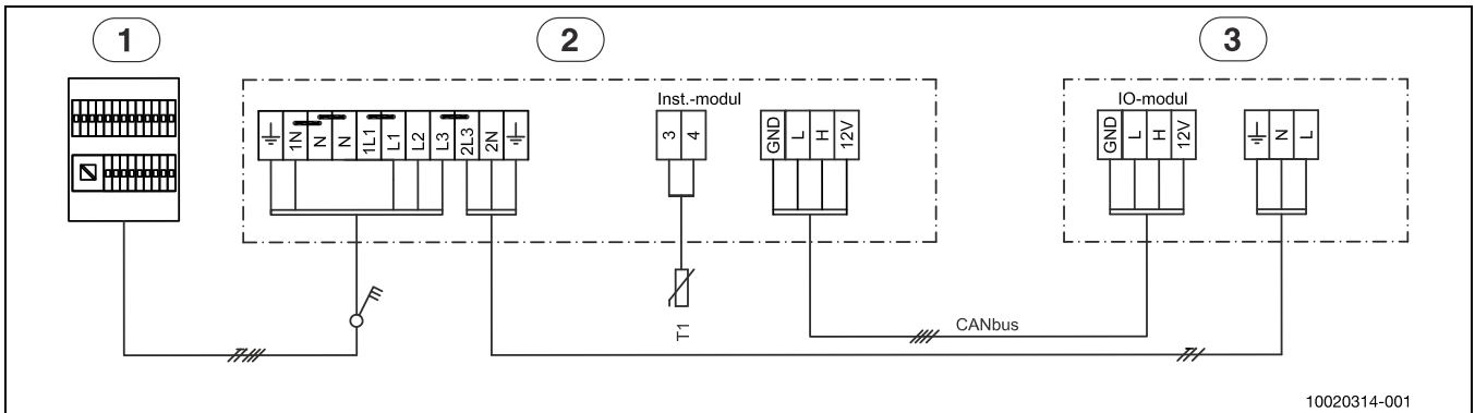
Bild 45 Schaltplan 3N~
