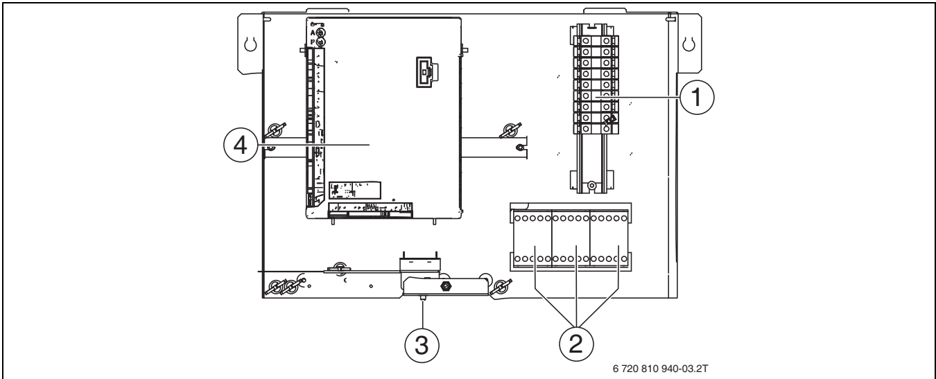
Bild 19 Klemmenkastenordnung
