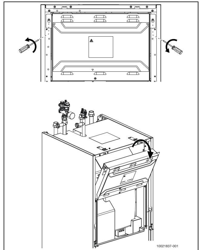
Bild 24 Klemmenkasten
