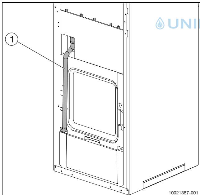
Bild 13 Rückansicht Ablaufschlauch
