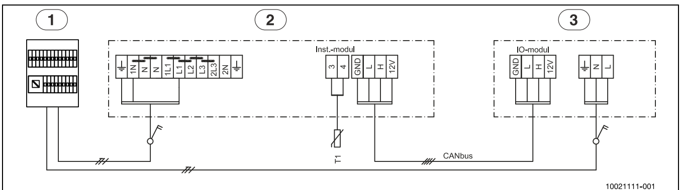
Bild 47 Schaltplan 1N~ 1)
