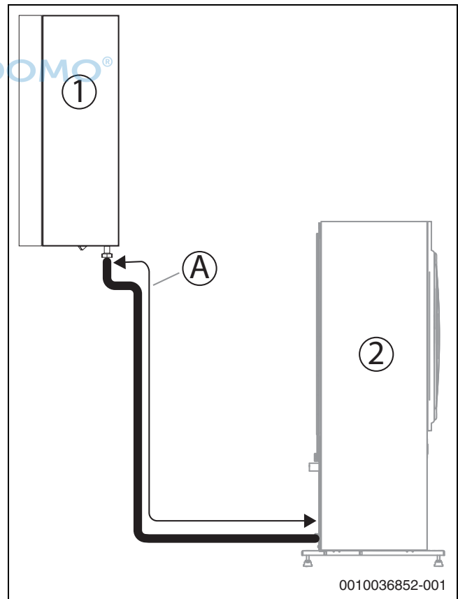
Bild 13 Rohrlänge A
