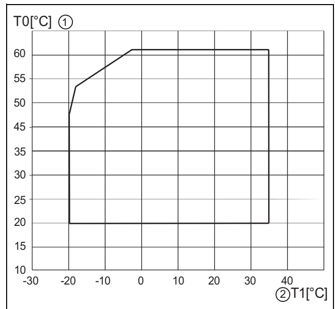
Bild 20 Wärmepumpe ohne Zuheizler
