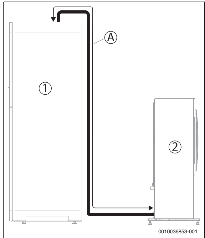
Bild 12 Rohrlänge A
