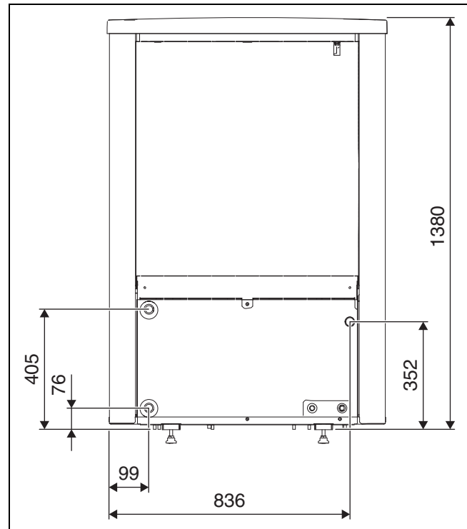
Bild 4 Abmessungen und Anschlüsse der Wärmepumpenmodelle 5 OR-7 OR, Rückseite
