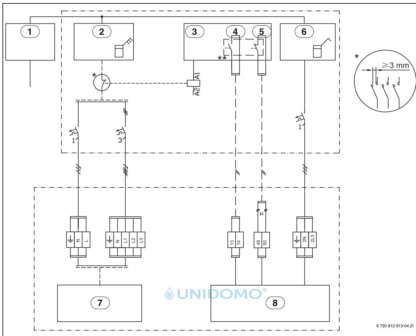
Bild 38 EVU 2, nur Abschaltung des Kompressors
