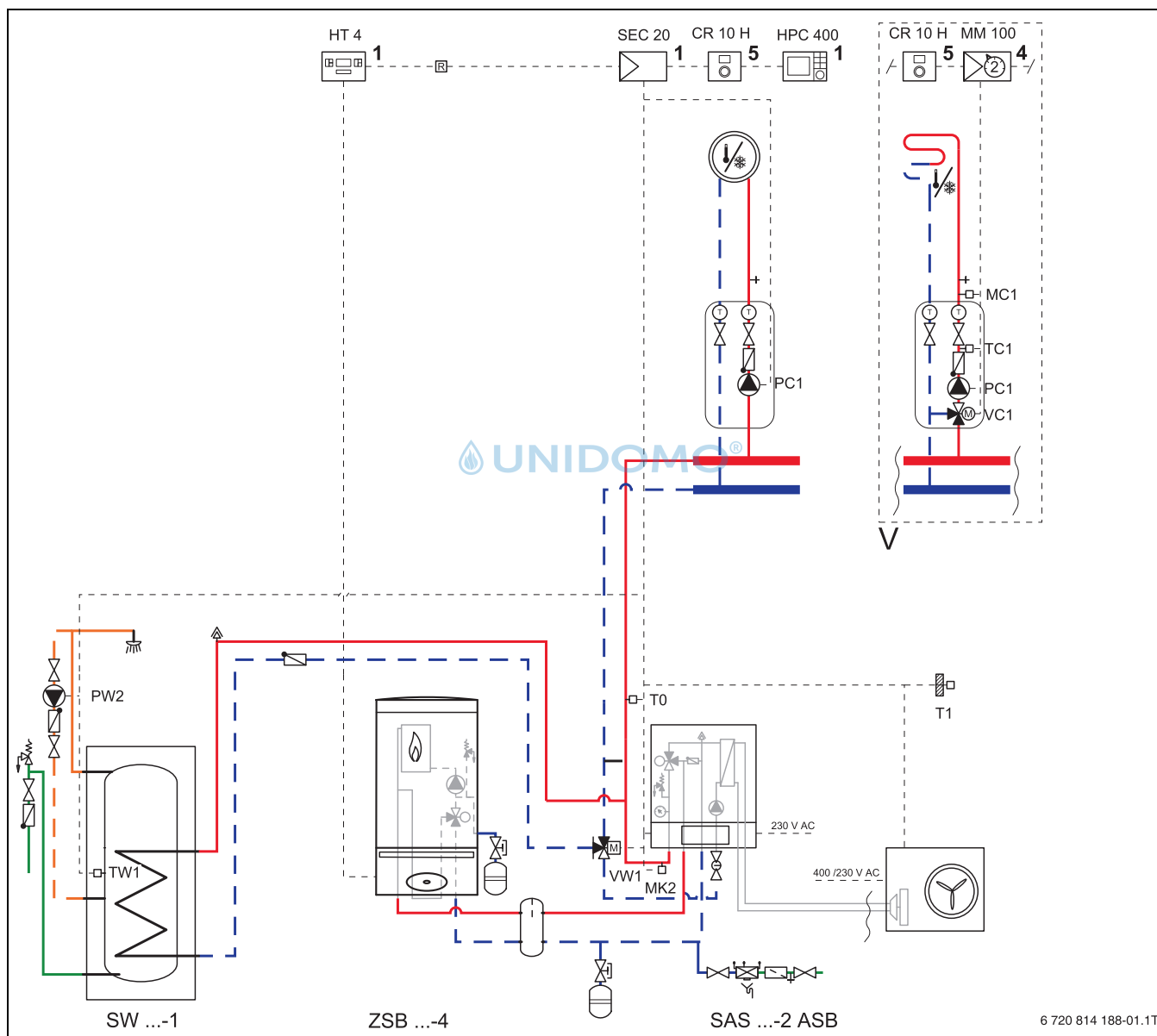
Bild 31 Anlagenkonfiguration mit Wärmepumpe und Inneneinheit mit Mischer für externen Zuheizter
