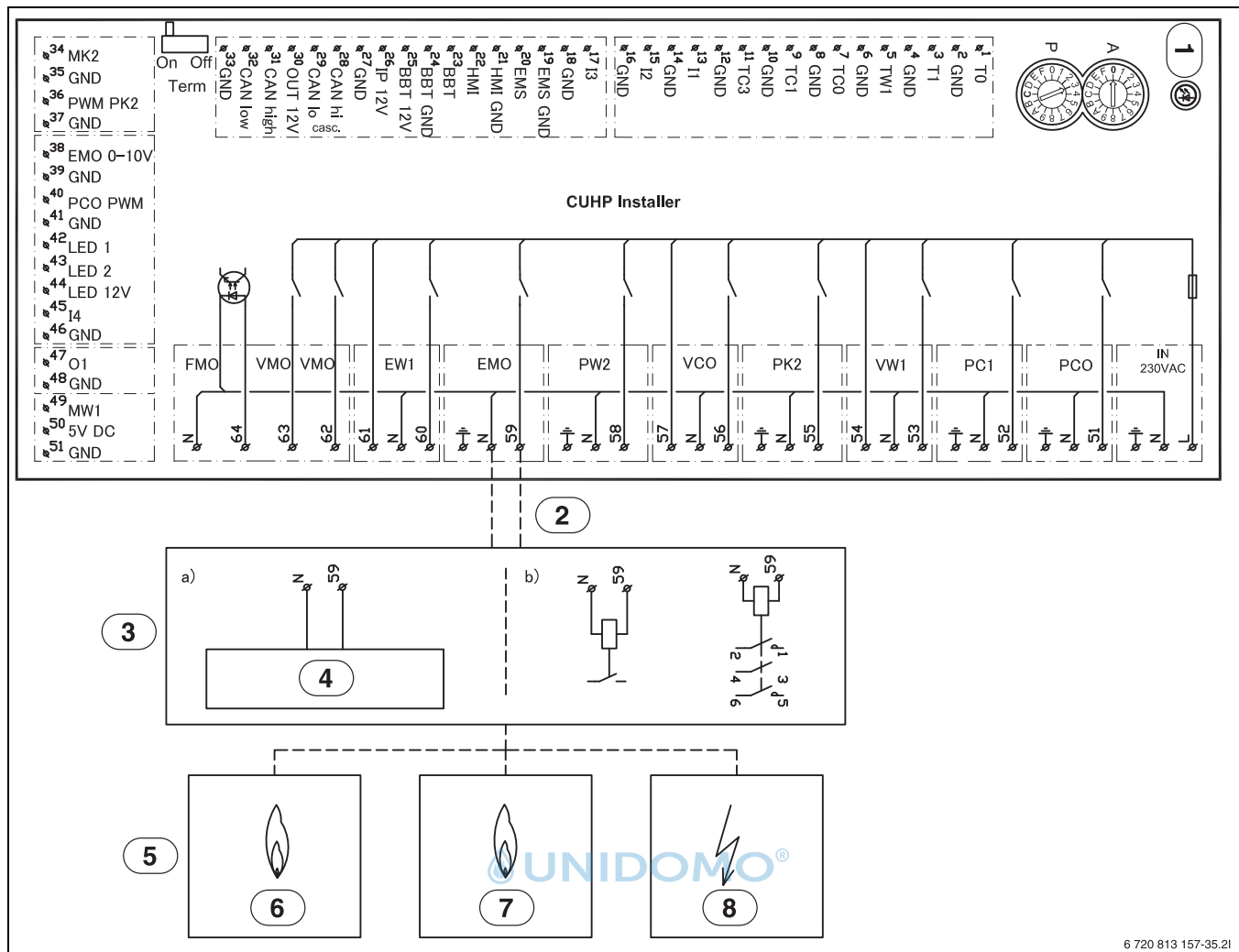
Bild 13 Schaltschema des Installationsmoduls ein-/ausschalten
