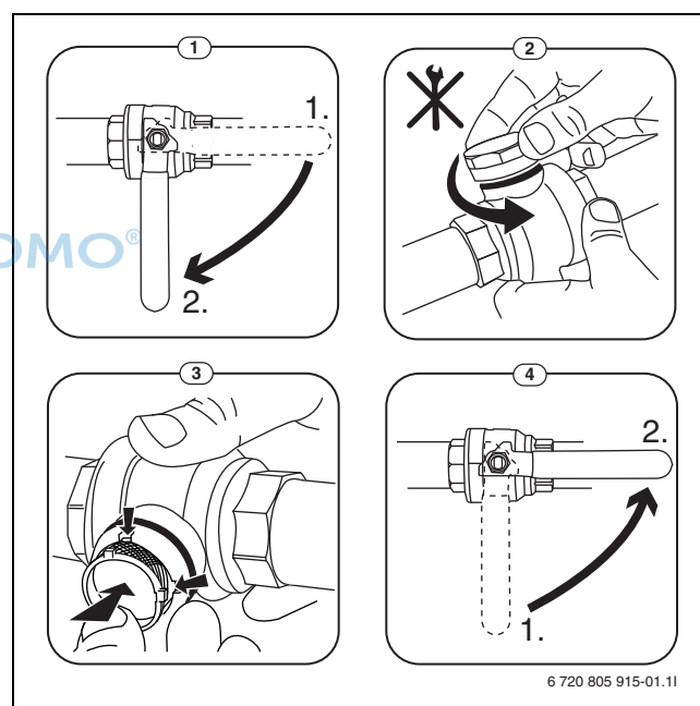
Bild 18 Siebreinigung
