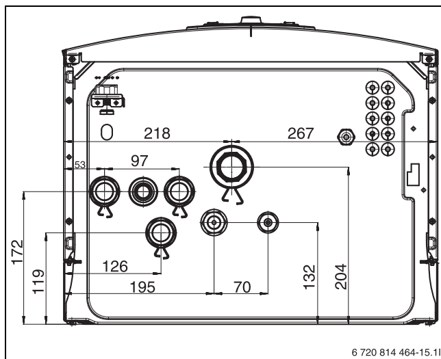
Bild 4 Abmessungen und Anschlüsse
