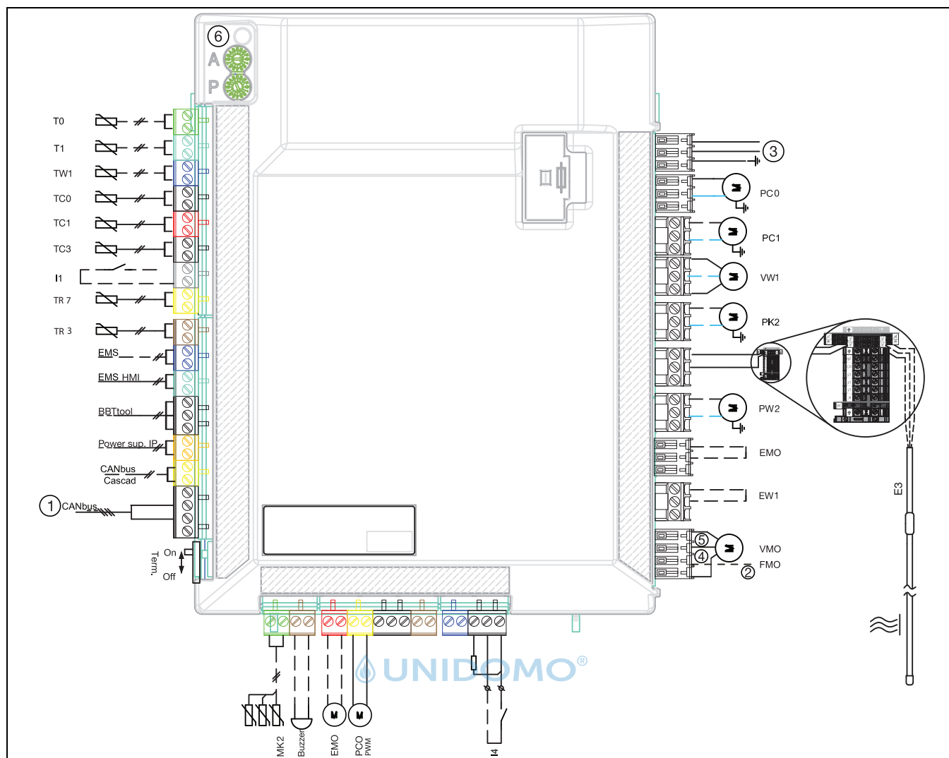
Bild 12 Schaltschema des Installationsmoduls für Inneneinheit mit Mischer
