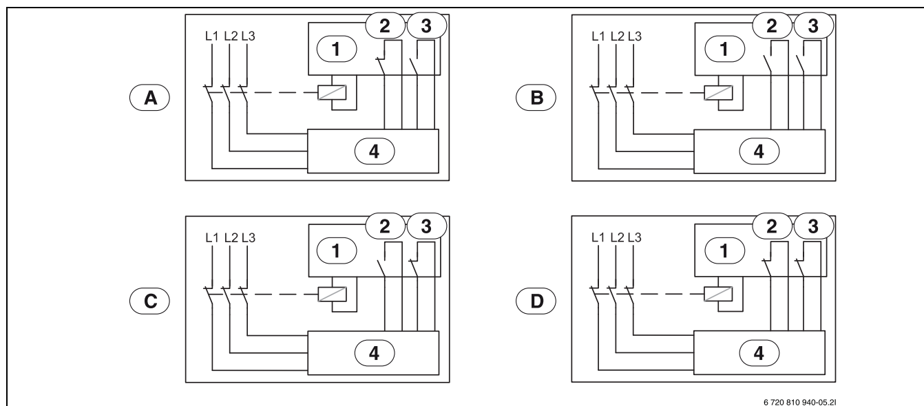
Bild 37 Anschlussplan für EVU/SG
