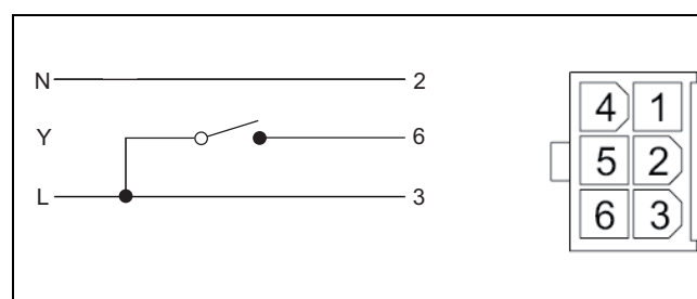
Bild 25 Molex-Stecker
