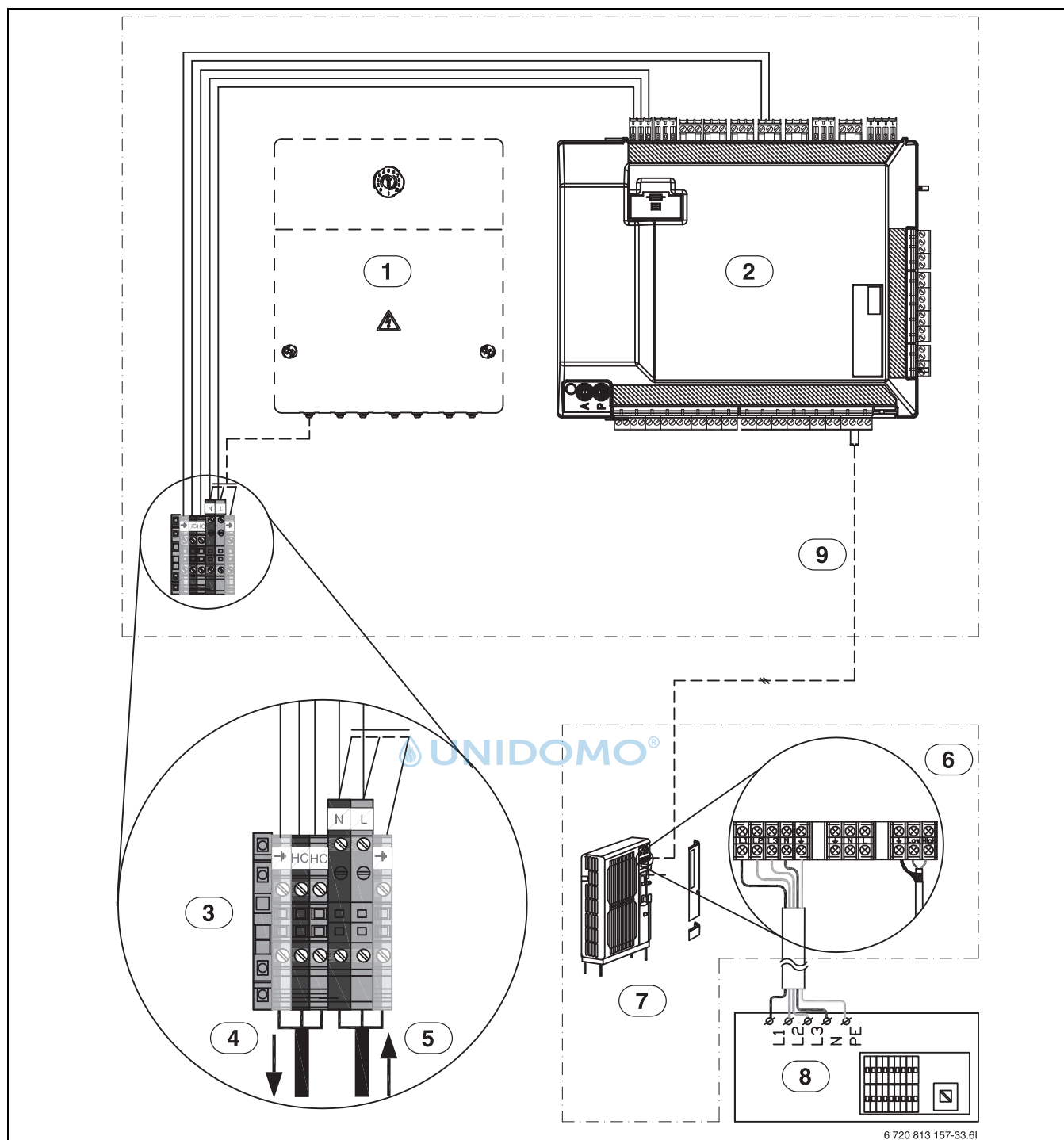
Bild 35 Inneneinheit mit 400V~ 3N Außeneinheit
