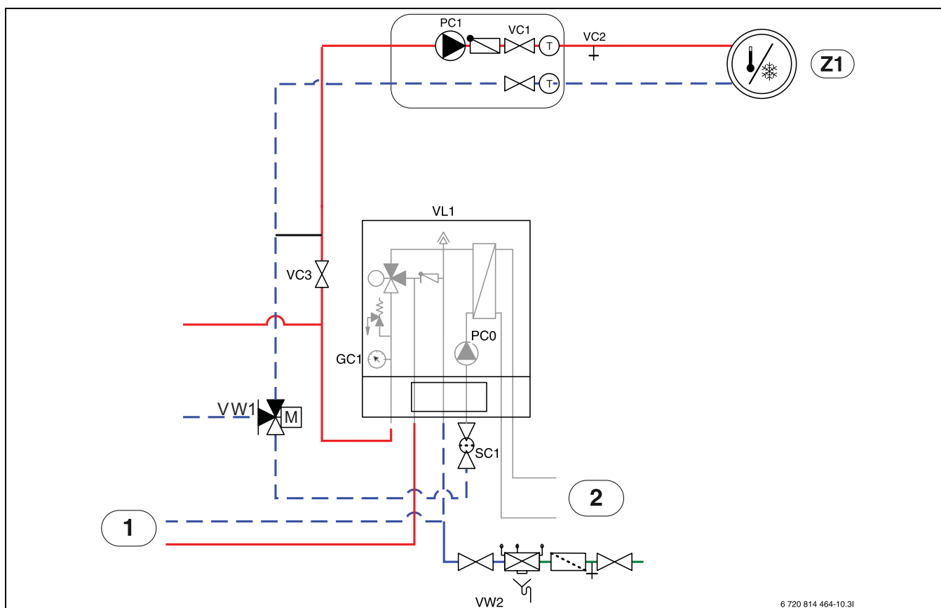
Bild 8 Inneneinheit mit externem Zuheizer und Heizsystem
