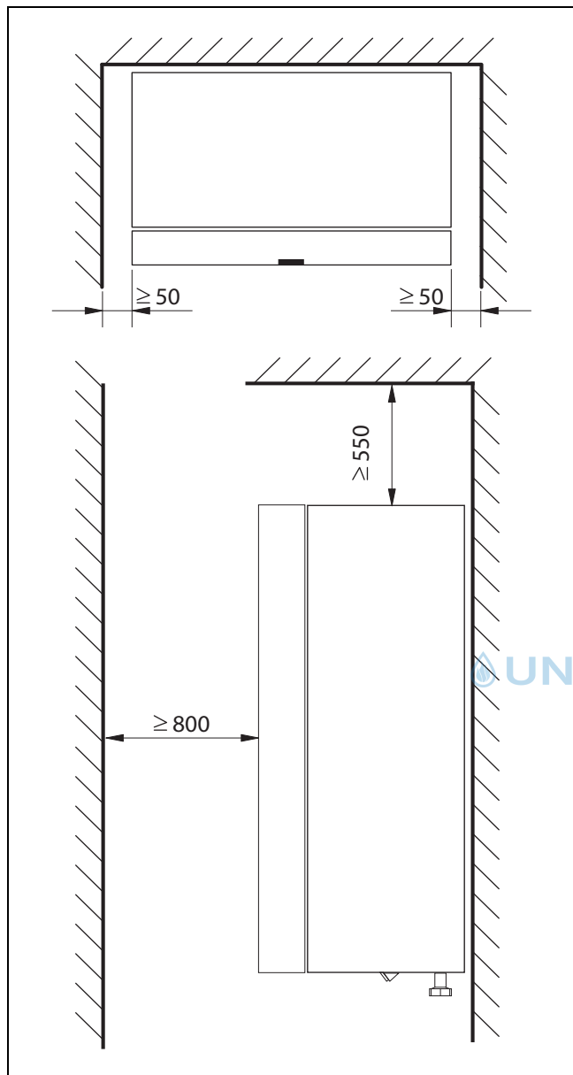
Bild 3 Mindestabstand (mm)
