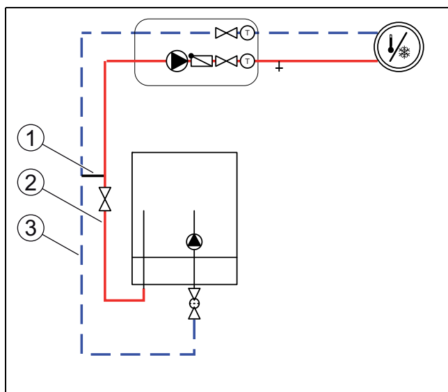
Bild 27 Inneneinheit mit Heizkreis und Bypass
