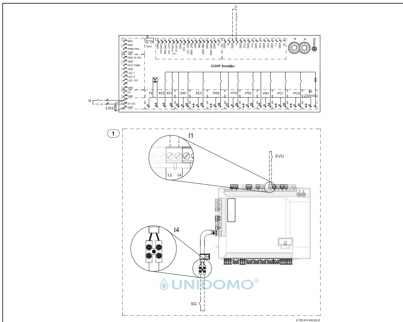
Bild 36 Externer Eingang EVU/SG
