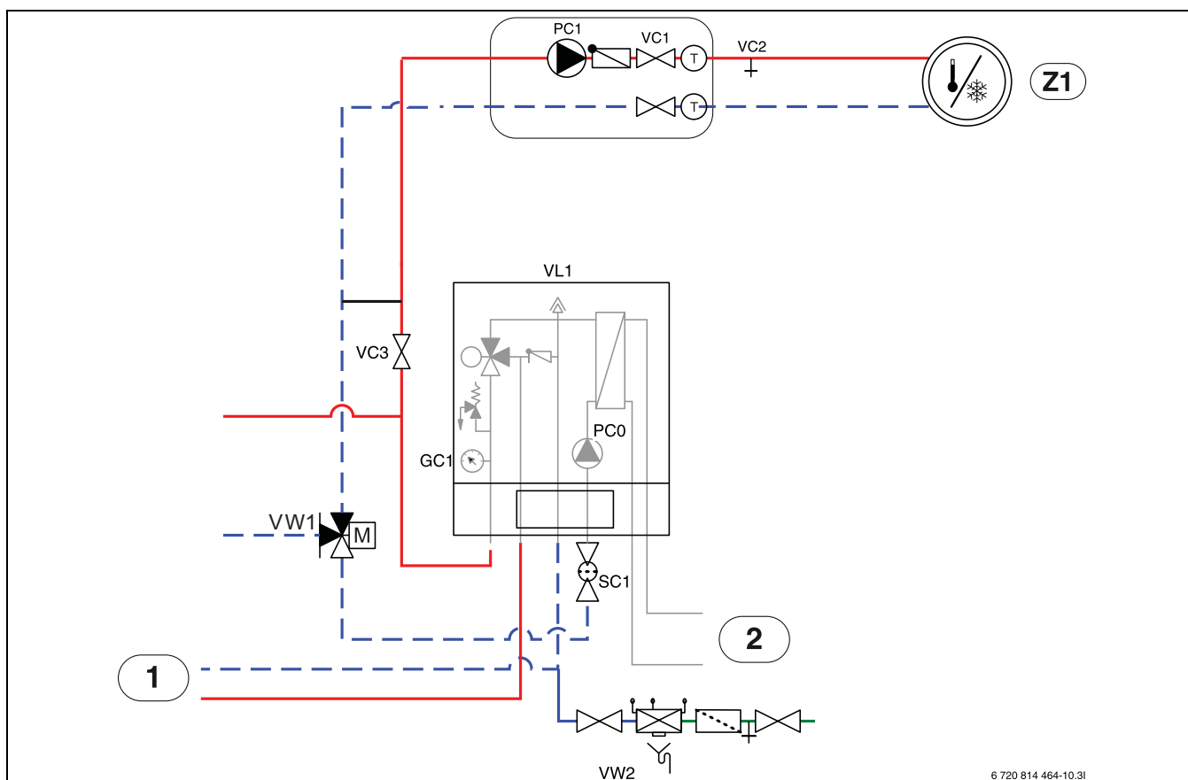
Bild 17 Inneneinheit mit externem Zuheizter und Heizsystem
