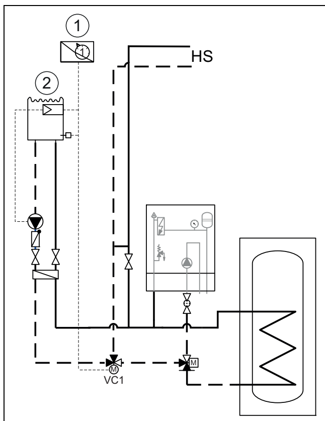
Bild 26 Beispieldarstellung für Pool-Installation
