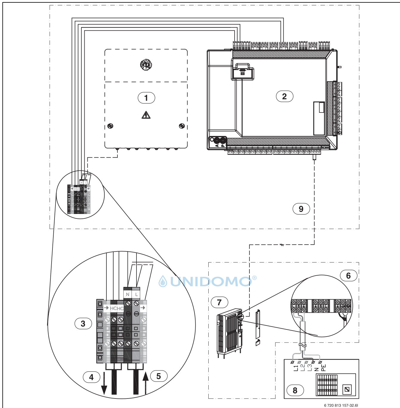
Bild 34 Inneneinheit mit 230V~ 1N Außeneinheit
