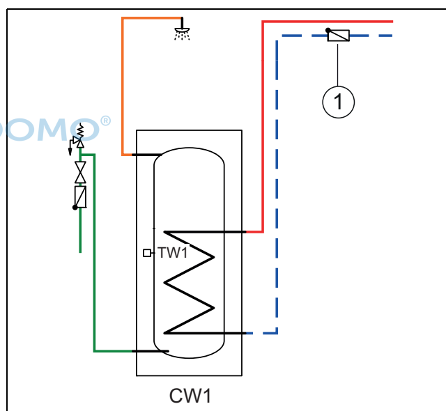
Bild 20 Warmwasserspeicher
