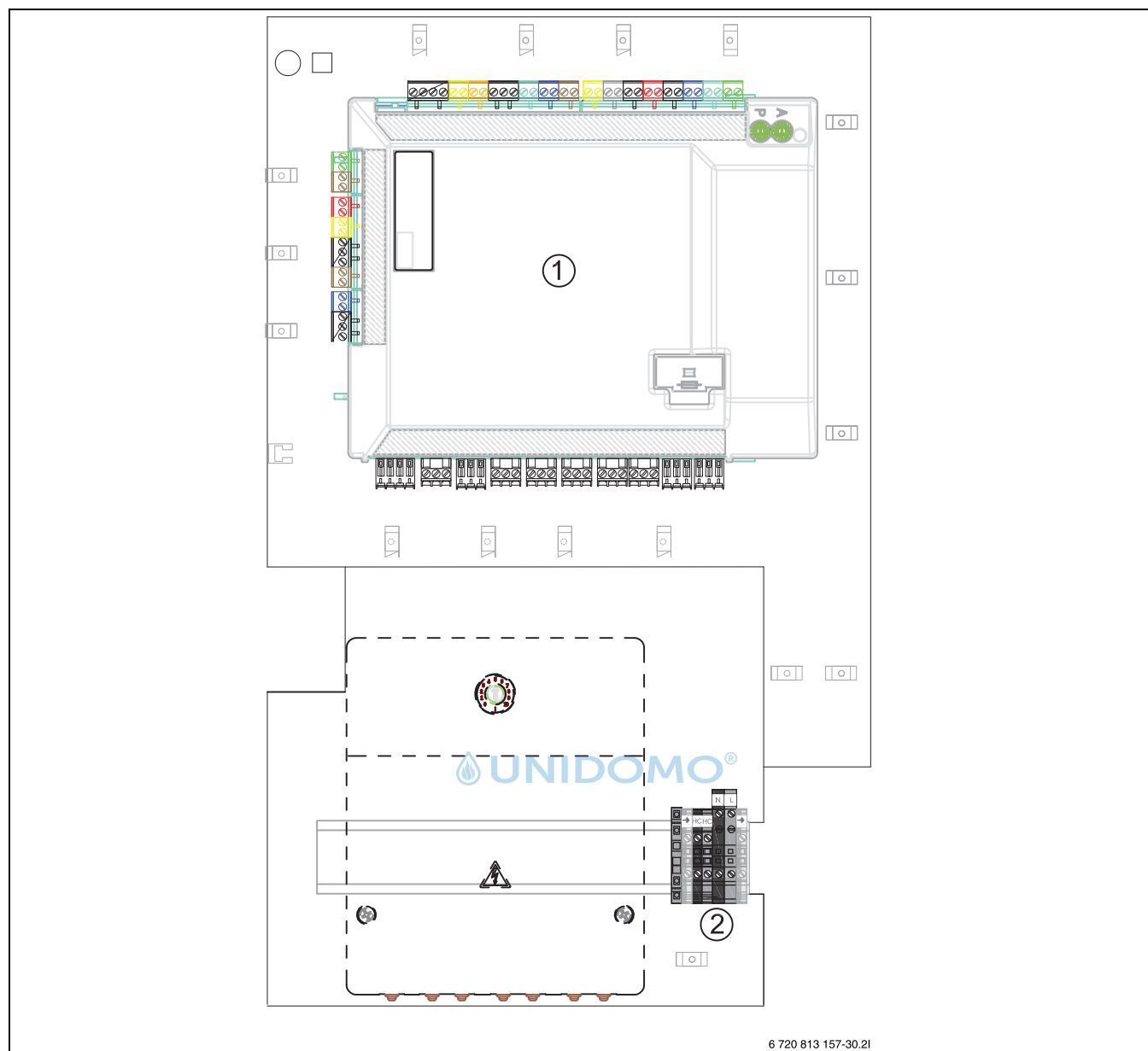
Bild 32 Überblick elektrische Anschlüsse in der Inneneinheit mit Mischventil
