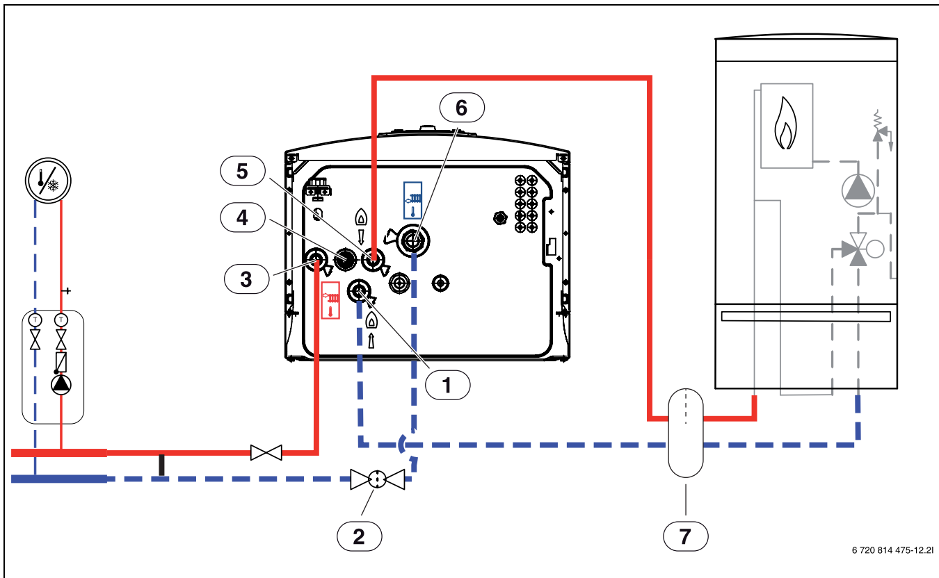
Bild 7 Anschluss der Inneneinheit mit Mischer für externen Zuheizer an die Heizungsanlage und den Zuheizer
