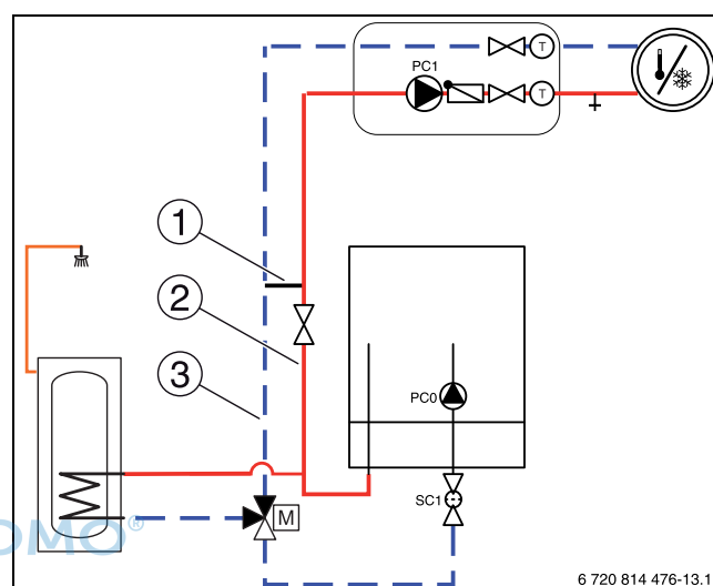
Bild 28 Inneneinheit mit Heizkreis und Warmwasserbereitung
