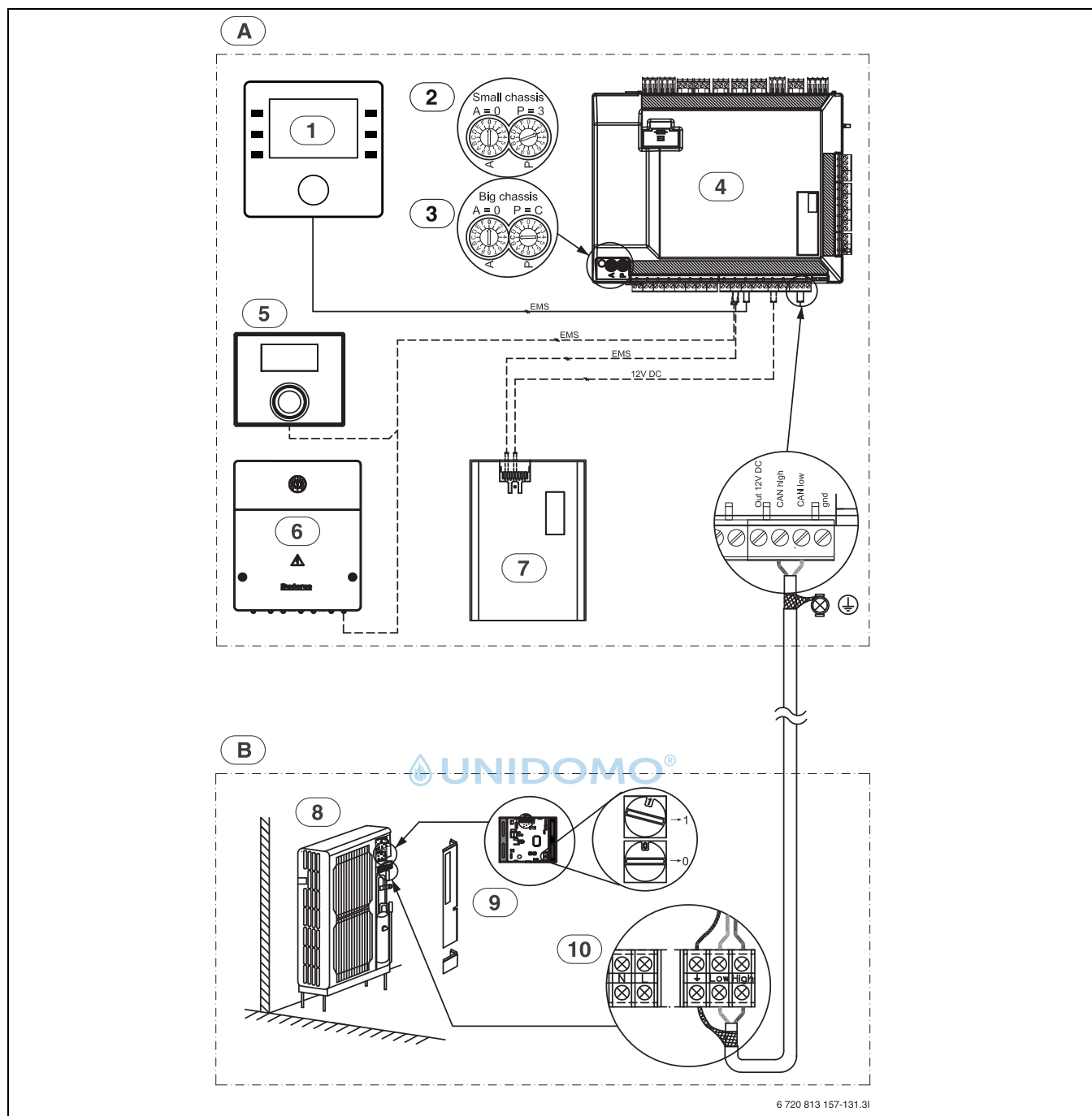
Bild 33 Übersicht der Inneneinheit mit externem Zuheizer
