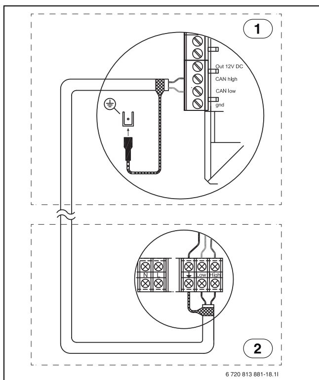
Bild 9 CAN-BUS-Verbindung
