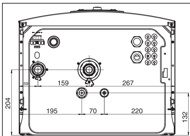
Bild 4 Abmessungen und Anschlüsse
