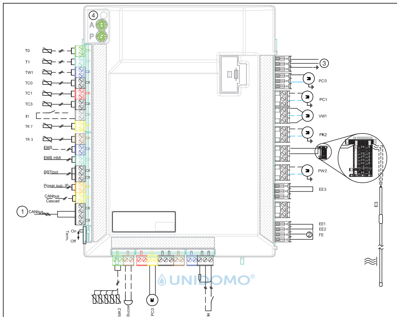
Bild 12 Installationsmodul SEC 20 Inneneinheit mit Elektroheizung
