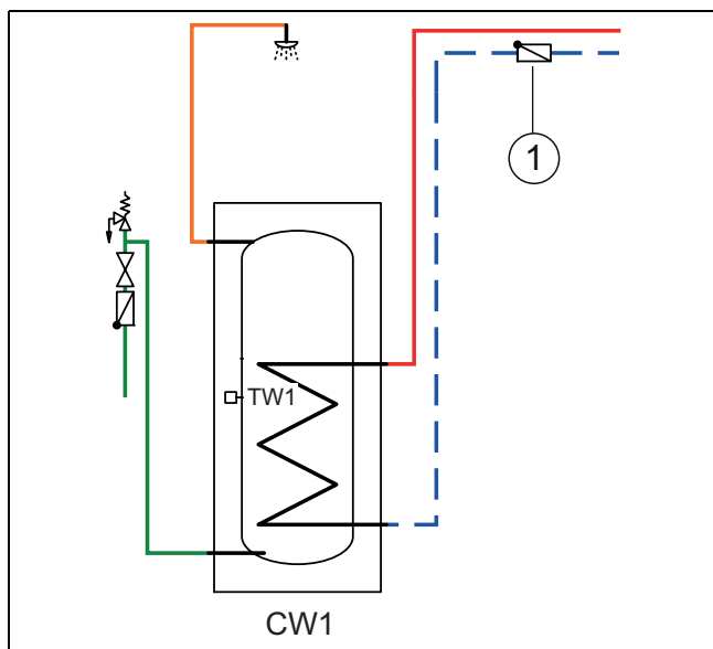
Bild 17 Warmwasserspeicher
