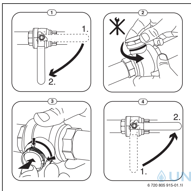
Bild 15 Siebreinigung
