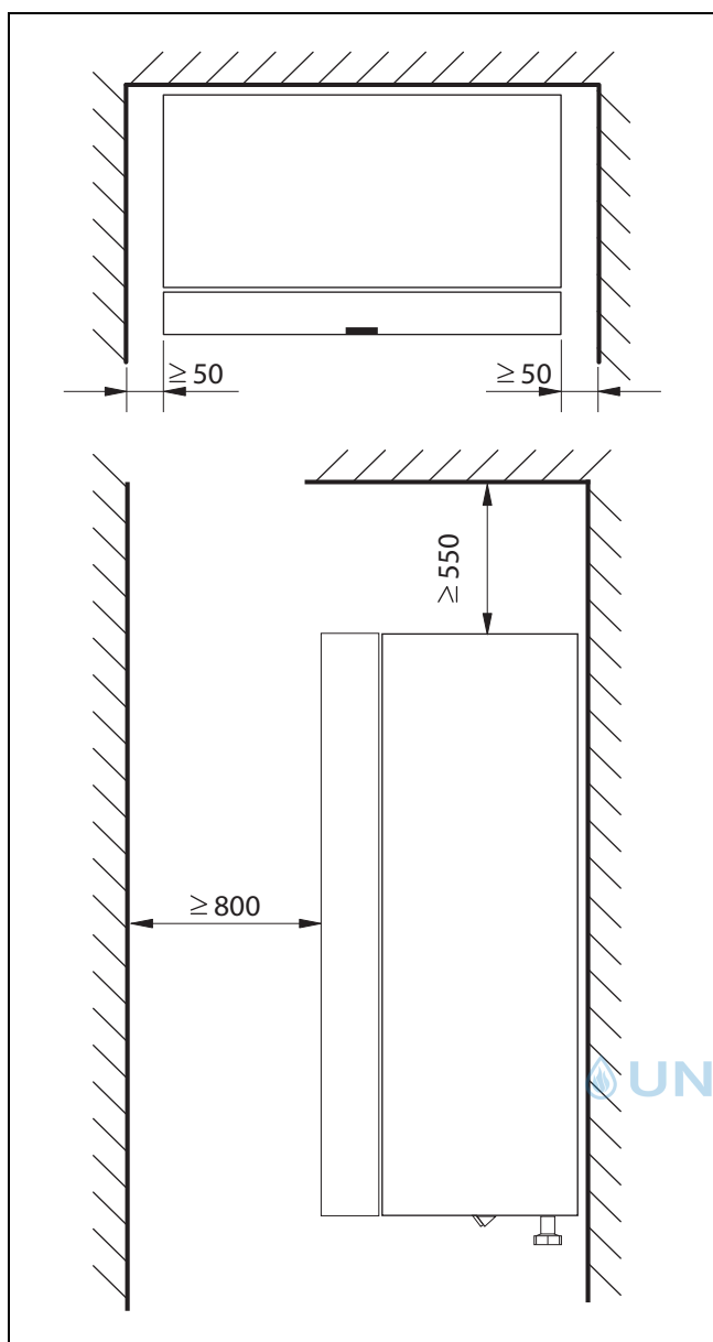
Bild 3 Mindestabstand (mm)
