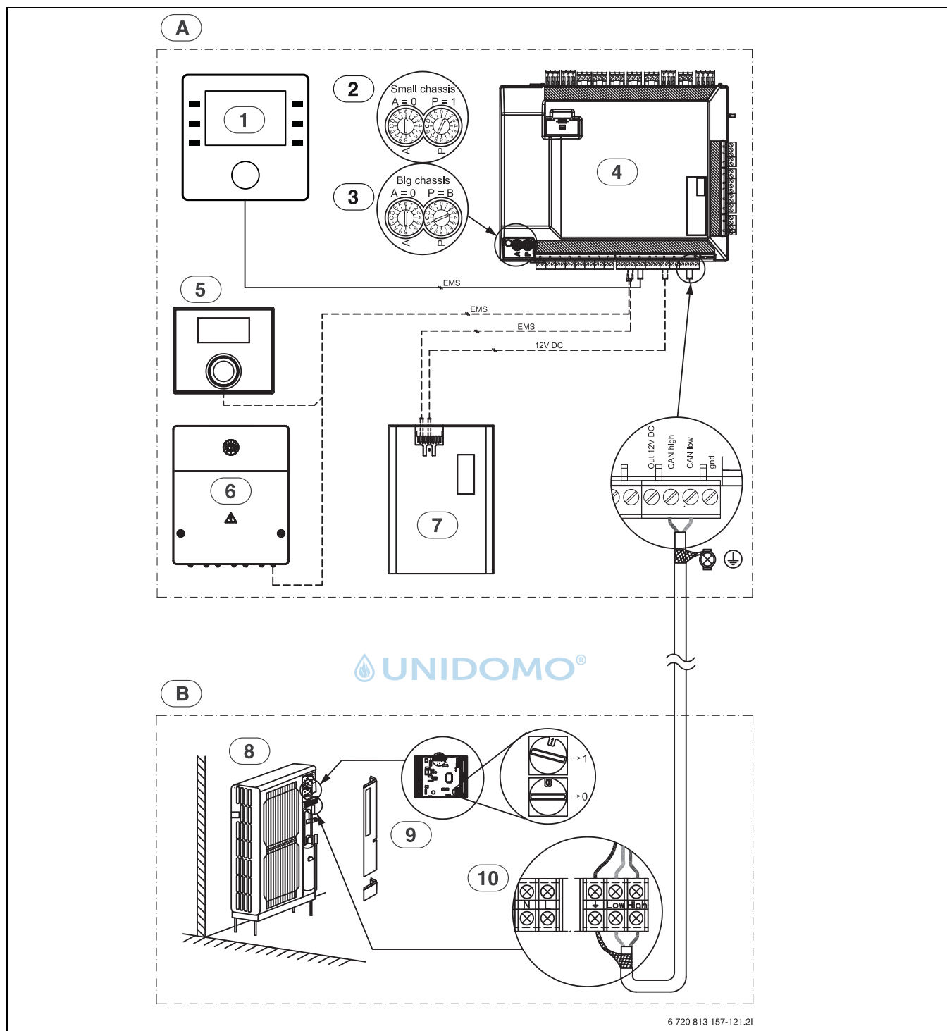
Bild 30 CAN und EMS Anschlüsse
