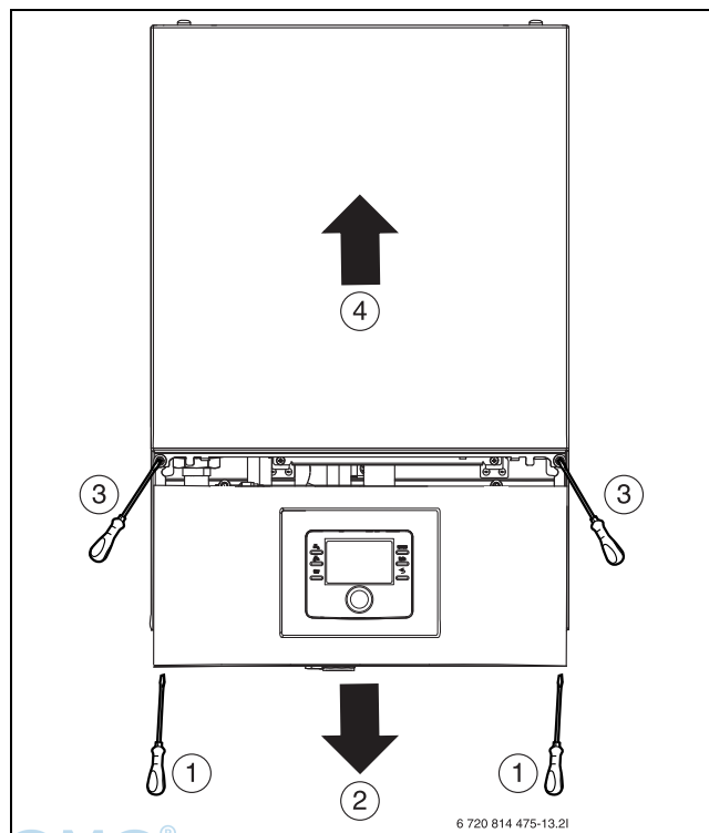
Bild 5 Frontverkleidung abnehmen
