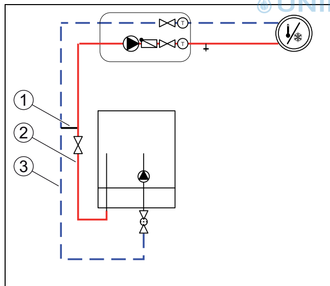
Bild 24 Inneneinheit mit Heizkreis und Bypass
