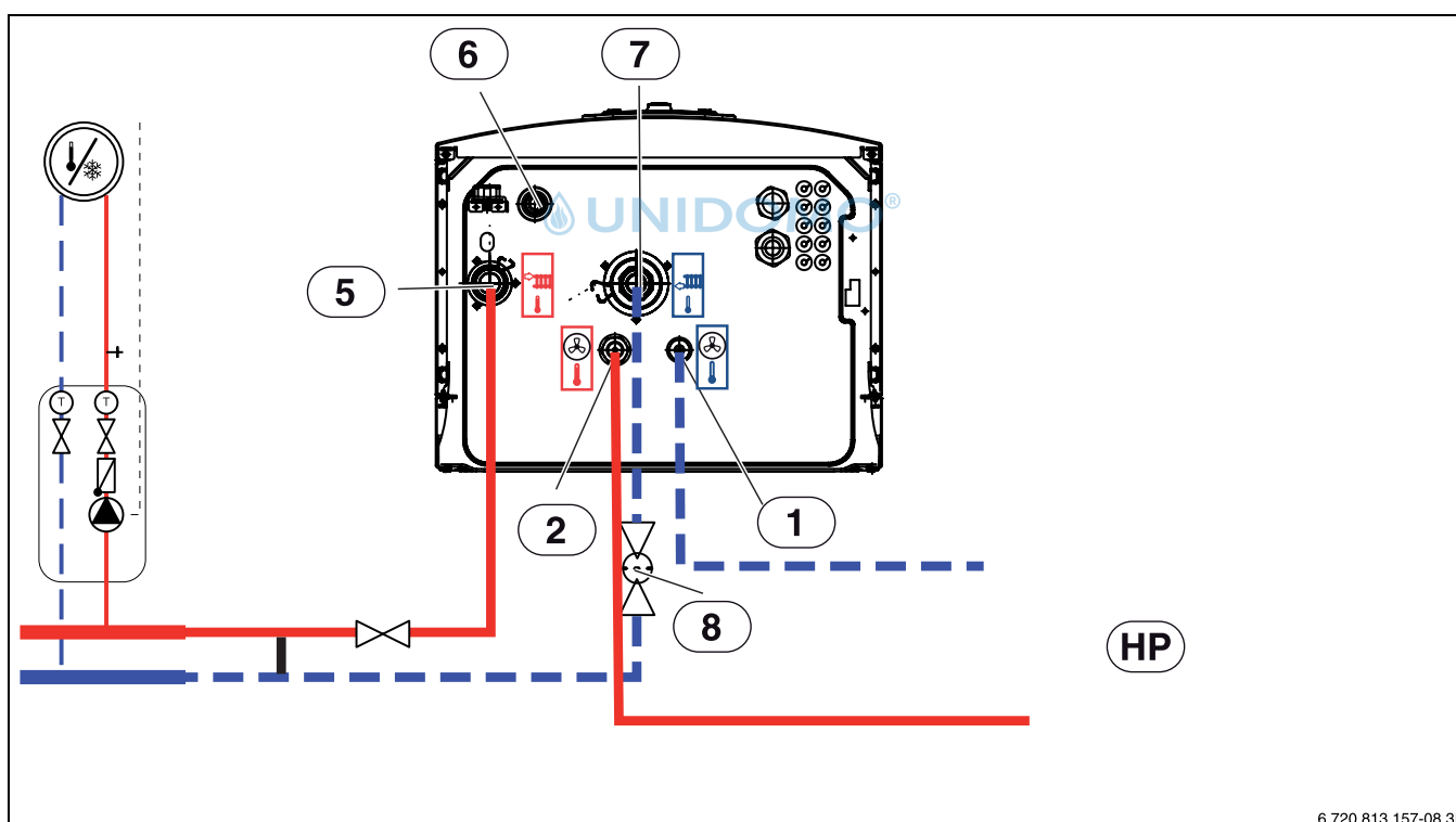
Bild 7 Anschluss einer Inneneinheit mit Elektro-Heizeinsatz an eine Wärmepumpe und ein Heizsystem
