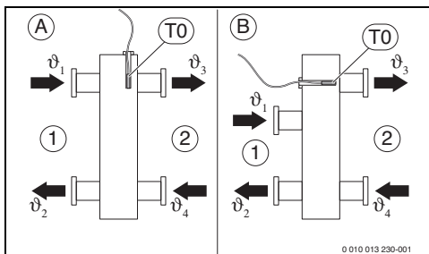
Fig. 3 Posición de la sonda de temperatura de impulsión (T0)
