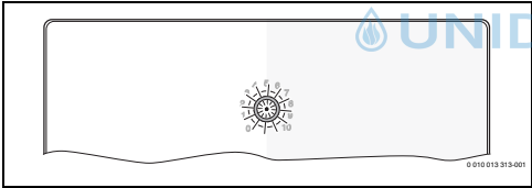
Fig. 5 Interruptor codificador con visualización de estado del módulo y visualización de estado de los módulos o generadores de calor conectados
