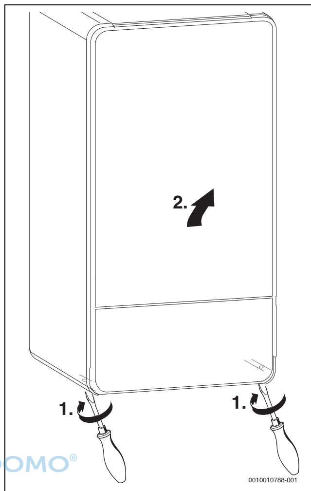
Bild 30 Verkleidung abnehmen
