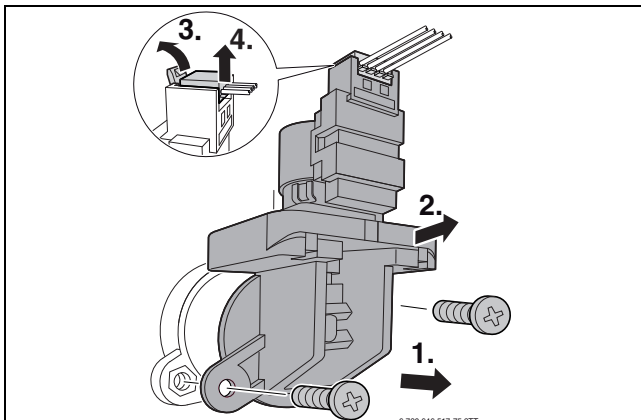
Bild 72 3-Wege-Ventil ausbauen
