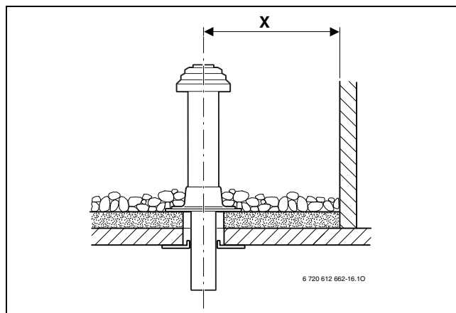
Bild 7 Abstandsmasse bei Flachdach
