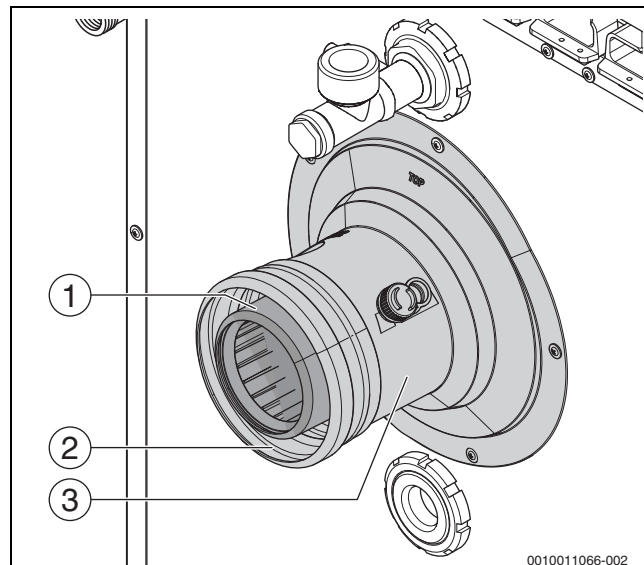
Bild 15 Abgasanschluss montieren
