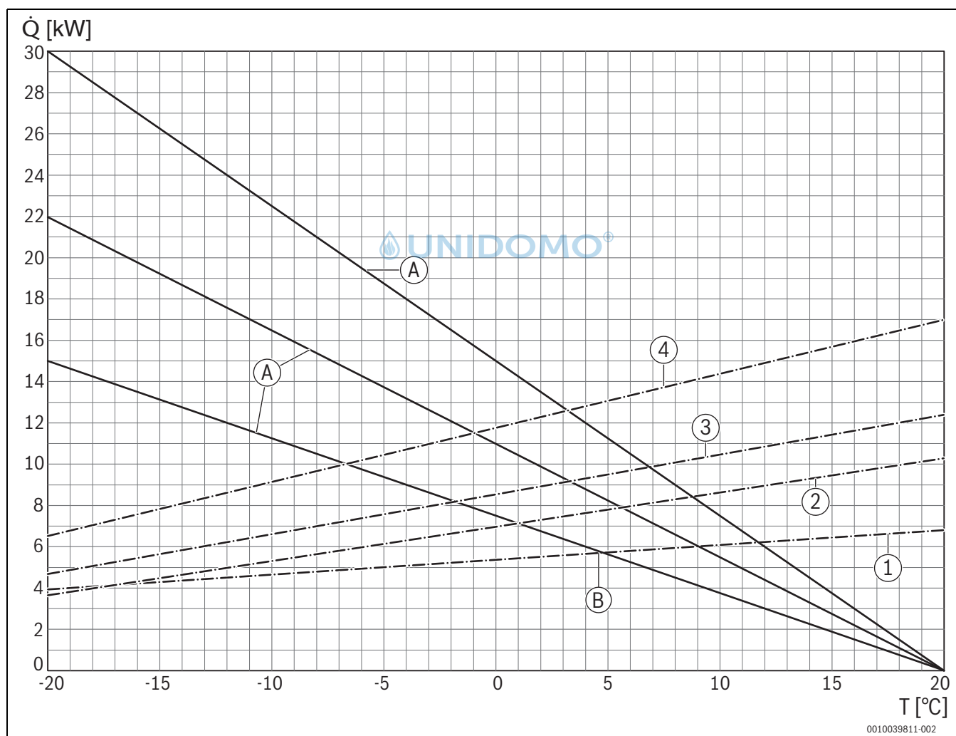
Bild 27 Diagramm zu Tab. 5; Zur Bestimmung der Bivalenzpunkte bei 55 °C Vorlauftemperatur
