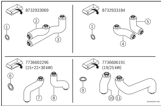
Bild 3 Optionale Rohrgruppen
