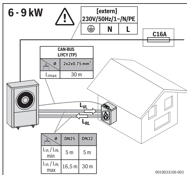
Bild 8 Maximale Längen der Leitungen 6 – 9 kW
