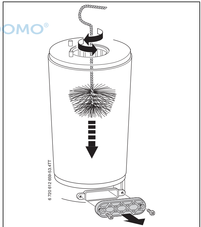
Bild 57 Wärmeblock reinigen
