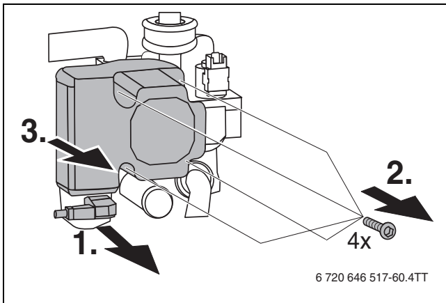
Bild 68 Heizungspumpe ausbauen
