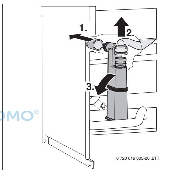
Bild 60 Kondensatsiphon ausbauen
