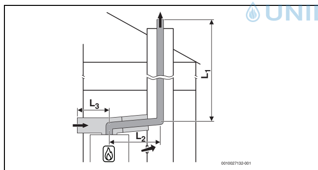
Bild 12 Starre Abgasführung nach C 53x im Schacht und Luft-Abgas-Führung mit separater Luftzufuhr und konzentrischer Abgasableitung im Aufstellraum
