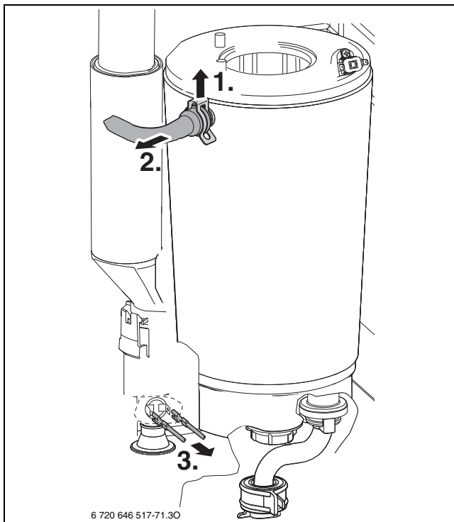
Bild 73 Vorlaufrohr lösen und Kabel abziehen
