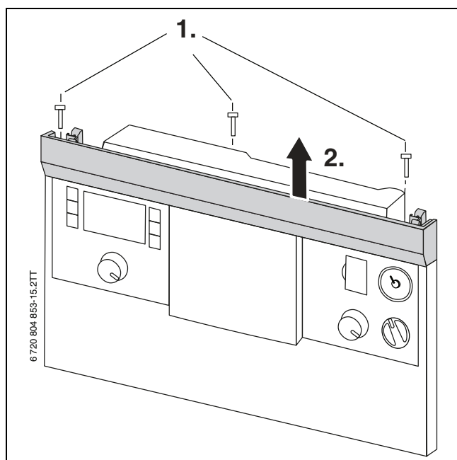
Bild 36 Abdeckung entfernen
