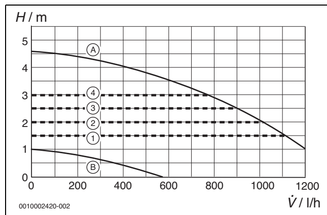
Bild 79 Pumpenkennfelder und Pumpenkennlinien
