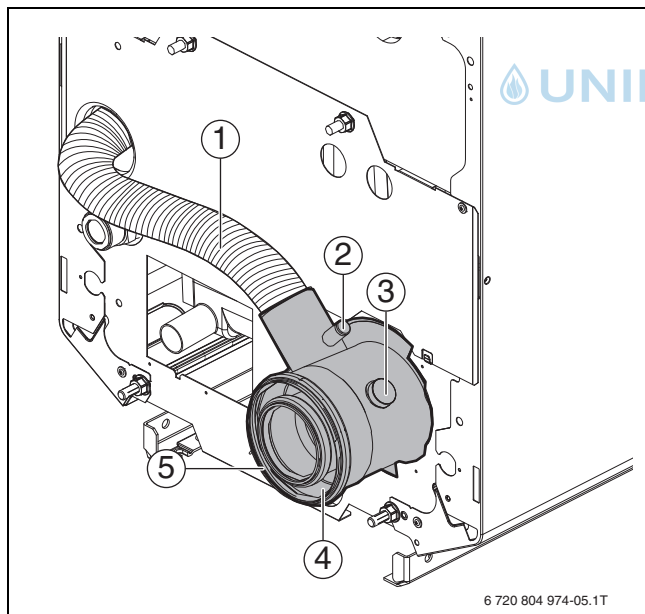
Bild 15 Luft-Abgas-Anschlussstutzen montieren
