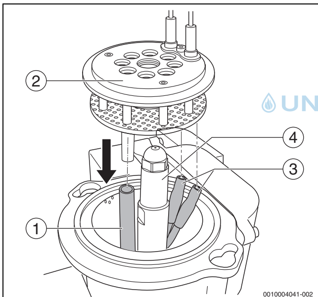
Bild 37 Mischsystem montieren
