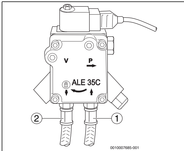
Bild 18 Ölpumpe – Suntec
