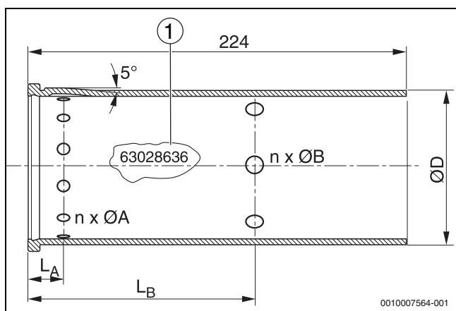
Bild 5 Brennerrohre
