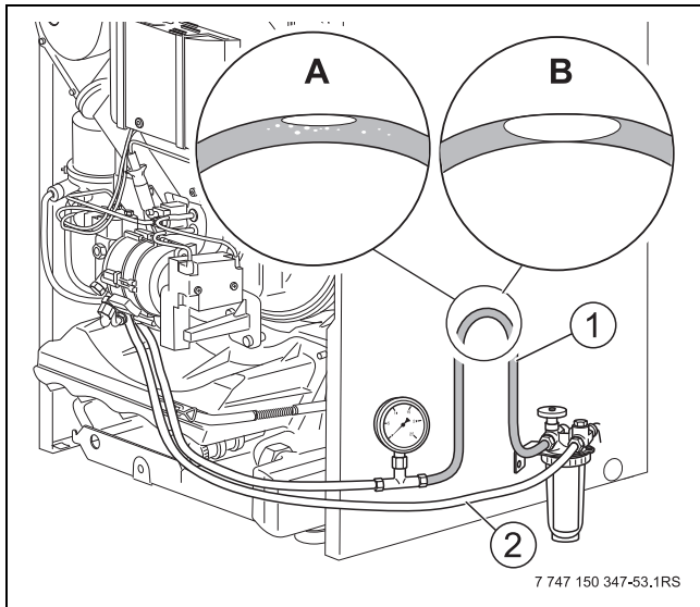
Bild 16 Transparenten Schlauch hochbinden
