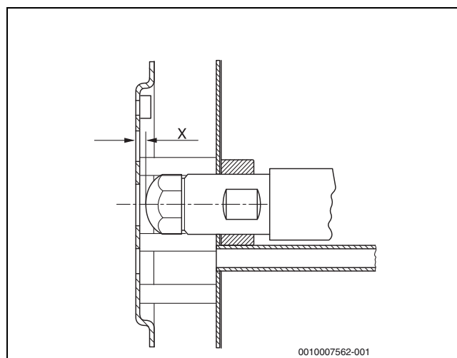
Bild 4 Mischsystem – Maß „X“
