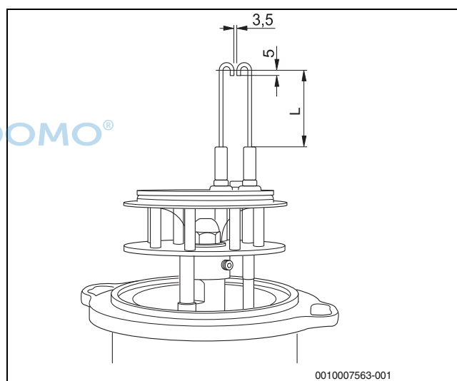
Bild 3 Zündeletrode (Maße in mm)
