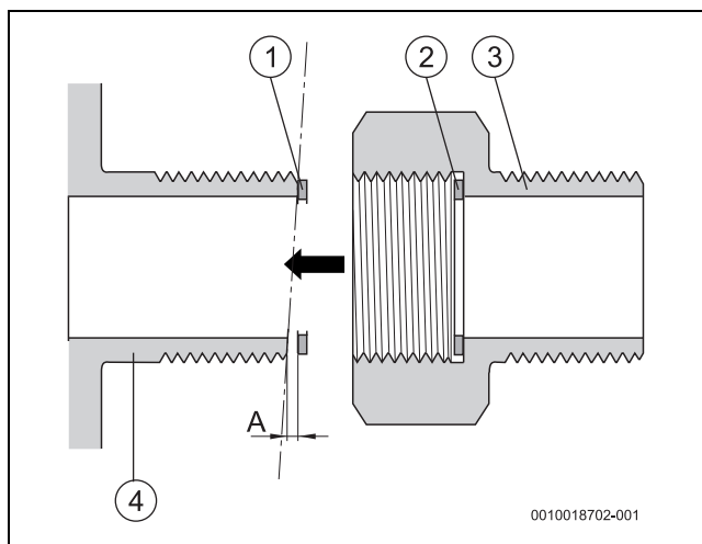
Bild 2 Messingadapter montieren
