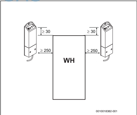
Bild 1 Empfohlener Installationsort bei wandhängenden Heizgeräten
