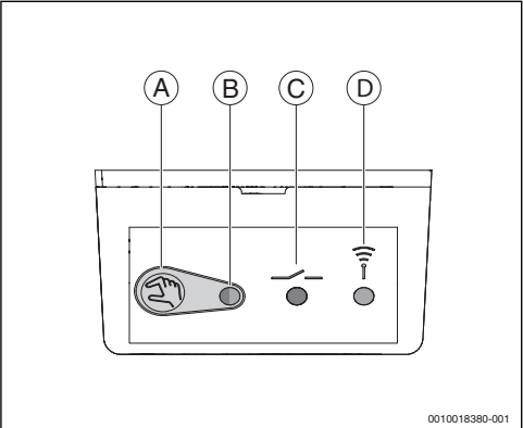
Bild 6 Bedien- und Anzeigeelemente
