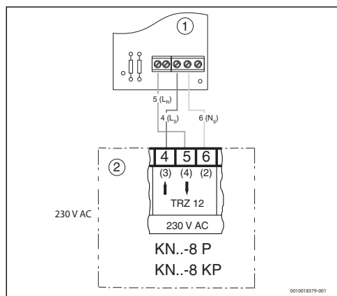
Fig. 11 Schéma de connexion de la chaudière Supramodul ou Supranorm
