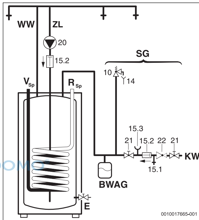
Bild 1 Trinkwasserseitiges Anschluss-Schema
