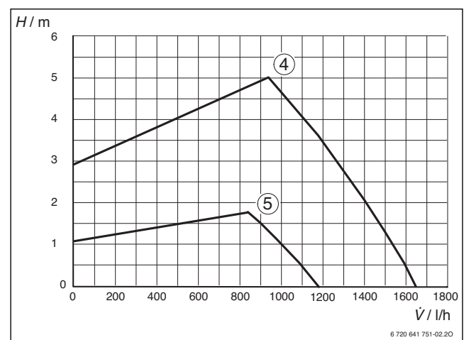
Bild 43 Proportionaldruck
