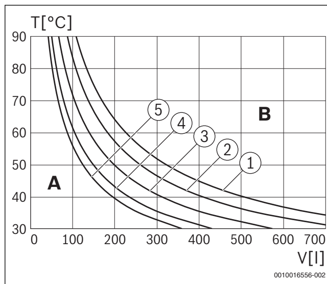
Bild 8 ZWR/ZSR 18/24...-7 KE
