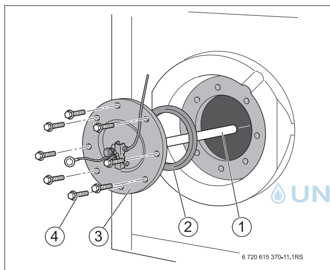
Bild 13 Prüföffnung öffnen
