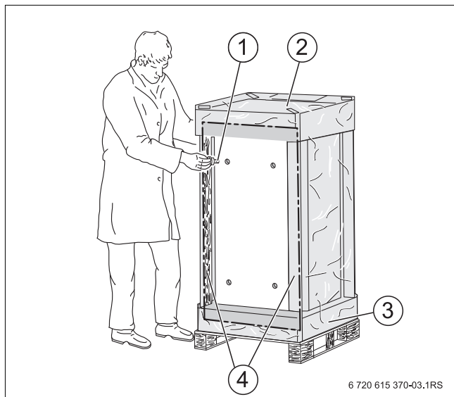
Sl.3 Razrežite pakirnu foliju i uvijte podne oslonce
