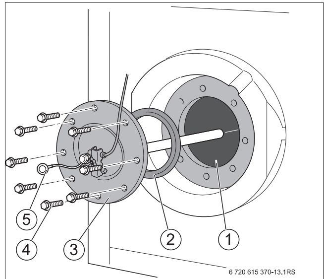
Afb. 16 Inspectieopening sluiten
