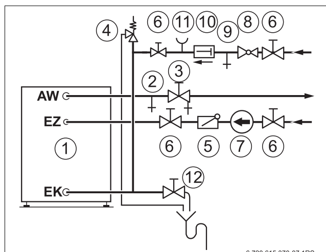
Fig. 7 Installation (schéma de principe)
