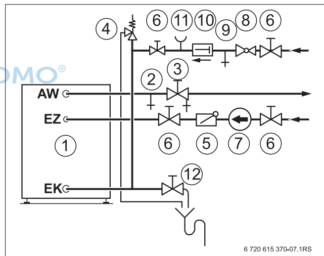
Afb. 7 Installatie (principeafbeelding)
