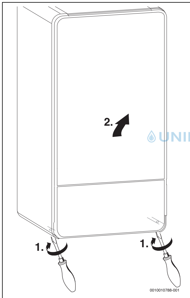
Bild 29 Verkleidung abnehmen
