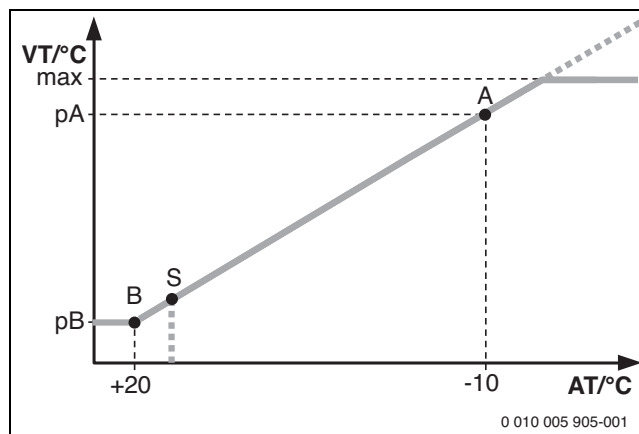
Bild 85 Heizkurve
