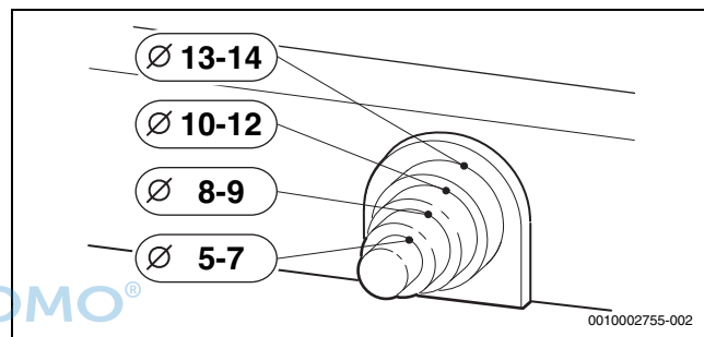
Bild 36 Zugentlastung an Kabeldurchmesser anpassen
