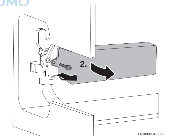
Bild 67 Plattenwärmetauscher ausbauen
