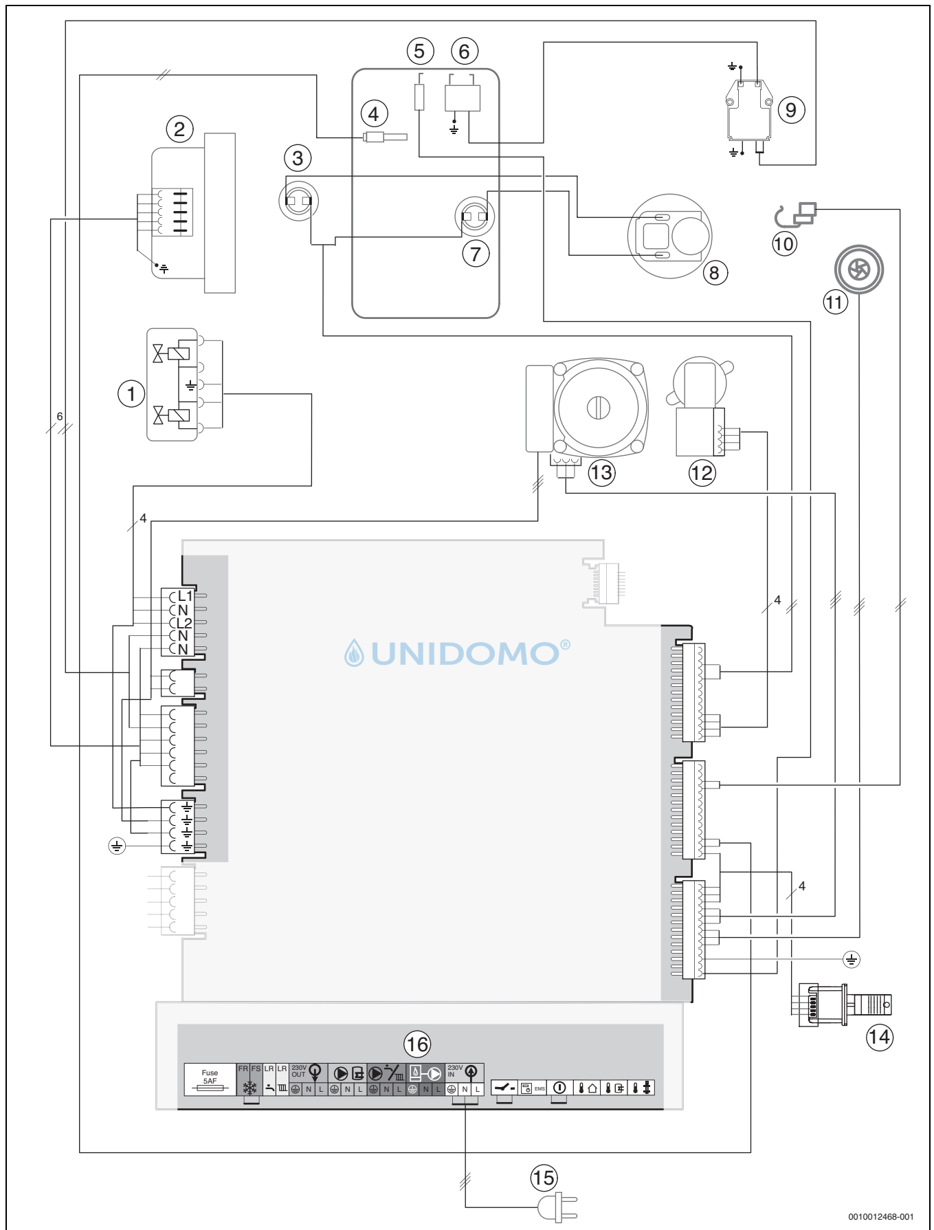
Bild 84 Elektrische Verdrahtung
