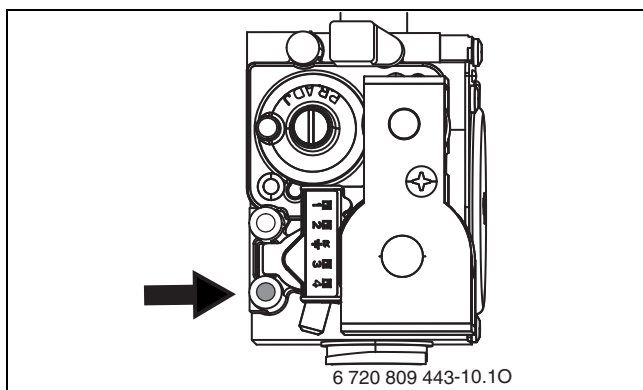
Bild 53 Messstutzen für Gas-Anschlussdruck
