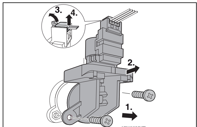
Bild 72 3-Wege-Ventil ausbauen
