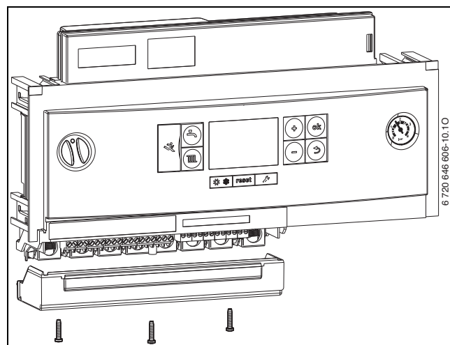
Bild 35 Abdeckung entfernen
