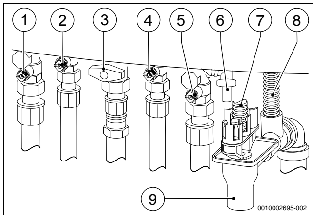
Bild 33 Gas- und wasserseitige Anschlüsse (Zubehör)
