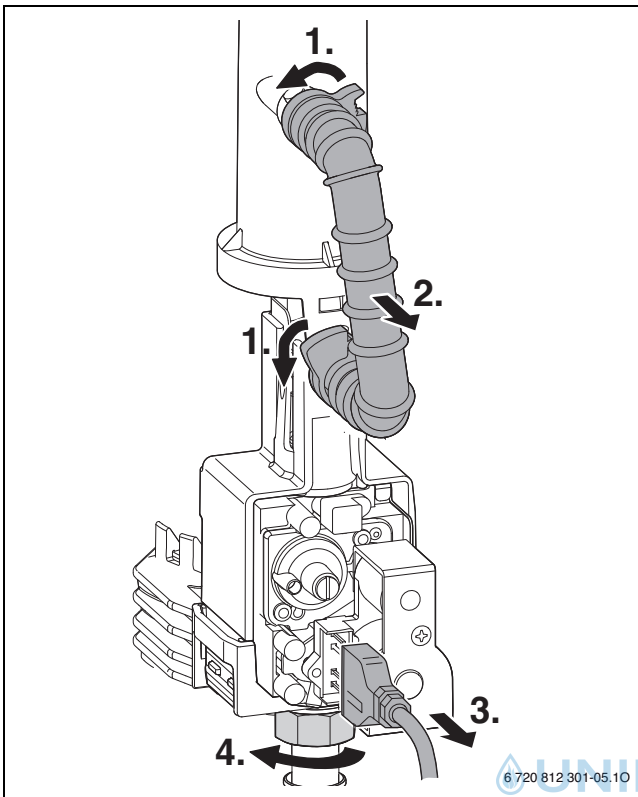
Bild 77 Gasarmatur ausbauen
