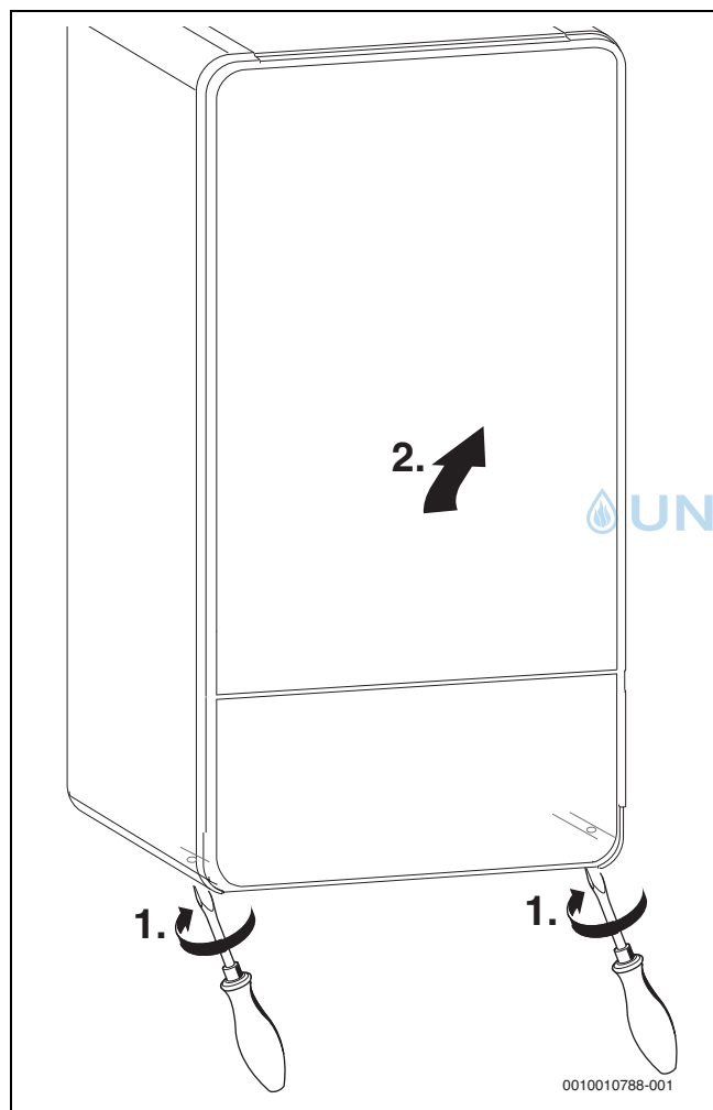
Bild 30 Verkleidung abnehmen
