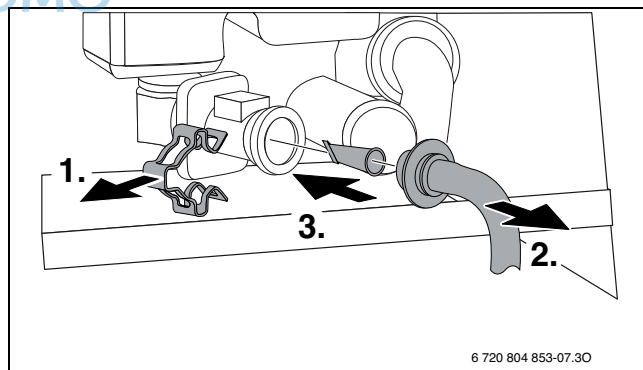
Bild 71 Sieb aus Kaltwasserrohr ausbauen
