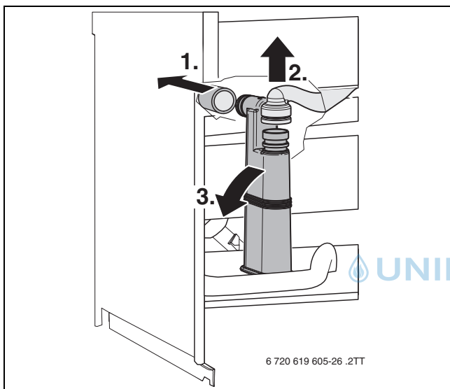
Bild 68 Kondensatsiphon ausbauen
