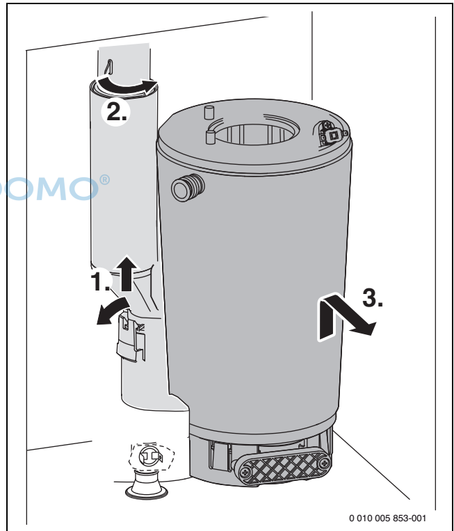
Bild 85 Wärmeblock ausbauen
