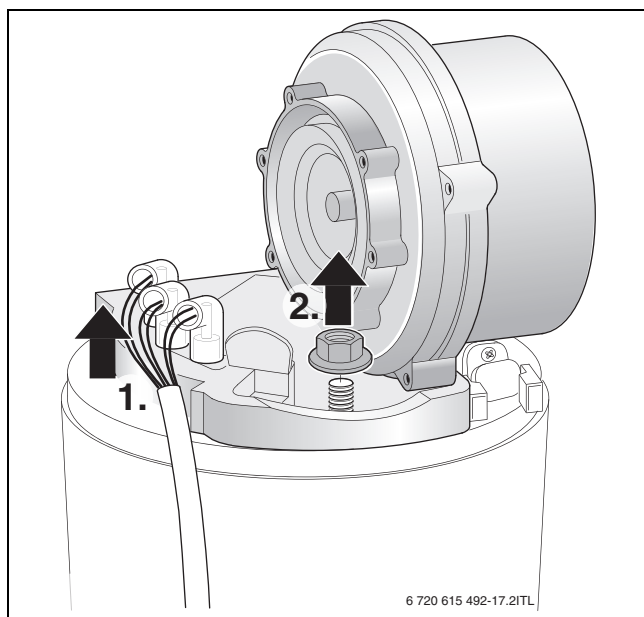
Bild 61 Gebläse herausnehmen
