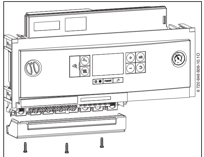
Bild 79 Abdeckung entfernen
