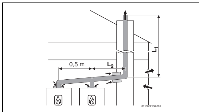
Bild 26 Kaskade mit 2 Geräten: Starre Abgasführung im Schacht nach B 23p /B 53p mit raumluftabhängiger Luftzufuhr am Gerät
