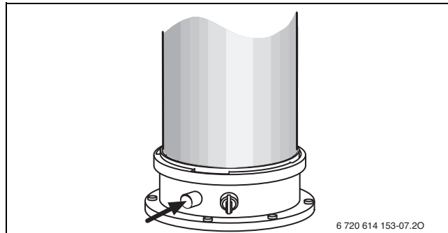
Bild 53 Abgasmessstutzen
