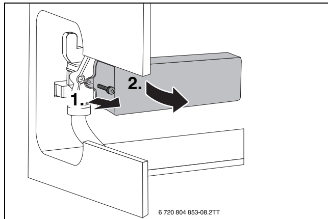
Bild 70 Plattenwärmetauscher ausbauen
