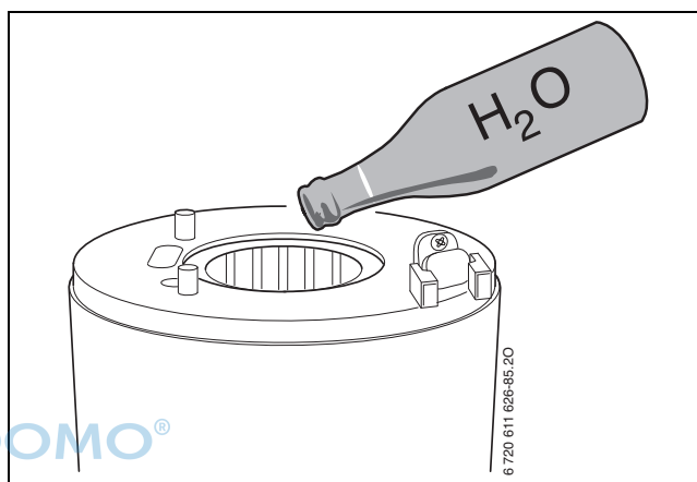
Bild 67 Wärmeblock mit Wasser spülen
