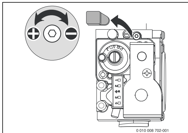
Bild 54 Plombe entfernen
