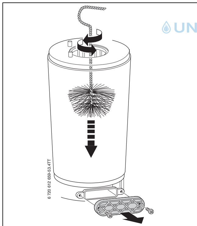
Bild 65 Wärmeblock reinigen
