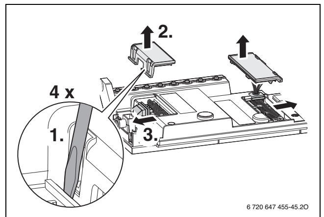
Bild 81 Abdeckung entfernen
