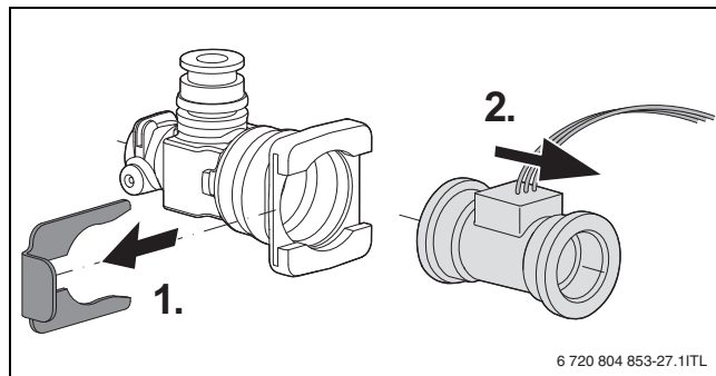
Bild 72 Turbine am Kaltwasserrohr ausbauen
