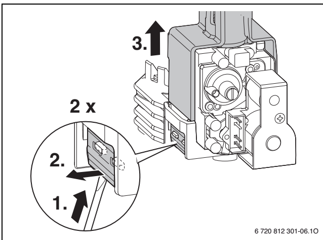
Bild 78 Gasarmatur ausbauen
