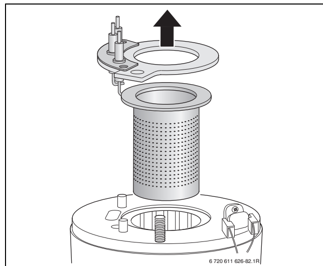
Bild 62 Brenner herausnehmen
