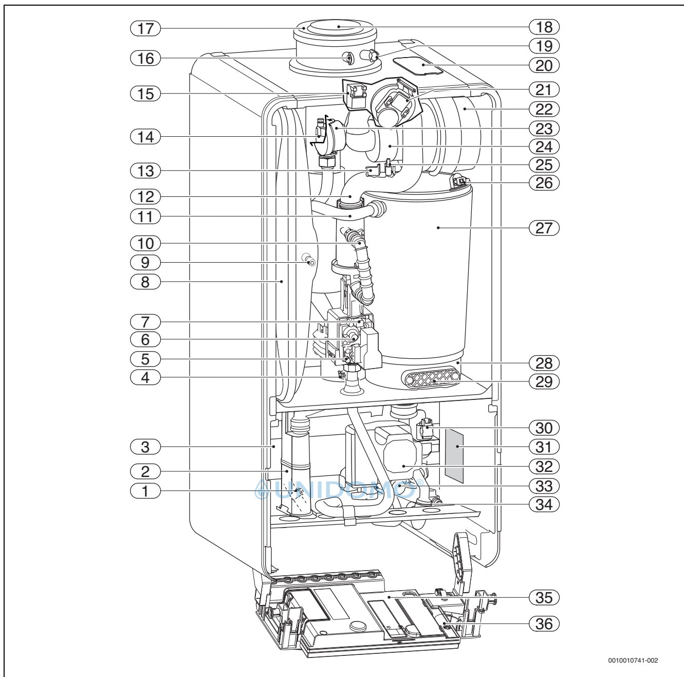
Bild 3 Produktübersicht
