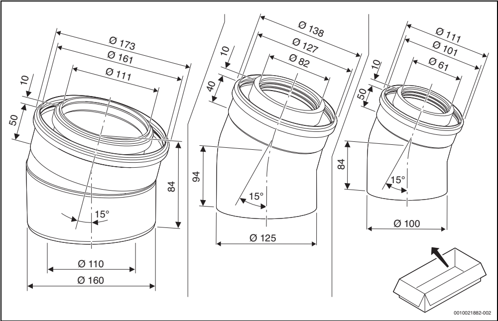
1 \varnothing 110/160 : 7738113102, \varnothing 80/125 : 7738112594, \varnothing 60/100 : 7738112529
