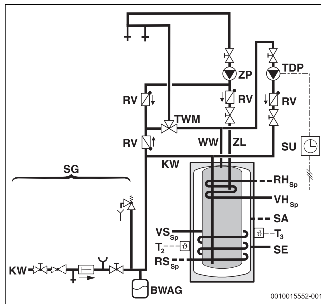
Afb. 2 Aansluitschema drinkwaterzijde
