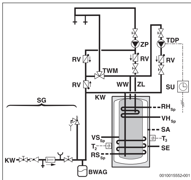
Rys. 2 Schemat podłączenia przewodów wody użytkowej
