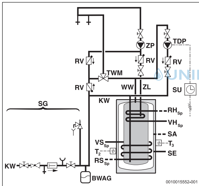
Obr. 2 Schéma pripojenia na strane pitnej vody
