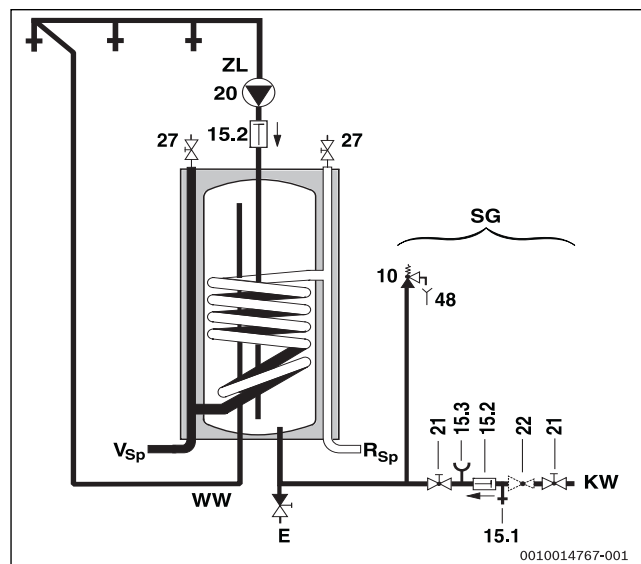
Fig. 4 Schéma de raccordement côté eau chaude sanitaire
