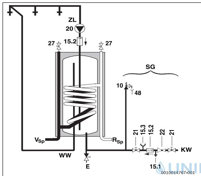
Bild 1 Trinkwasserseitiges Anschluss-Schema
