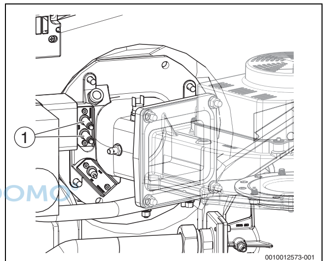
Bild 37 Zündelektroden
