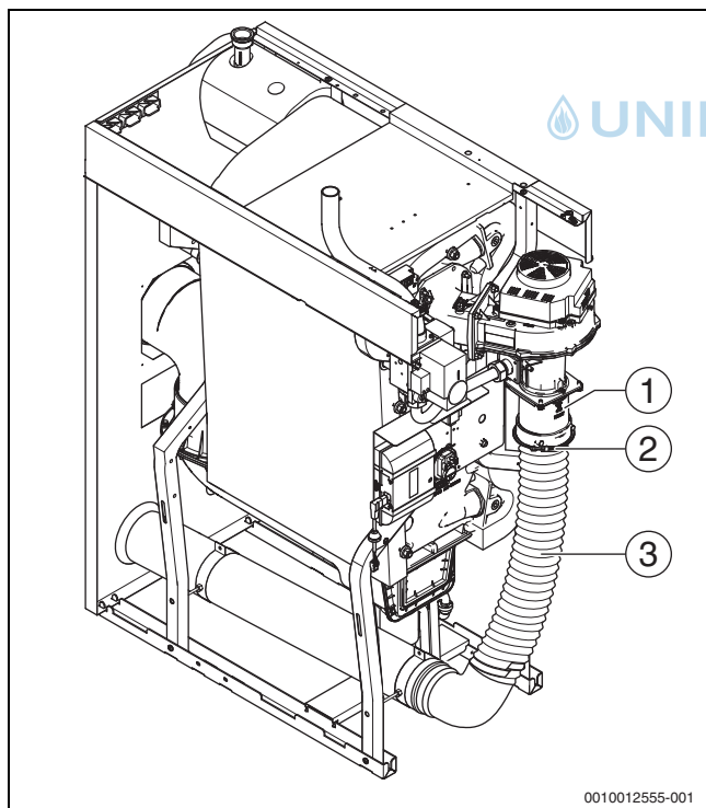
Bild 40 Zuluftleitung
