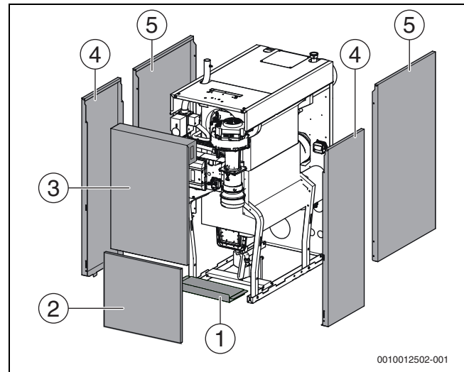
Bild 30 Verkleidungsteile montieren
