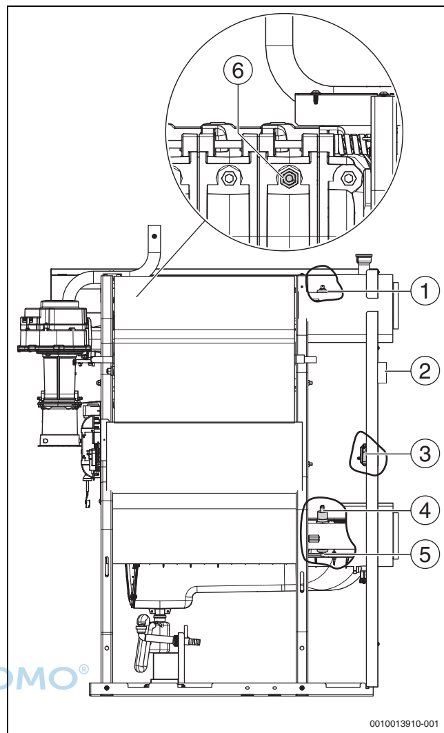
Bild 33 Detail-Übersicht: Position der Fühler
