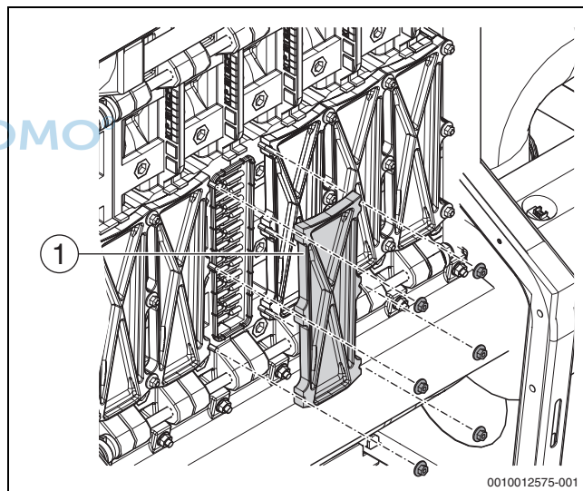
Bild 50 Reinigungsdeckel abnehmen
