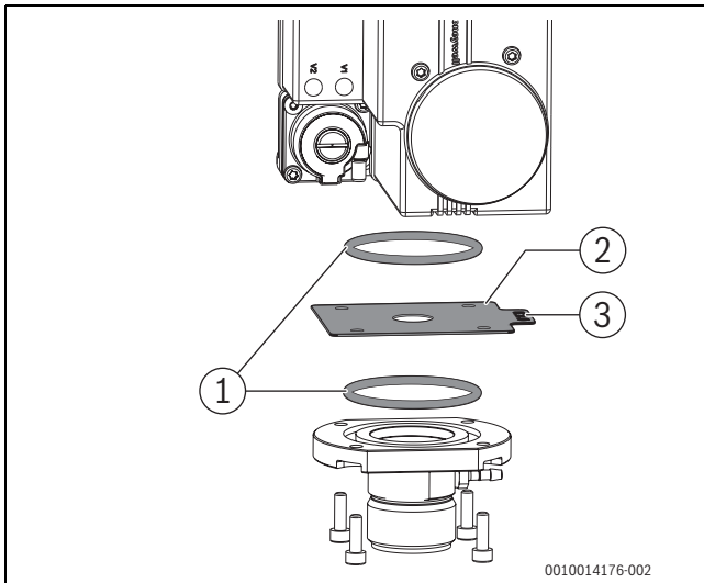
Bild 24 Gasblende austauschen
