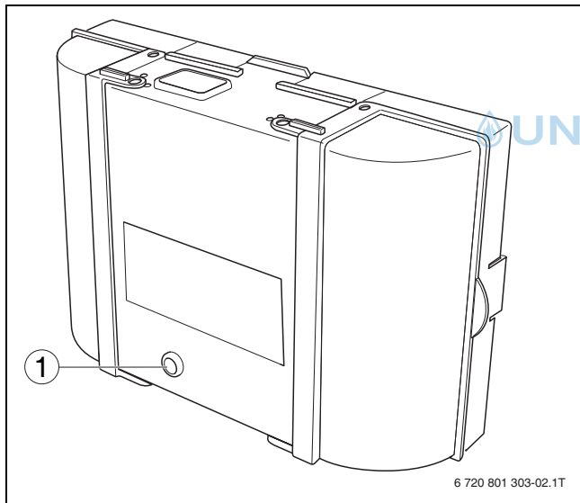
Bild 60 Störung am Feuerungsautomat zurücksetzen
