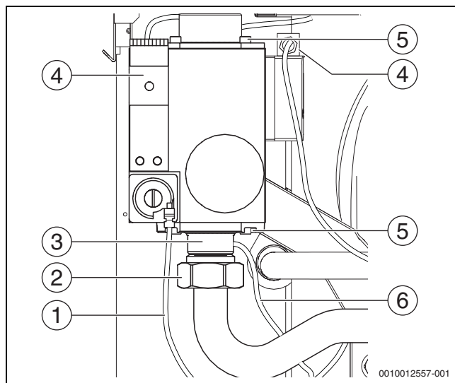
Bild 55 Anschlüsse Gasarmatur (150 ... 300 kW) lösen
