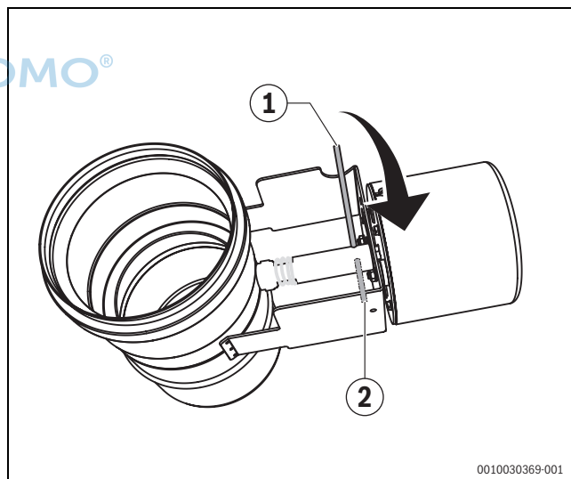
Bild 27 Stellstift an der Absperrklappe
