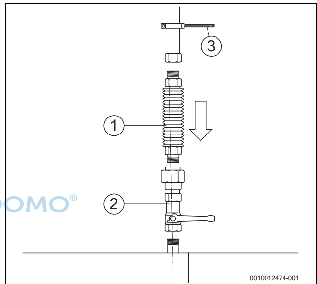
Bild 20 Gasanschluss herstellen
