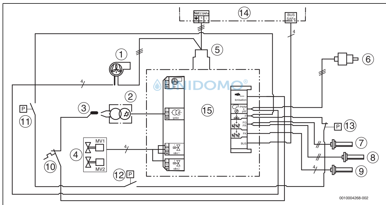
Bild 71 Anschlussplan Feuerungsautomat
