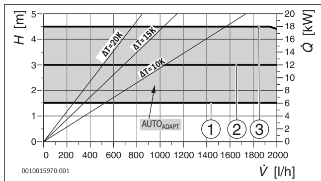
Bild 11 Pumpenkennlinien Konstantdruck
