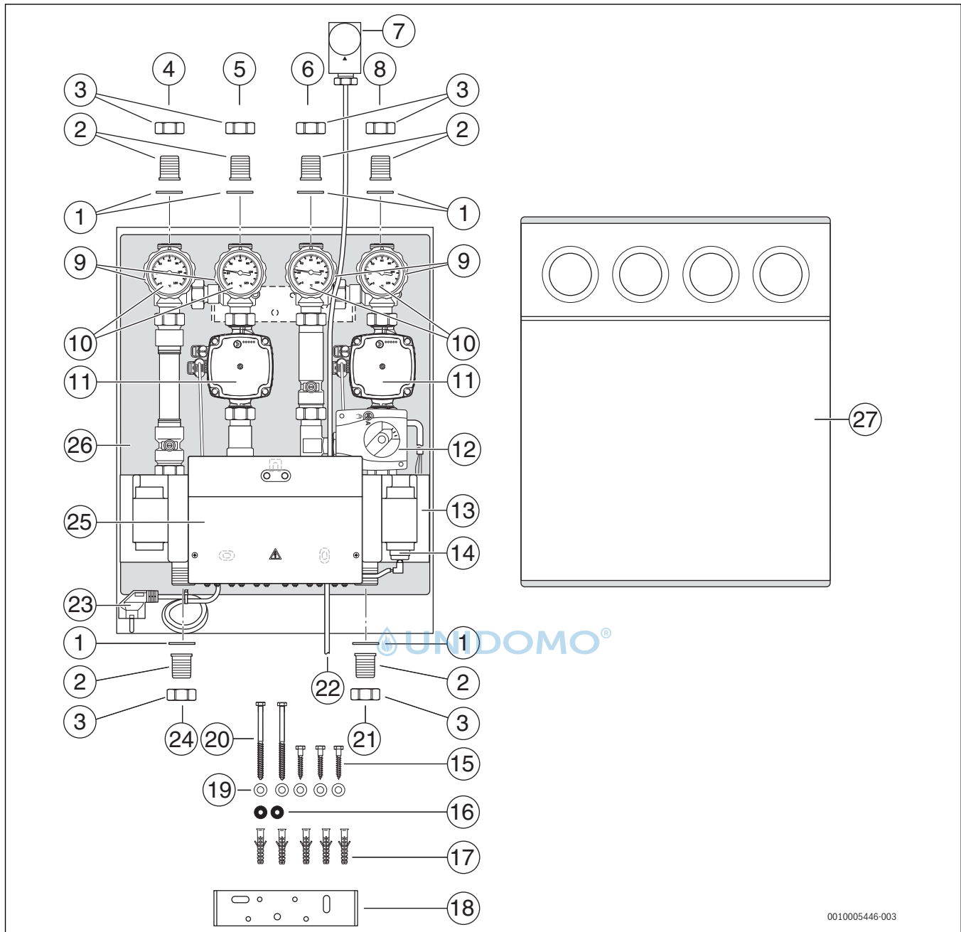
Bild 3 Lieferumfang MCM101
