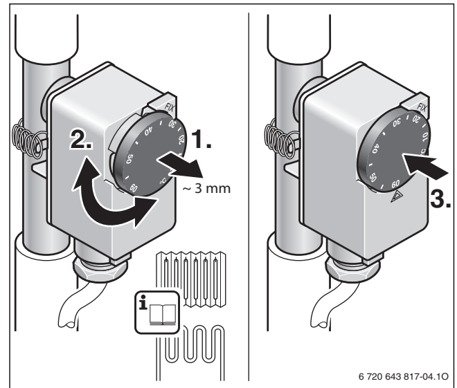
Bild 18 Temperatur einstellen
