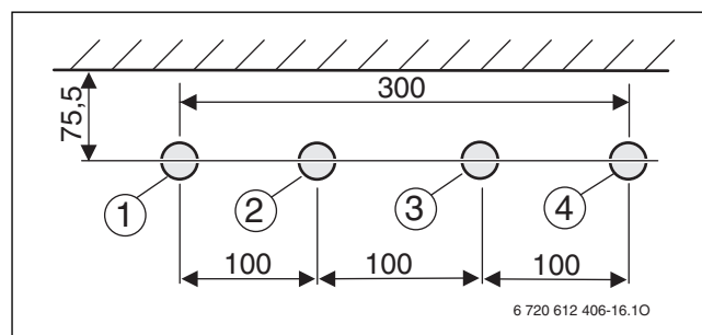
Bild 13 Maße für bauseitige Anschlussinstallation
