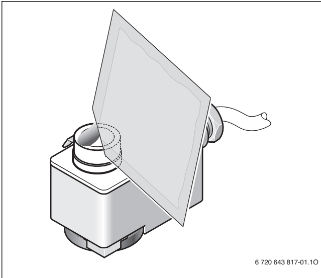
Bild 16 Wärmeleitpaste auftragen
