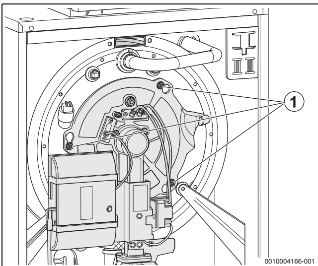
Bild 62 Befestigungsmuttern lösen
