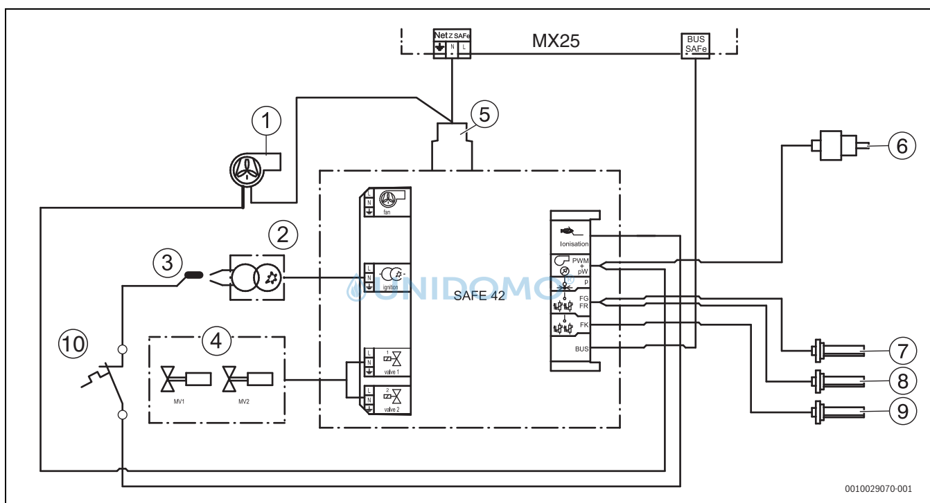
Bild 82 Anschlussplan Feuerungsautomat SAFe (50 kW; nicht bei allen Modellen)
