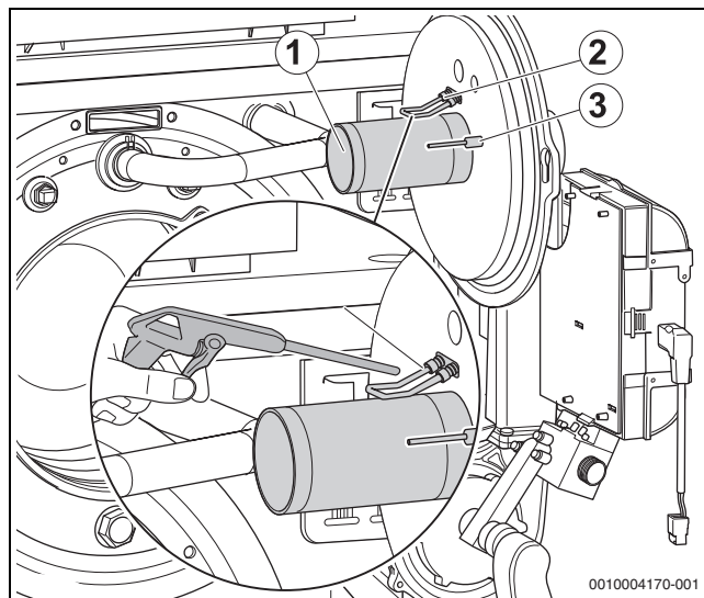
Bild 66 Brennerrohr mit Druckluft ausblasen
