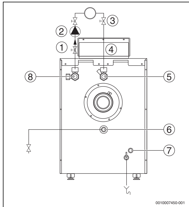
Bild 14 Anschlussschema Hydraulik
