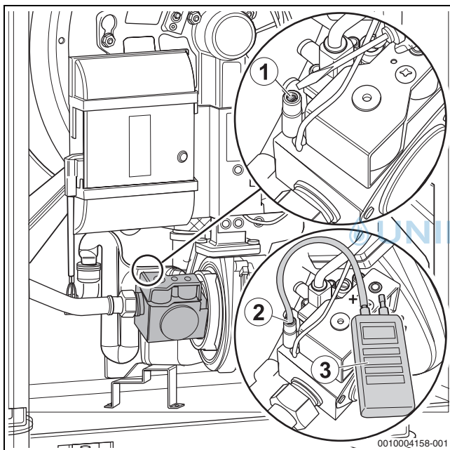
Bild 48 Gas-Anschlussdruck messen
