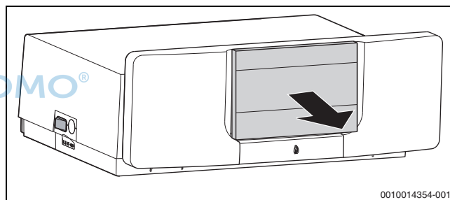
Bild 33 Abdeckung abziehen
