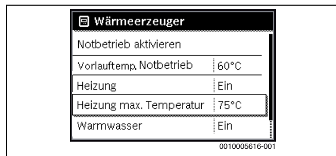
Bild 41 Maximale Vorlauftemperatur
