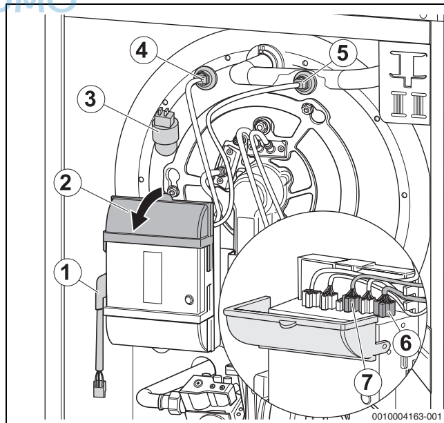
Bild 59 Steckverbinder lösen
