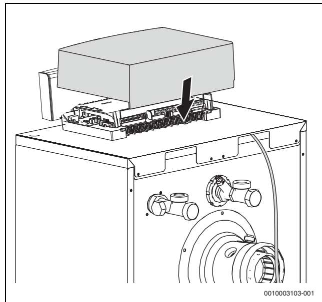
Bild 29 Abdeckhaube montieren
