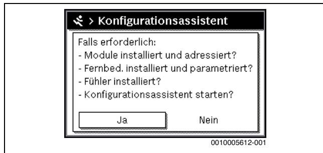
Bild 38 Konfigurationsassistent starten
