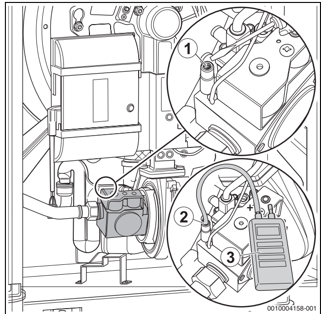
Bild 56 Gas-Anschlussdruck messen
