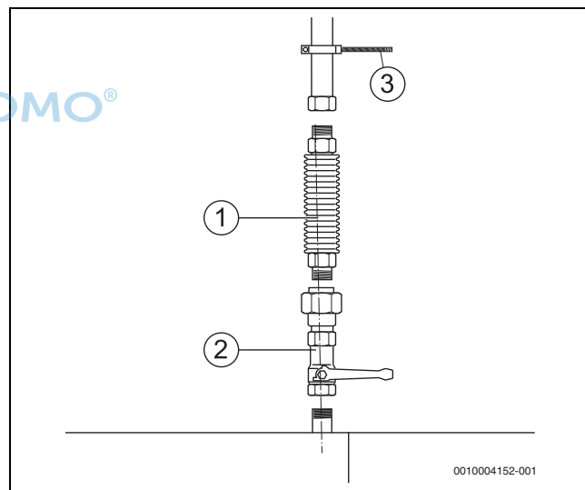
Bild 16 Gasanschluss herstellen
