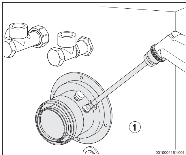
Bild 52 Messwerte aufnehmen
