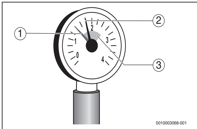
Bild 30 Manometer für geschlossene Anlagen
