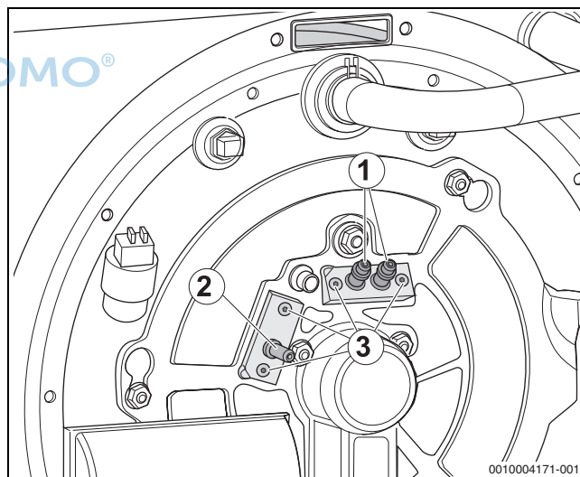
Bild 67 Elektrodenposition
