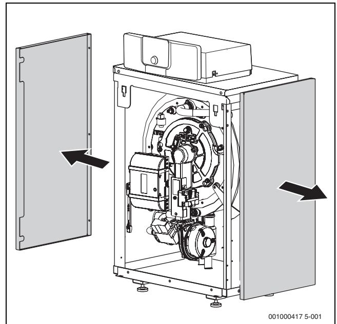
Bild 73 Seitenwände abnehmen
