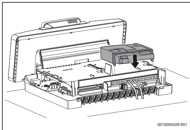
Bild 27 Funktionsmodule einstecken
