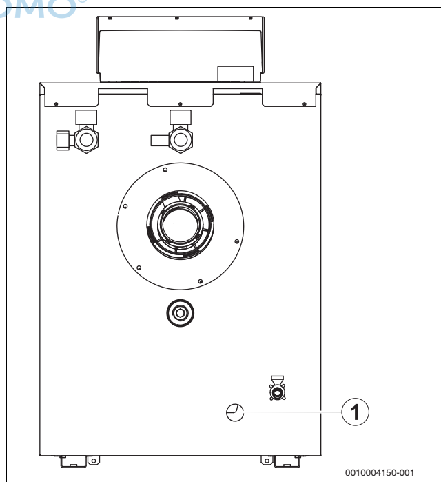
Bild 12 Kondensatschlauch montieren
